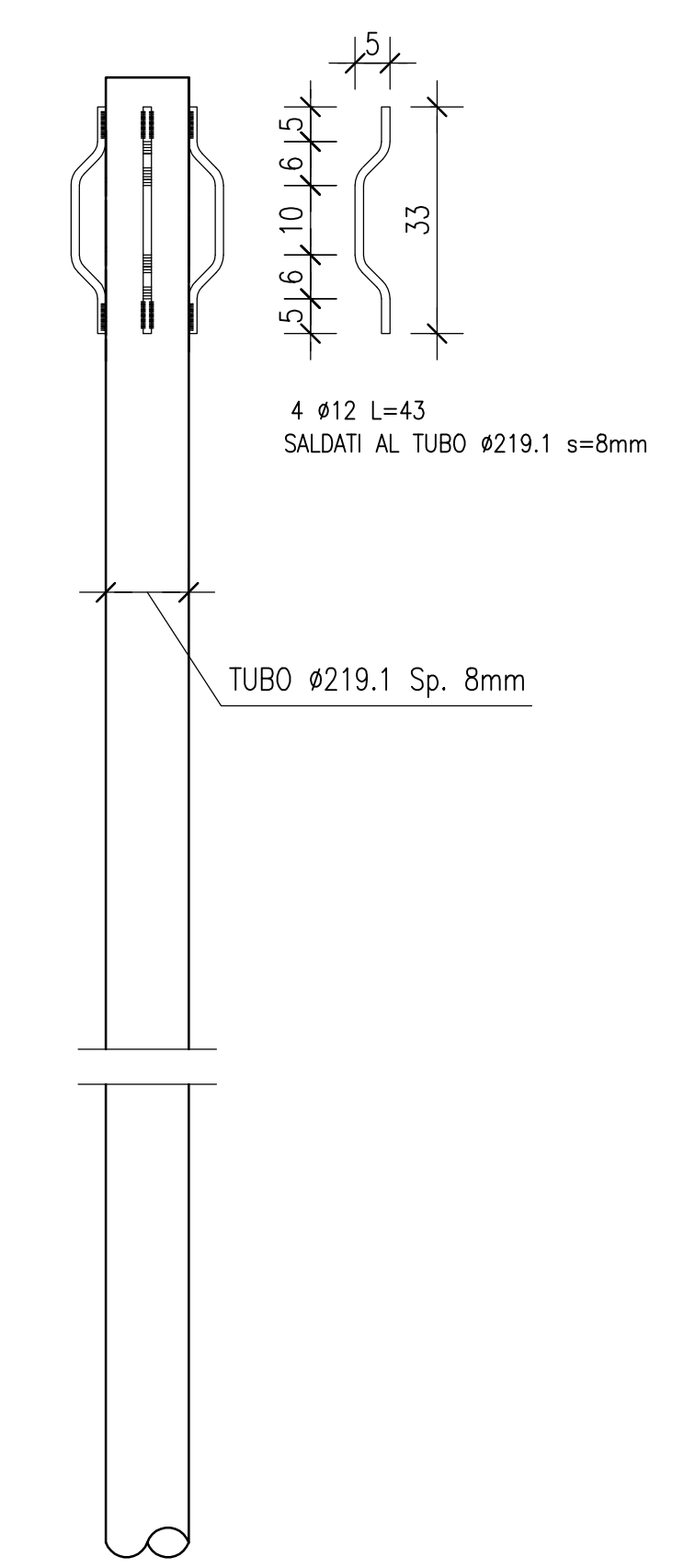
ARMATURA MICROPALO Scala 1:10
