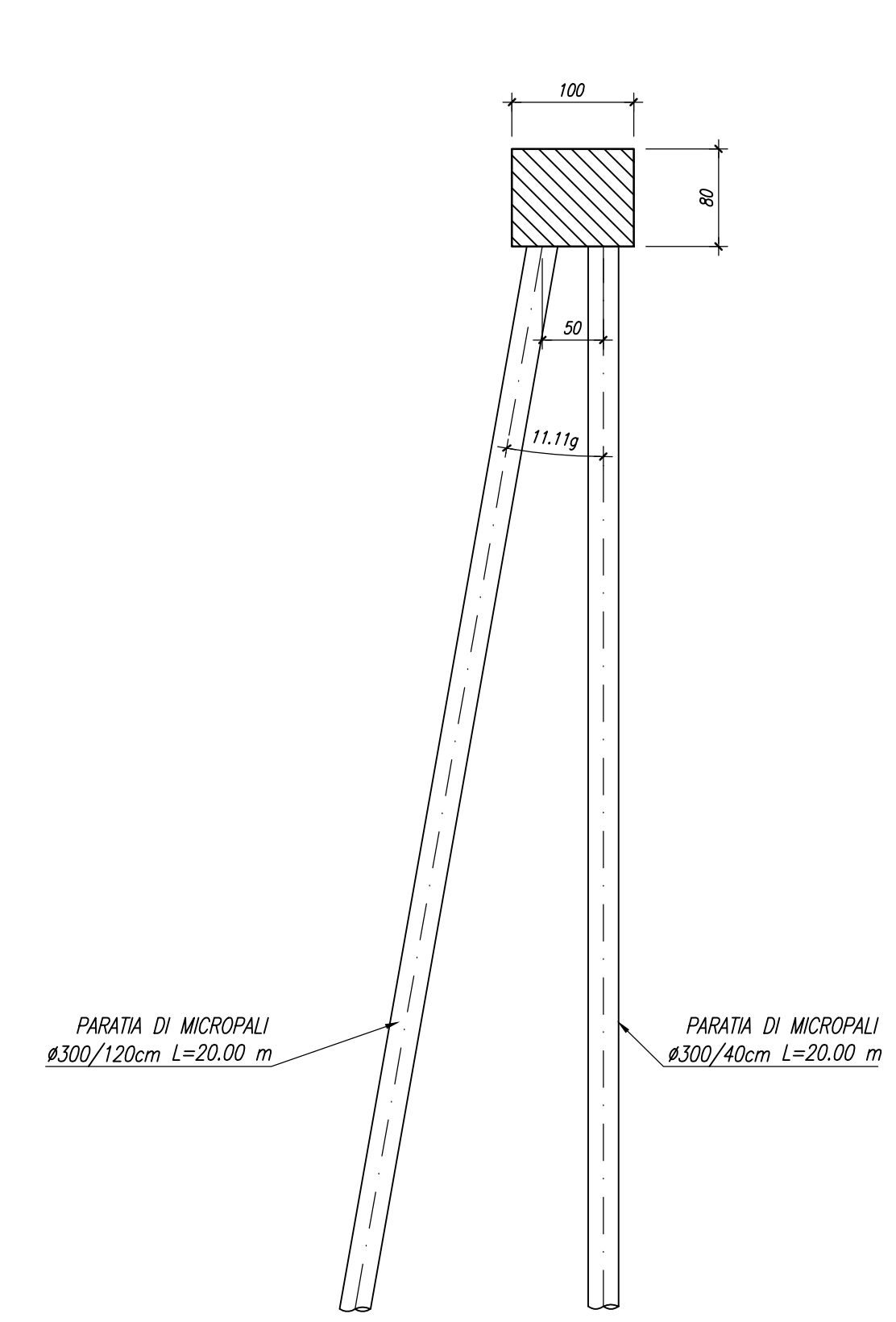
PARATIA MICROPALI Scala 1:50
