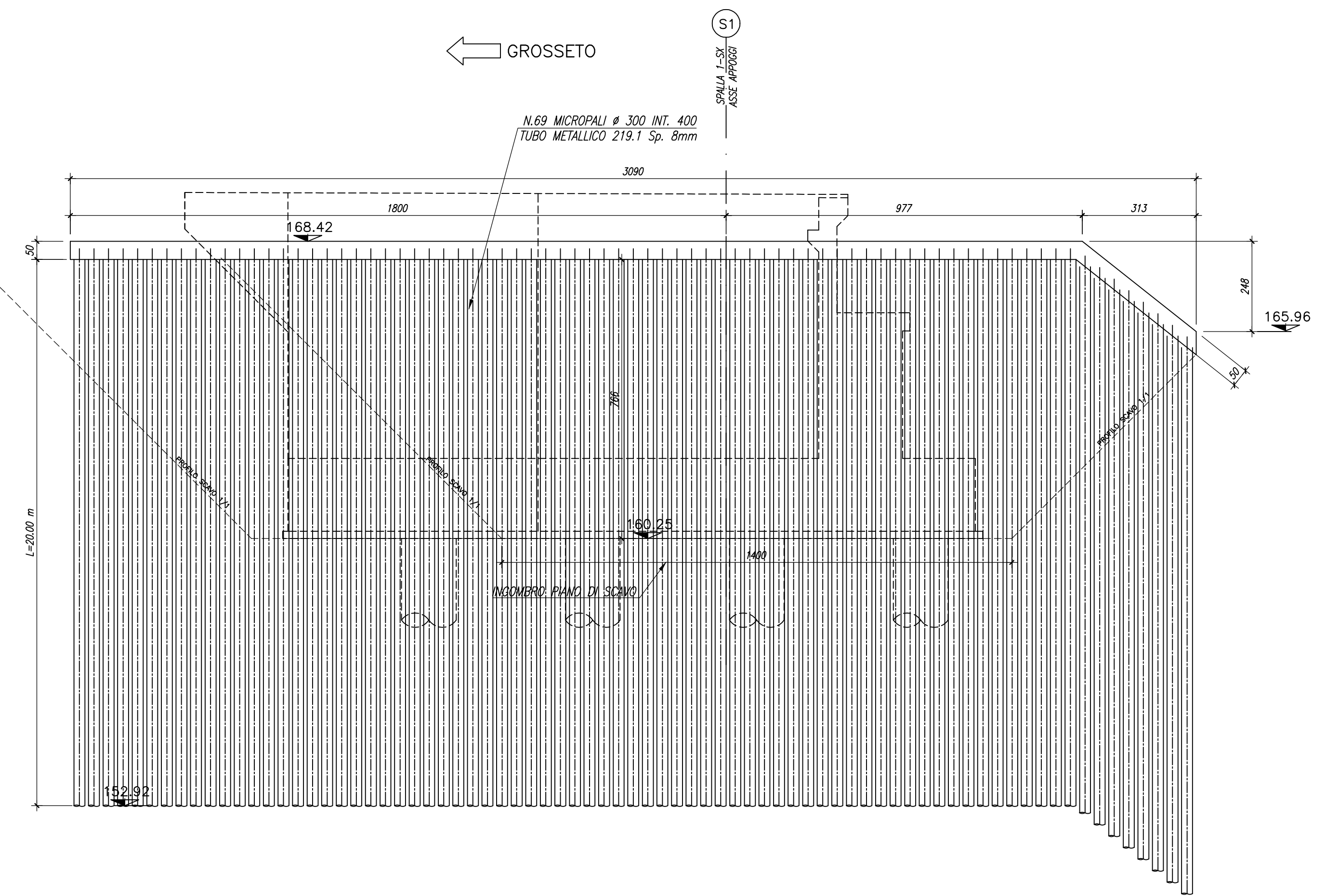
PROSPETTO PARATIA PROVVISORIALE SPALLA S1 Scala 1:100
