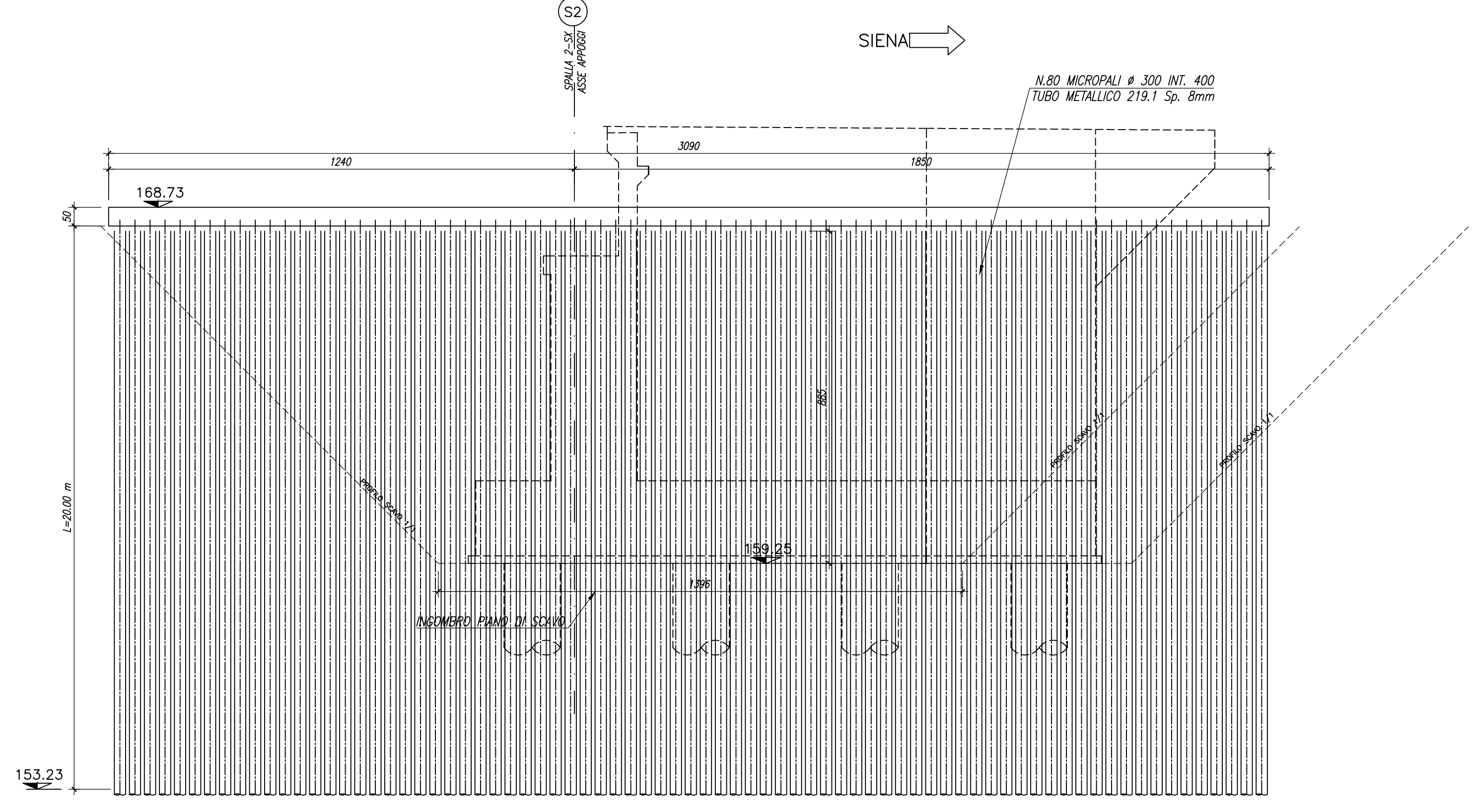
PROSPETTO PARATIA PROVVISORIALE SPALLA S2 Scala 1:100
