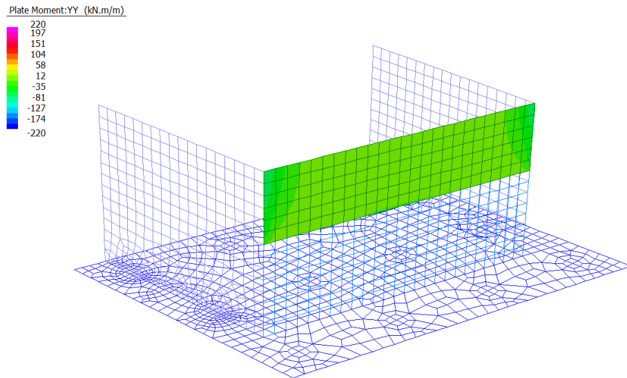
Figura 31: Momento Flettente orizzontale - Inviluppo SLE
