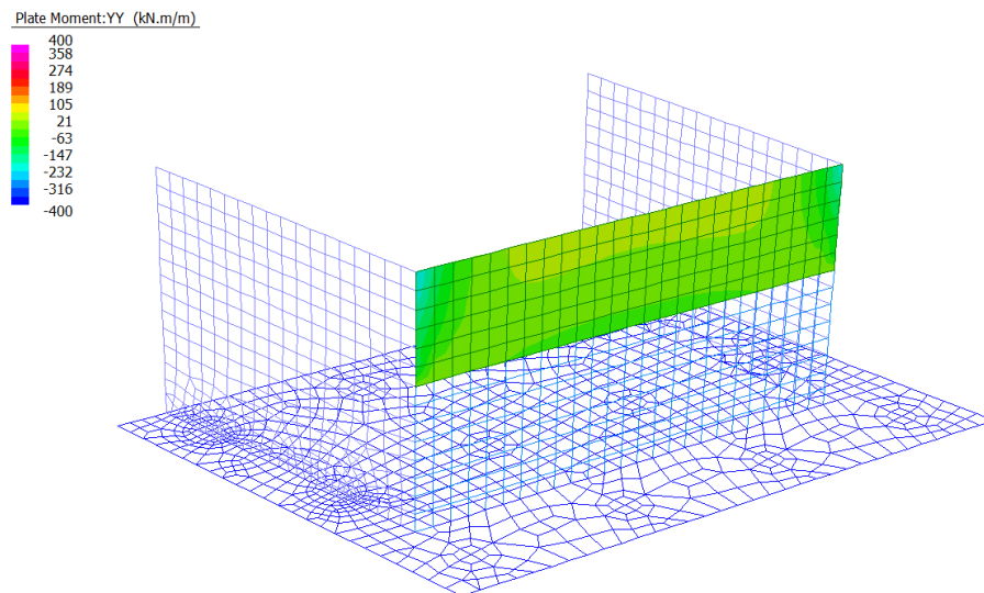
Figura 32: Momento Flettente orizzontale - Inviluppo SLU/SLV
