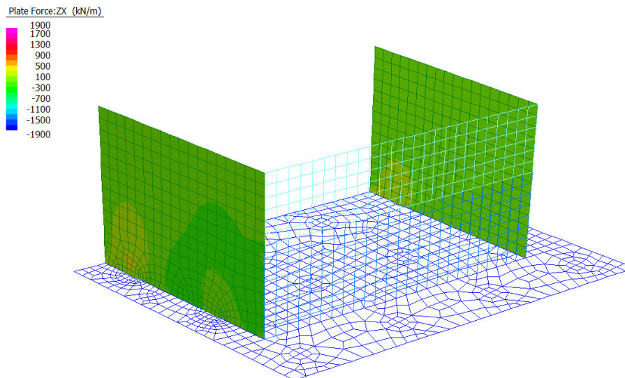
Figura 24: Sollecitazioni Taglianti Vxz - Inviluppo SLU/SLV
