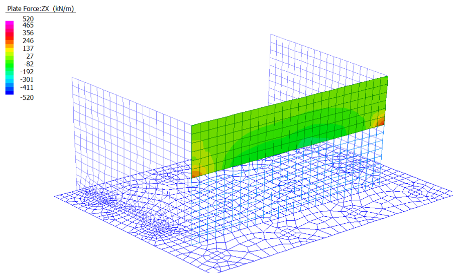
Figura 30: Sollecitazioni Taglianti Vxz - Inviluppo SLU/SLV
