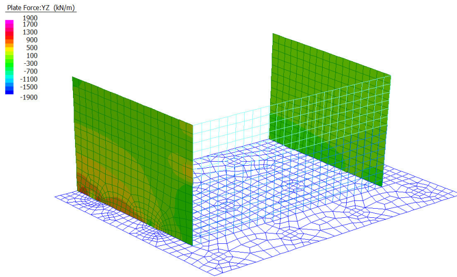
Figura 23: Sollecitazioni Taglianti Vyz - Inviluppo SLU/SLV
