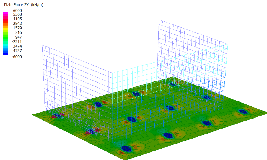
Figura 36: Sollecitazioni Taglianti Vxz- Inviluppo SLU/SLV
