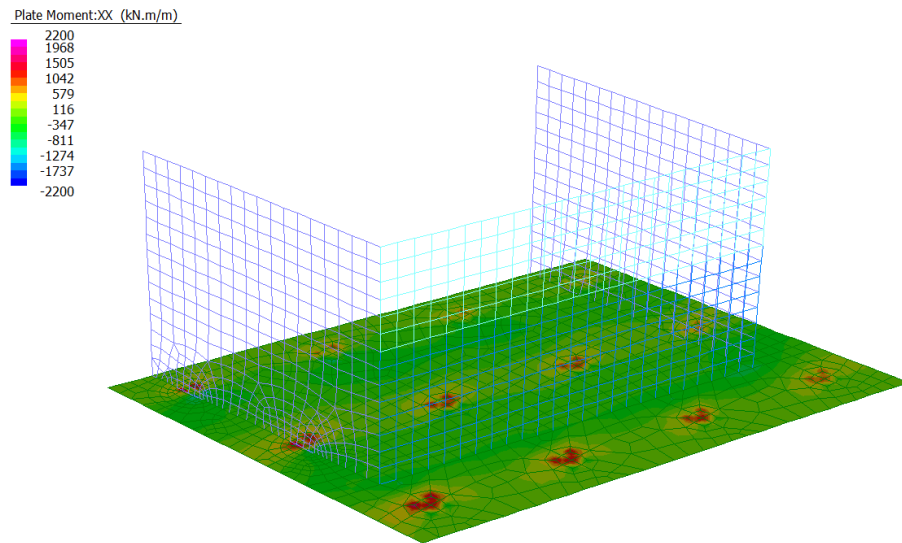
Figura 37: Momento Flettente longitudinale - Involuppo SLE
