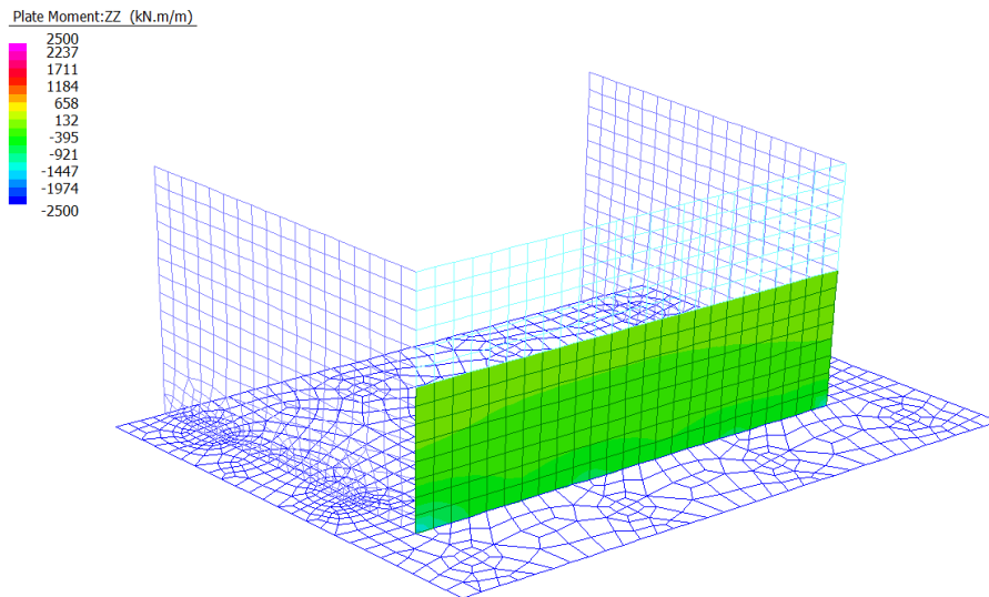
Figura 15: Momento Flettente verticale - Inviluppo SLE
