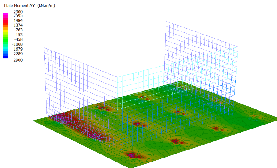
Figura 34: Momento Flettente trasversale - Involuppo SLU/SLV
