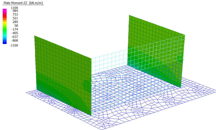
Figura 21: Momento Flettente verticale - Inviluppo SLE
