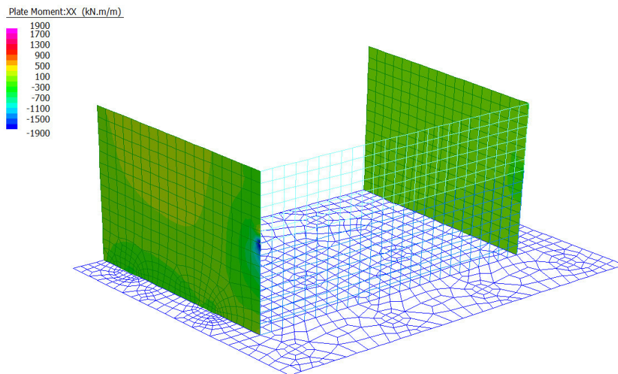
Figura 26: Momento Flettente orizzontale - Involuppo SLU/SLV
