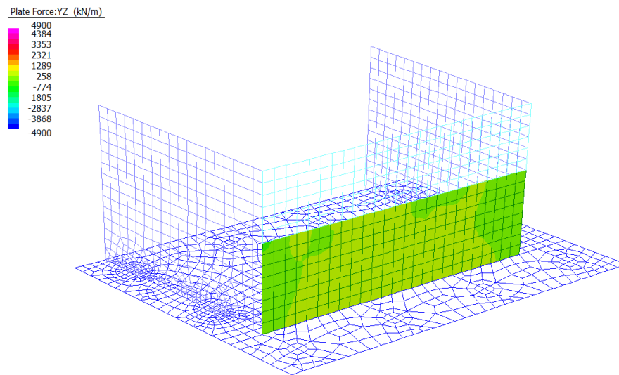
Figura 17: Sollecitazioni Taglianti Vyz - Involuppo SLU/SLV
