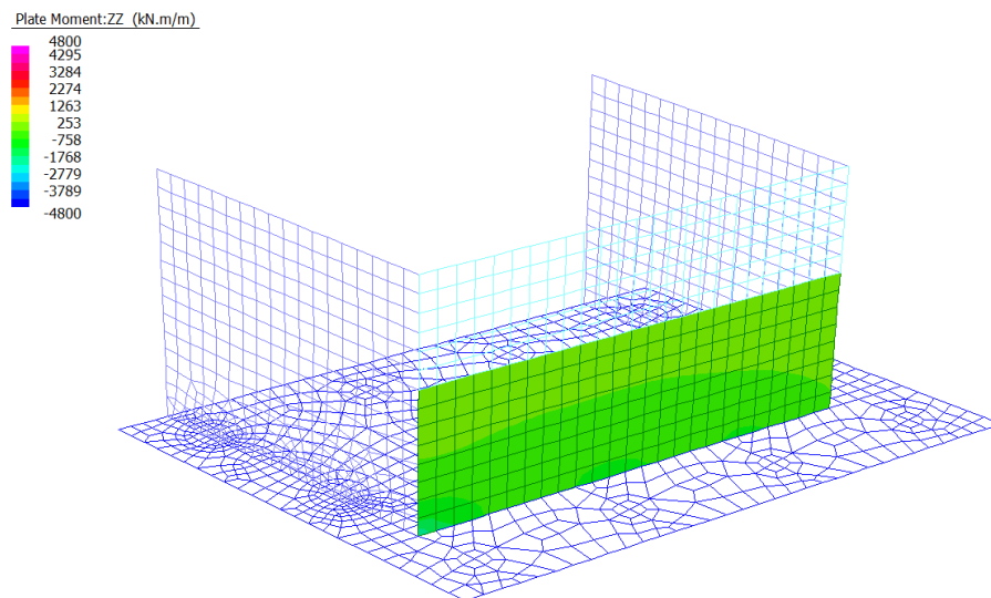
Figura 16: Momento Flettente verticale - Inviluppo SLU/SLV
