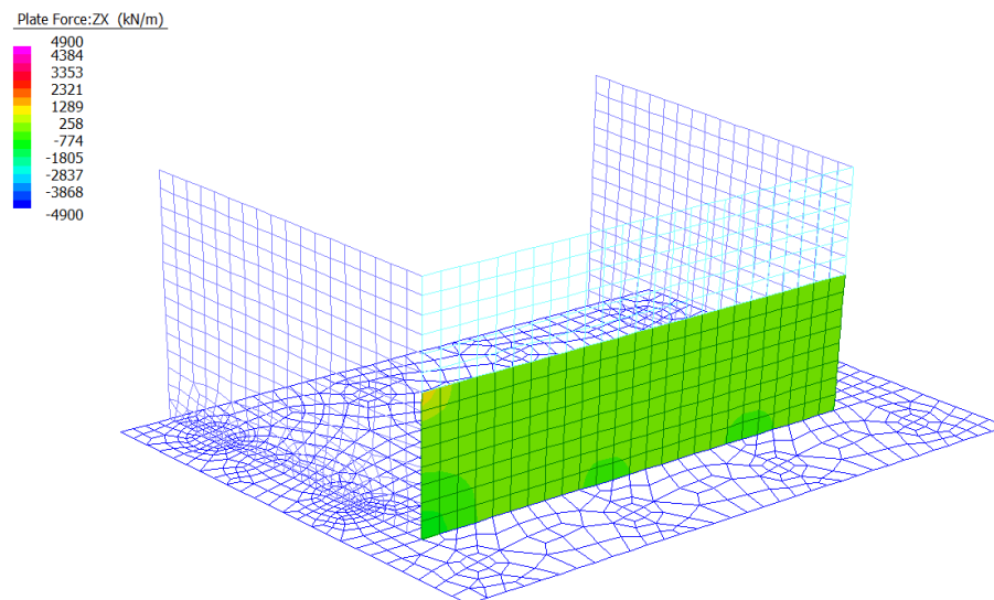
Figura 18: Sollecitazioni Taglianti Vxz - Involuppo SLU/SLV
