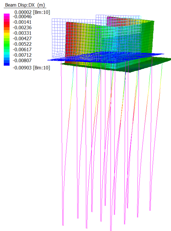
Figura 11: Valutazione spostamenti dell'opera
