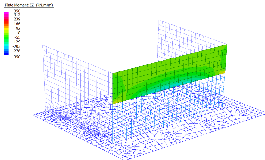
Figura 28: Momento Flettente verticale - Inviluppo SLU/SLV
