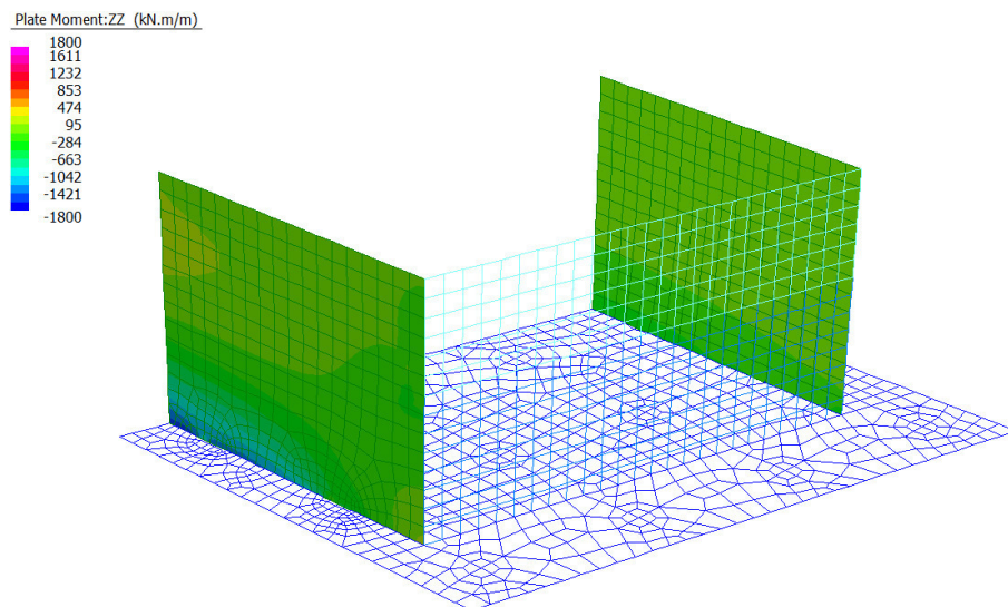
Figura 22: Momento Flettente verticale - Inviluppo SLU/SLV
