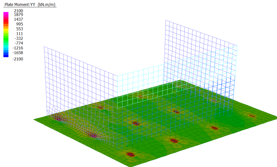
Figura 33: Momento Flettente trasversale - Involuppo SLE
