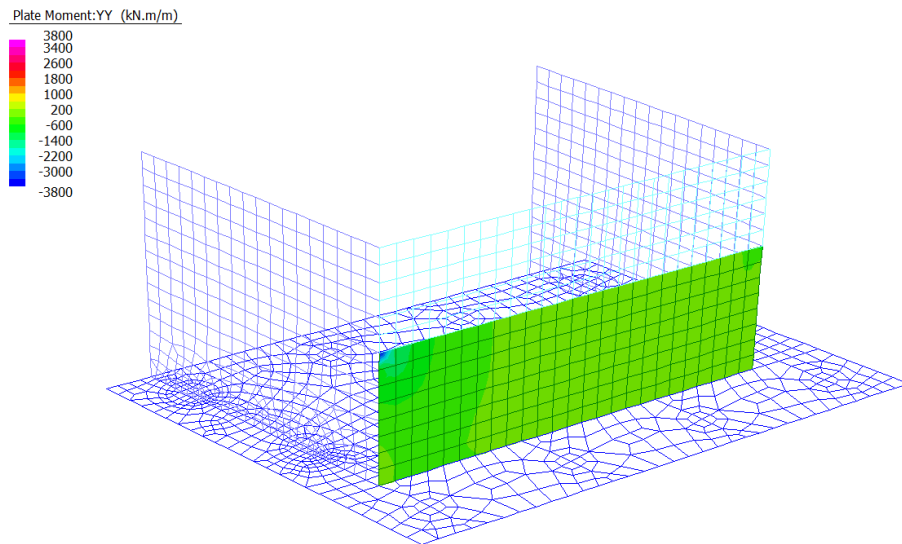
Figura 20: Momento Flettente orizzontale - Involuppo SLU/SLV
