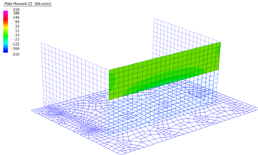
Figura 27: Momento Flettente verticale - Inviluppo SLE
