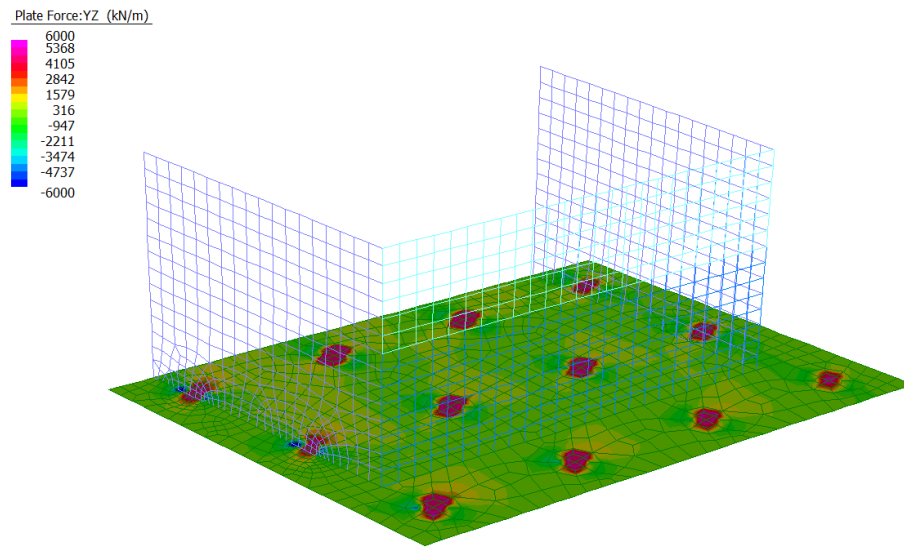
Figura 35: Sollecitazioni Taglianti Vyz- Inviluppo SLU/SLV
