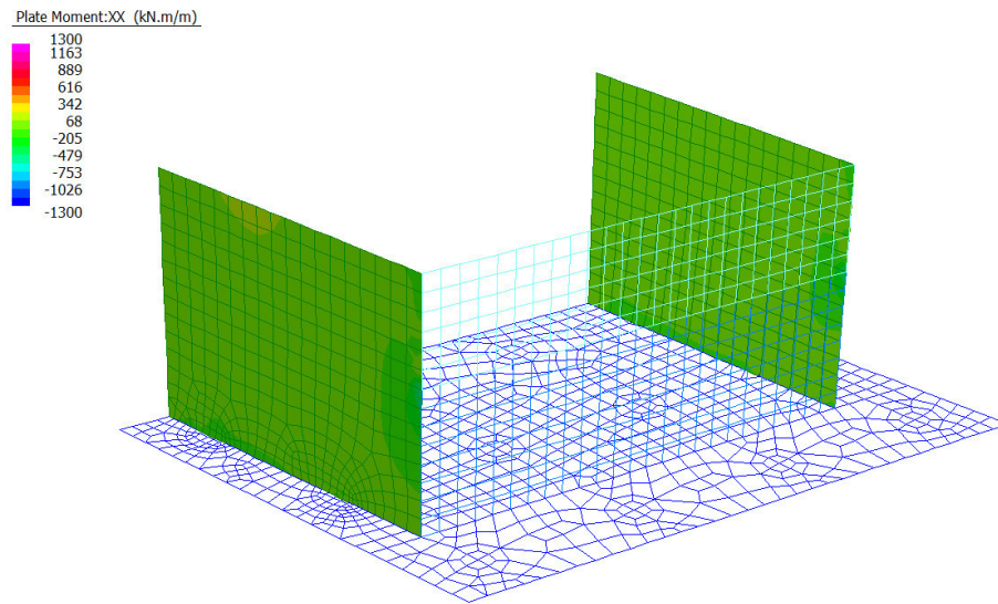
Figura 25: Momento Flettente orizzontale - Involuppo SLE
