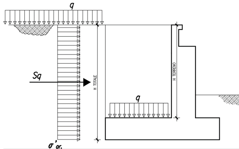
Figura 9: Schema per il calcolo degli effetti della spinta dovuta al sovraccarico accidentale
