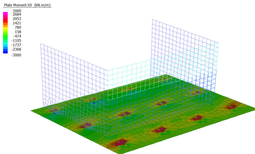
Figura 38: Momento Flettente longitudinale - Involuppo SLU/SLV
