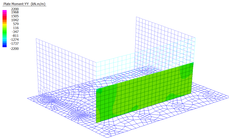
Figura 19: Momento Flettente orizzontale - Involuppo SLE
