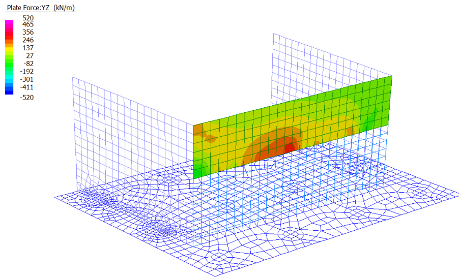
Figura 29: Sollecitazioni Taglianti Vyz - Inviluppo SLU/SLV
