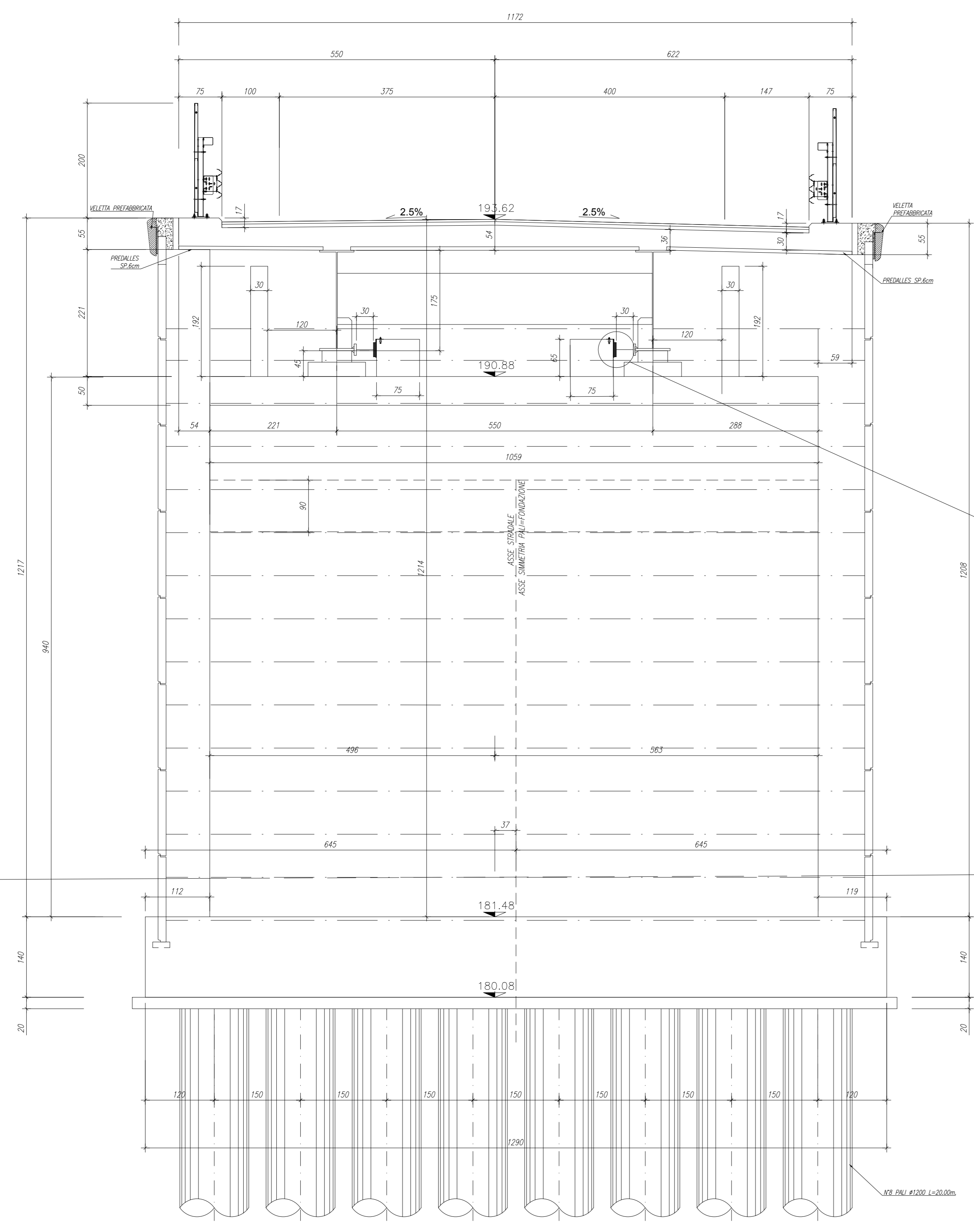
VISTA FRONTALE SPALLA 1 Scala 1:50
