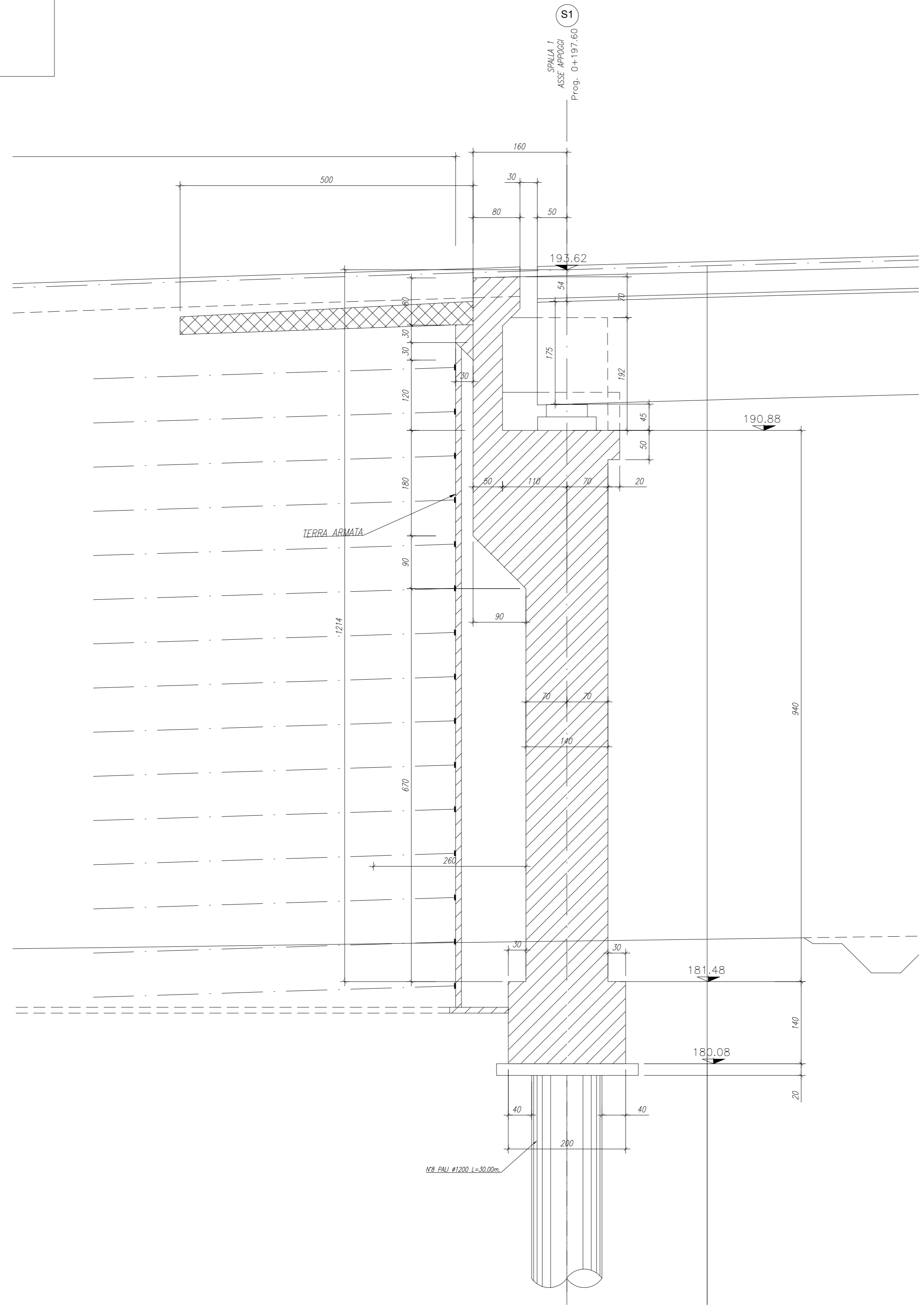
SEZIONE SPALLA 1 Scala 1:50
