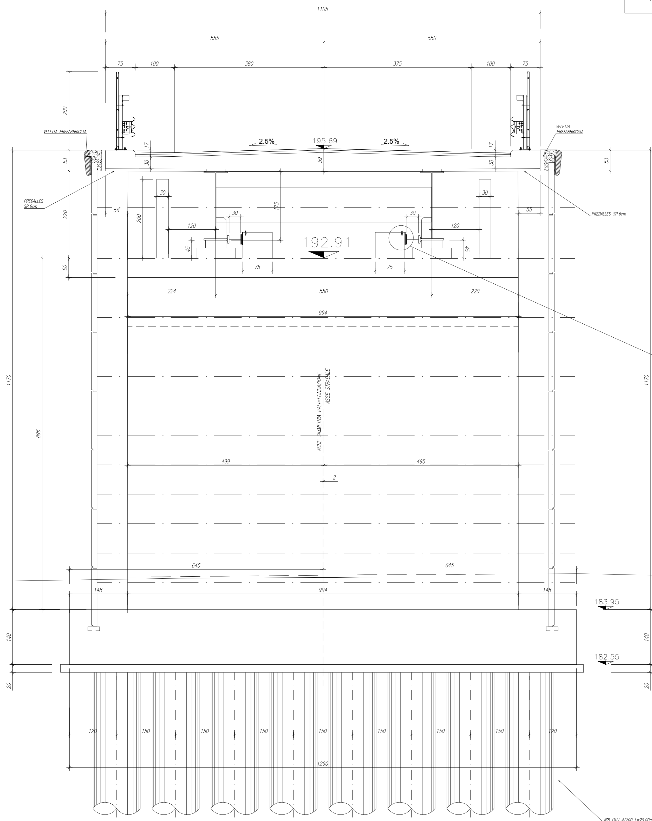
VISTA FRONTALE SPALLA 2 Scala 50
