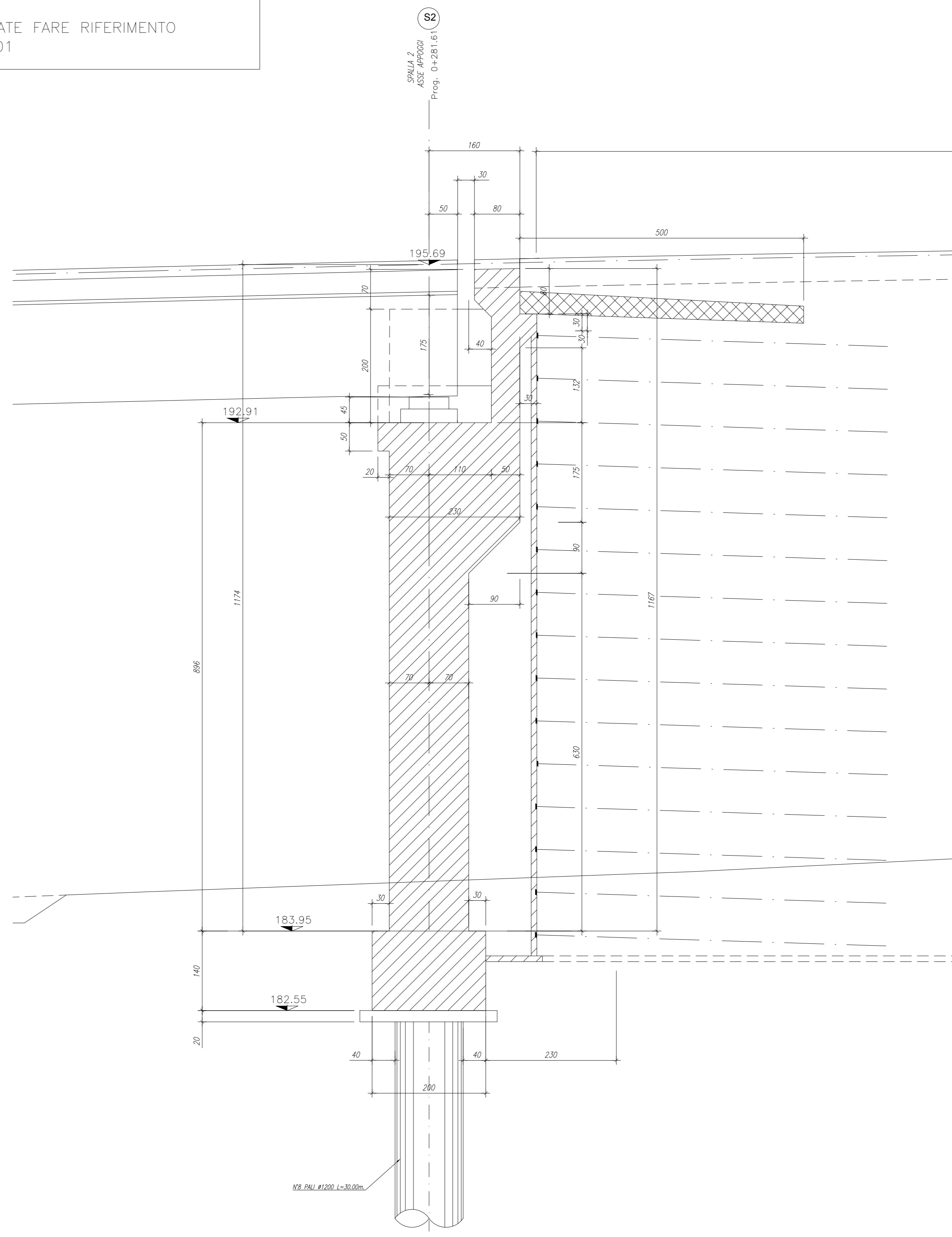
SEZIONE SPALLA 2 Scala 1:50
