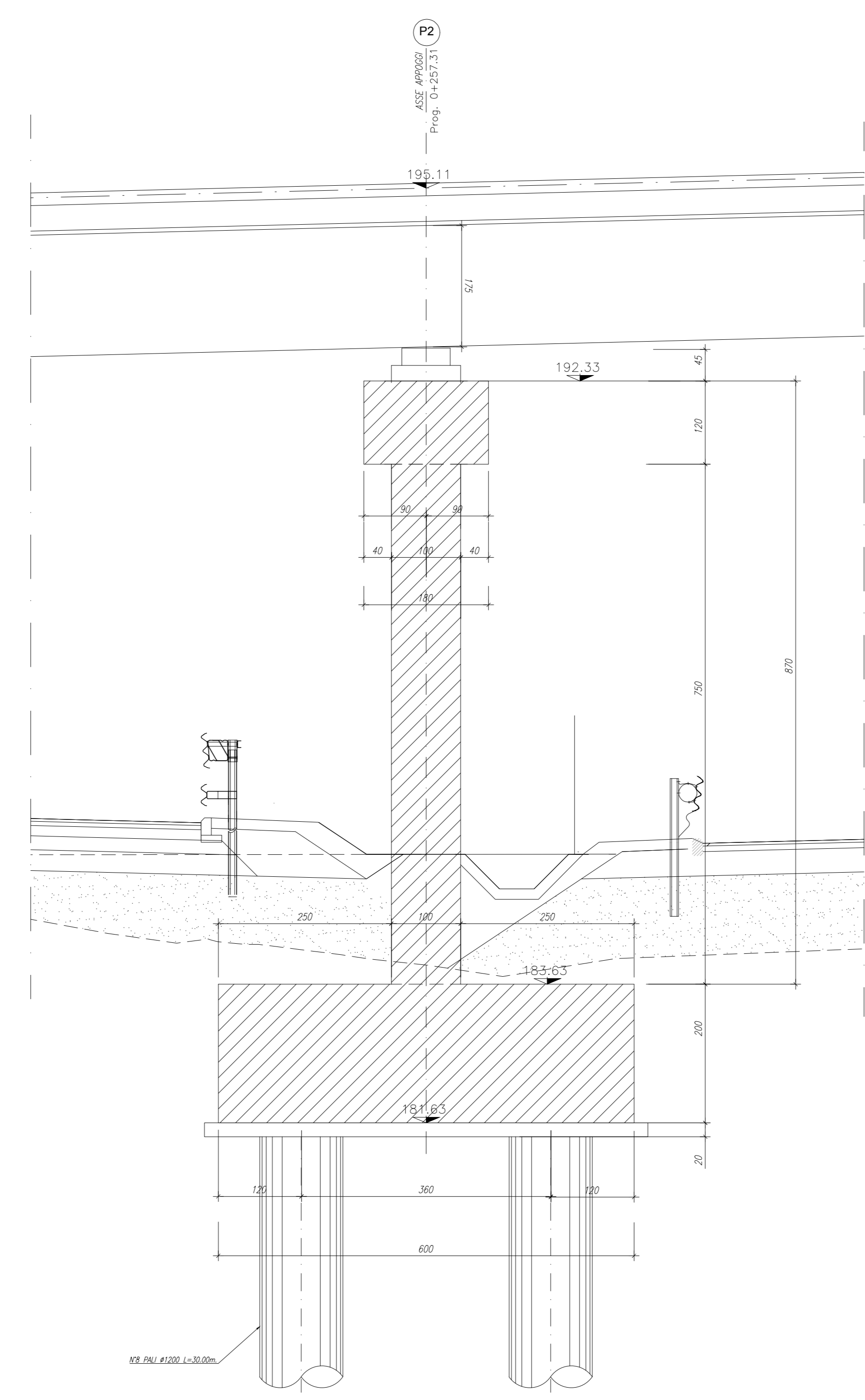
SEZIONE PILA 2 Scala 1:50
