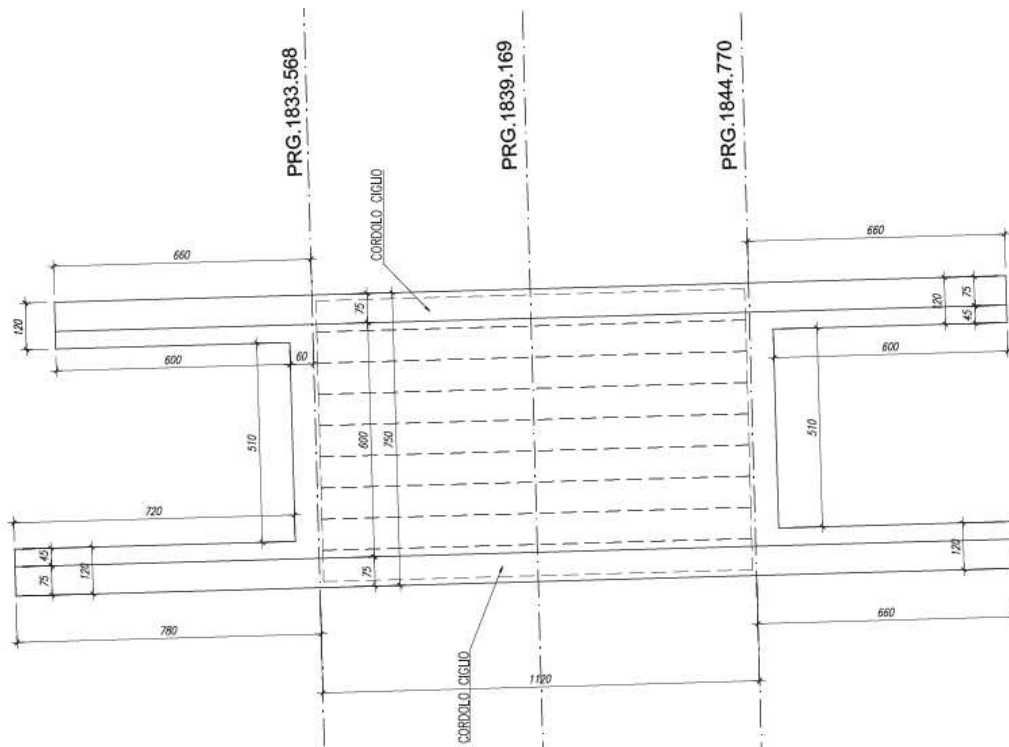
Figura 1 Pianta impalcato
