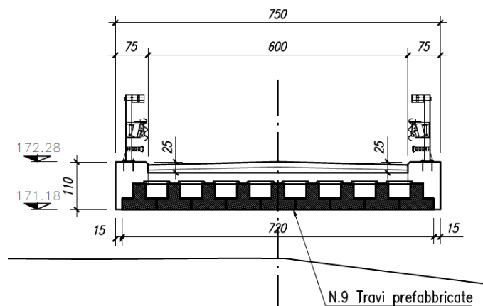
Figura 2 Sezione trasversale in asse
