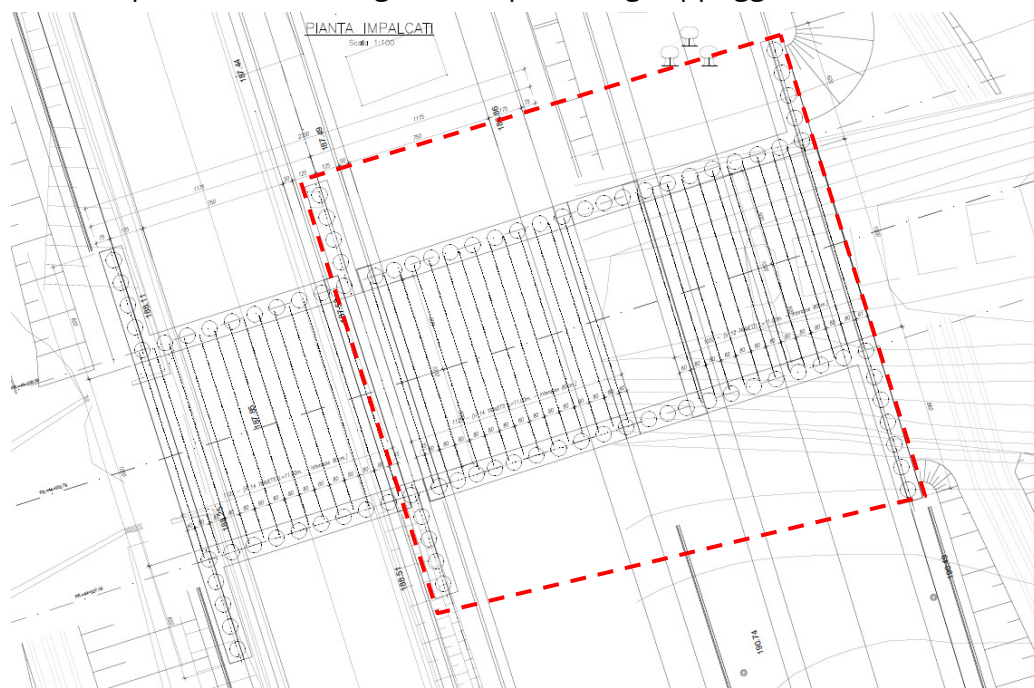
Figura 1 Pianta impalcato
