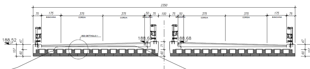
Figura 2 Sezione trasversale in asse
