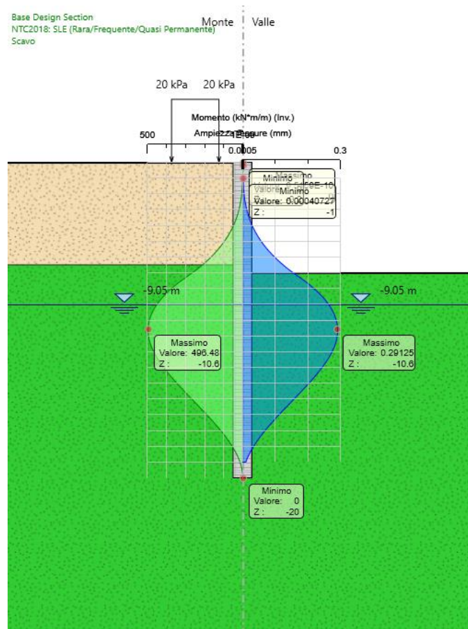
Figura 6: Modello SLE: verifica a fessurazione
