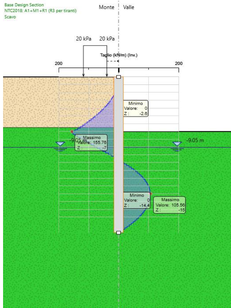
Figura 3: Modelli SLU: Involuppo Diagramma del Taglio
