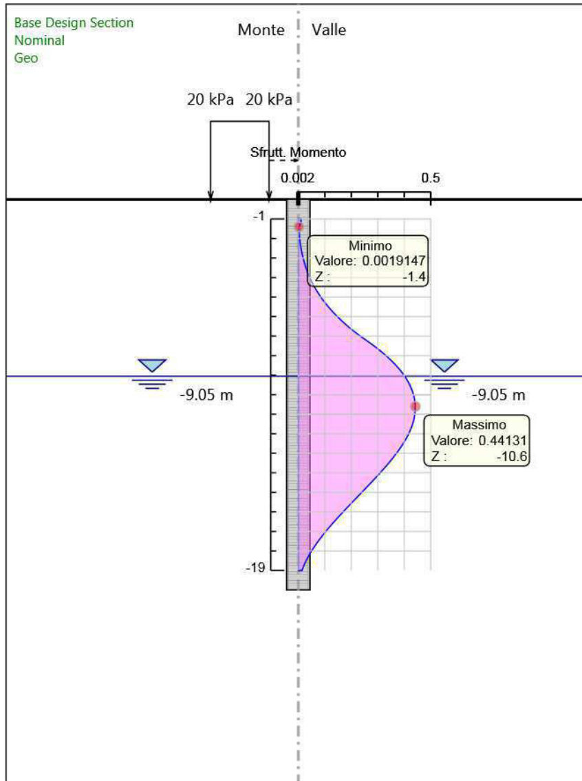
Involuppi Tasso di Sfruttamento a Momento - Cover
