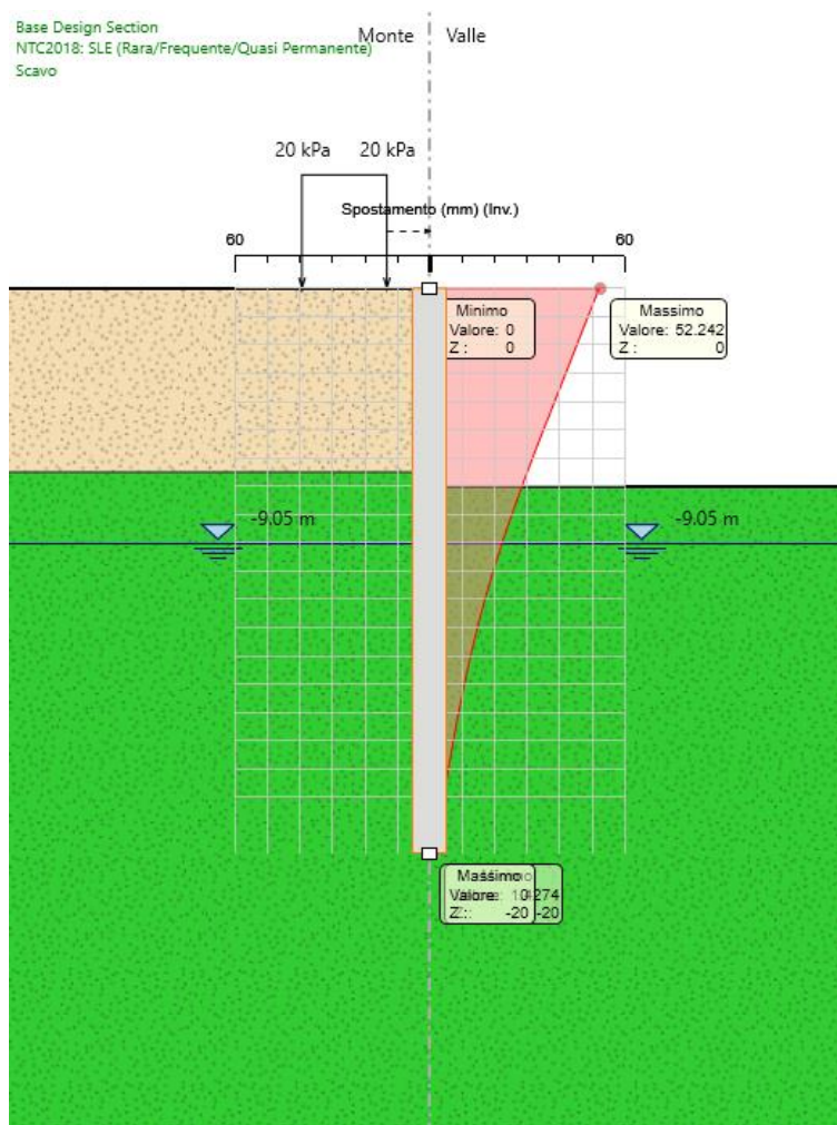
Figura 4: Modello SLE: Inviluppo degli spostamenti
