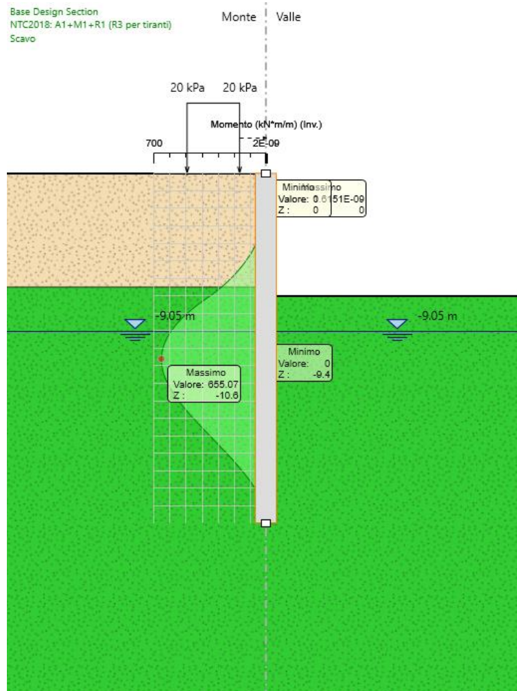
Figura 2: Modelli SLU: Involuppo Diagramma del Momento
