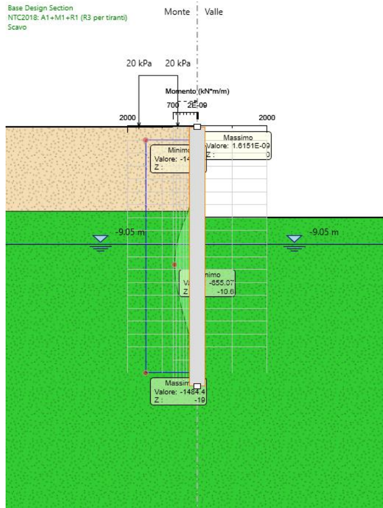
Figura 7: Modello SLU: Verifica flessionale
