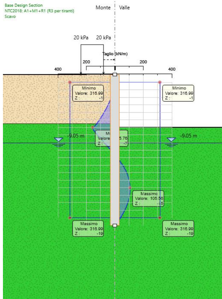
Figura 8: Modello SLU: Verifica a taglio
