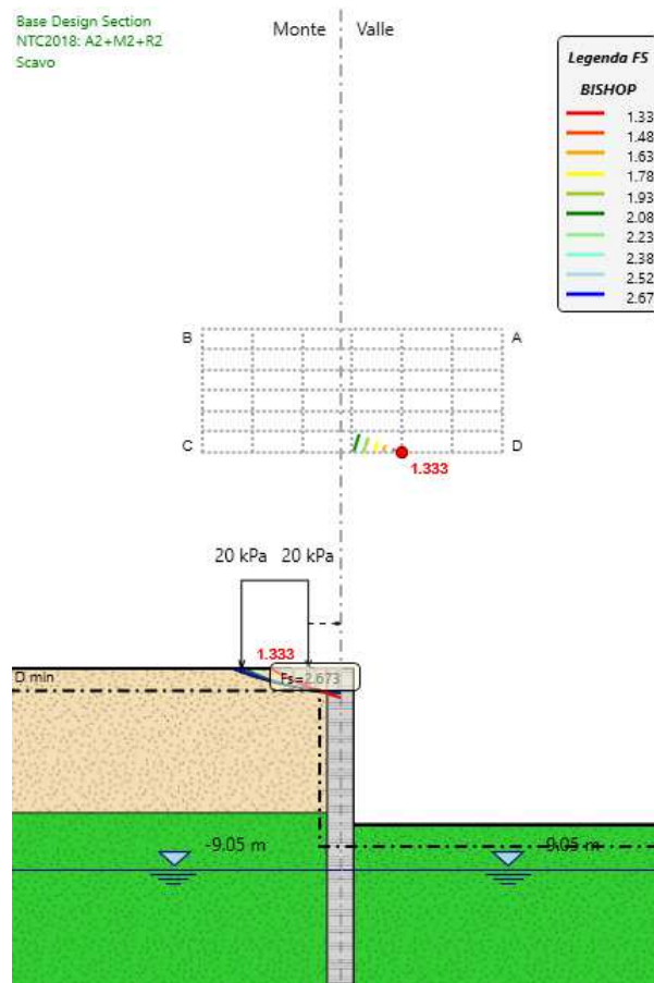
Figura 5: Risultati dell’analisi di stabilità globale
