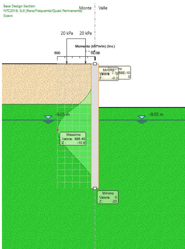
Figura 1: Modello SLE: Involuppo Diagramma del Momento
