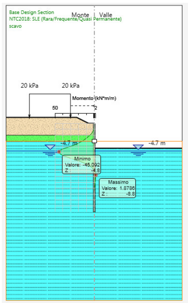
Figura 1: Modello SLE: Involuppo Diagramma del Momento
