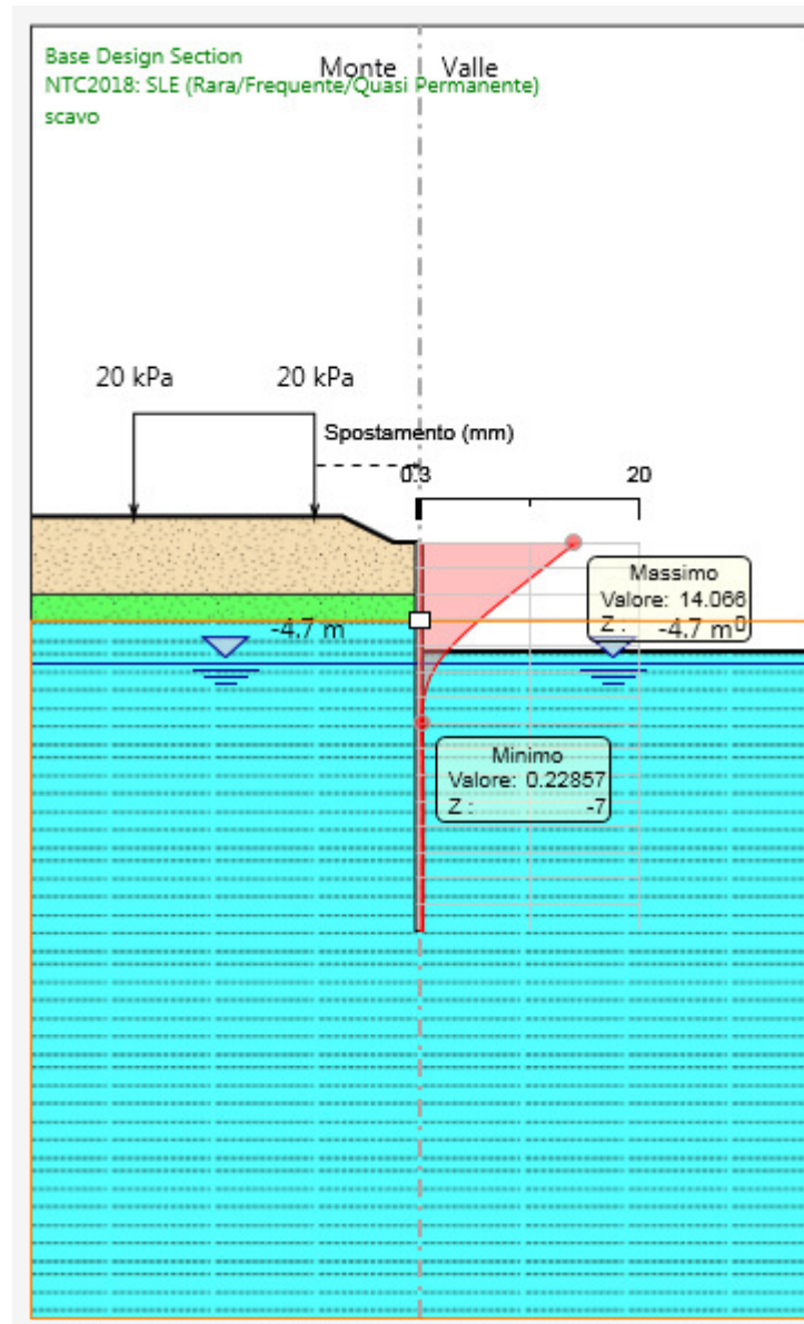
Figura 4: Modello SLE: Involuppo degli spostamenti
