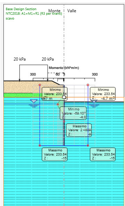
Figura 6: Modello SLU: Verifica flessionale
