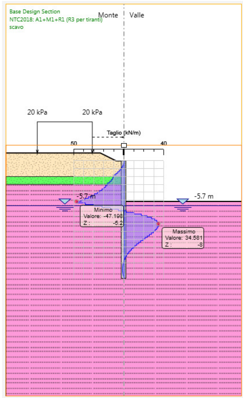
Figura 3: Modelli SLU: Inviluppo Diagramma del Taglio
