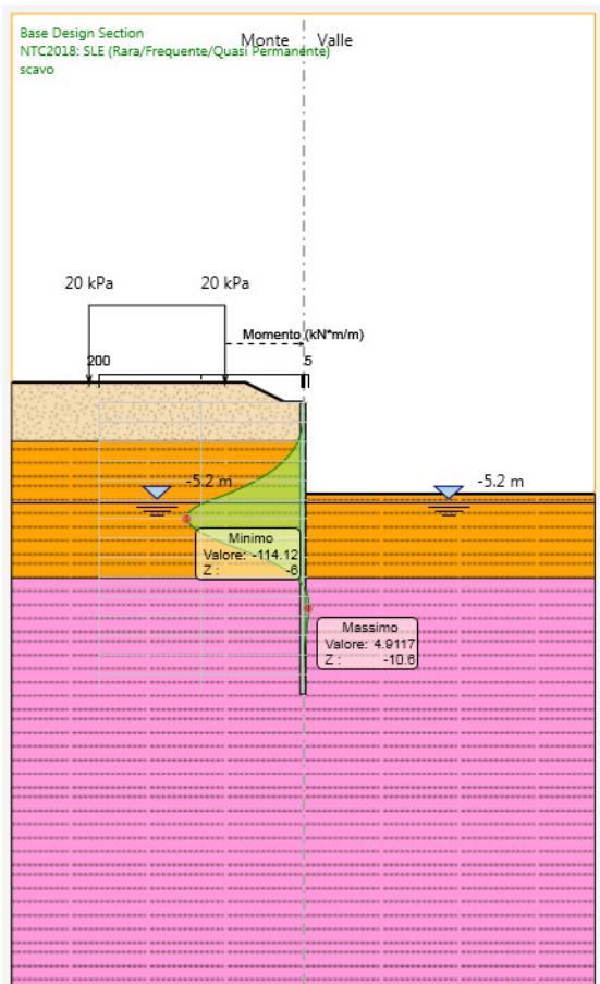
Figura 1: Modello SLE: Inviluppo Diagramma del Momento
