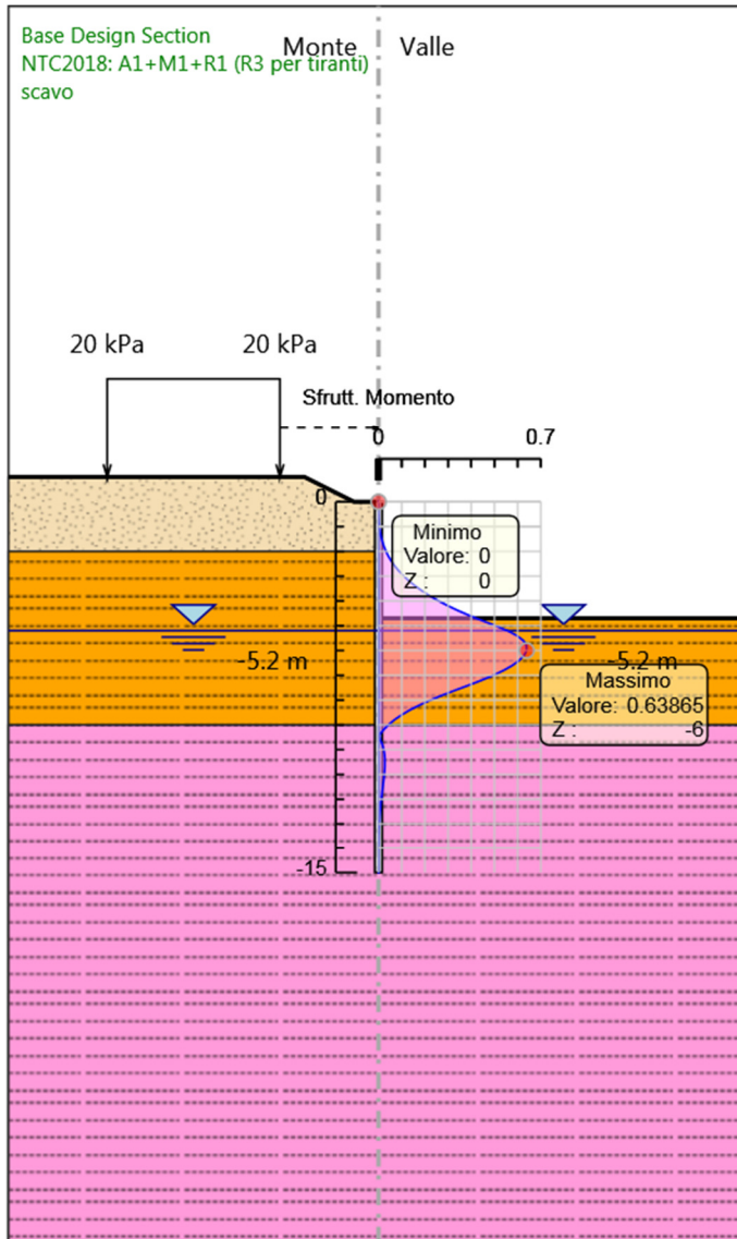
Involupi Tasso di Sfruttamento a Momento - SteelWorld
