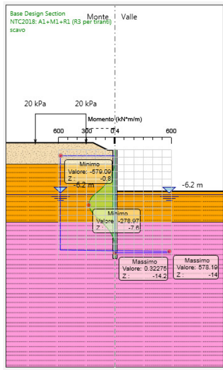
Figura 7: Modello SLU: Verifica flessionale
