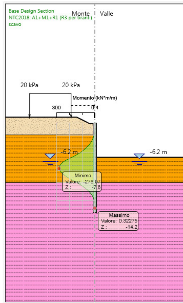
Figura 2: Modelli SLU: Involuppo Diagramma del Momento
