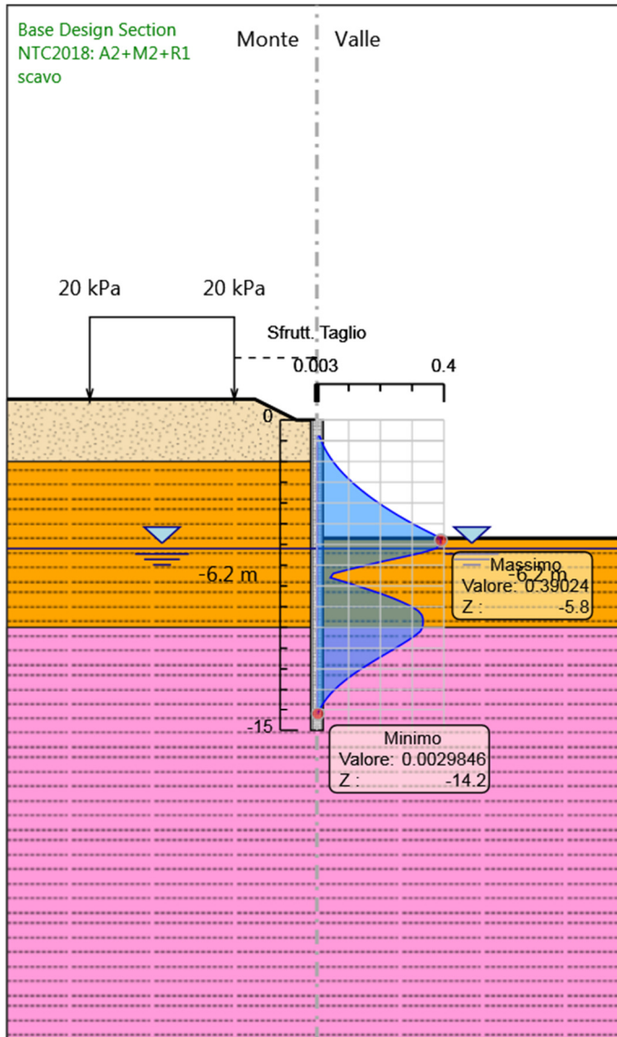
Involuppi Tasso di Sfruttamento a Taglio - Caver
