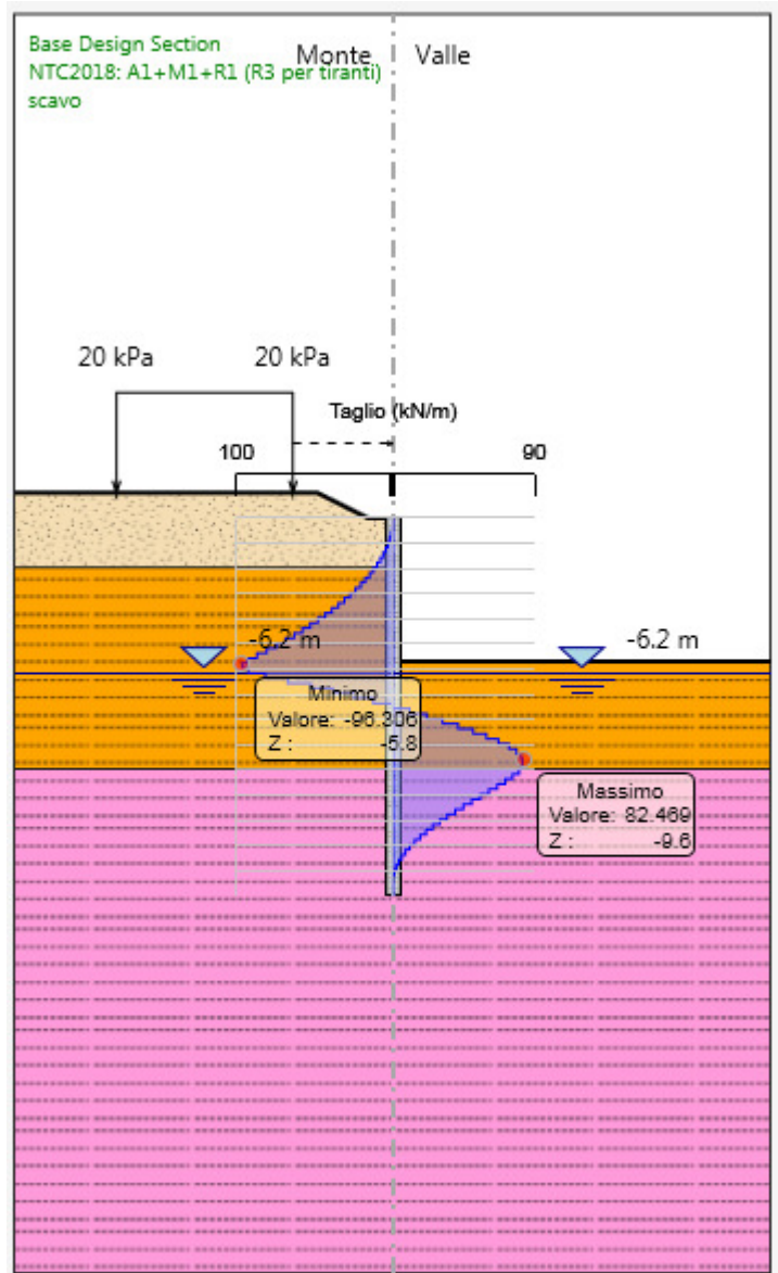
Figura 3: Modelli SLU: Inviluppo Diagramma del Taglio
