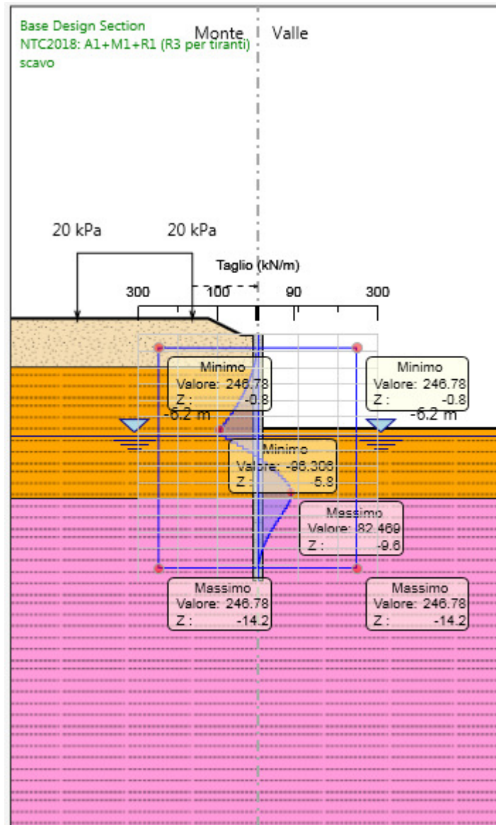
Figura 8: Modello SLU: Verifica a taglio
