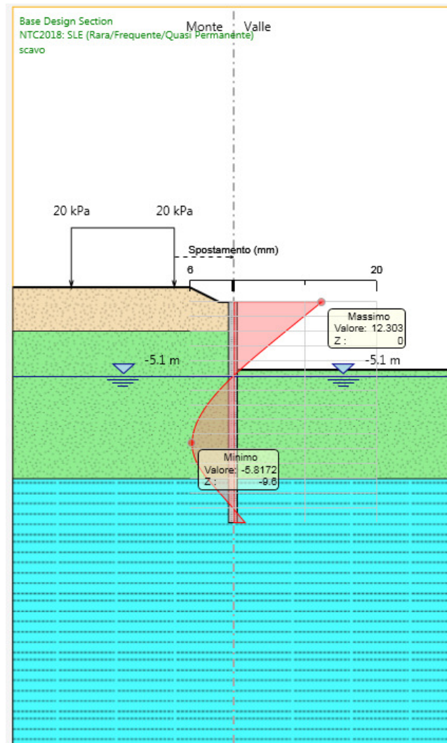
Figura 4: Modello SLE: Involuppo degli spostamenti
