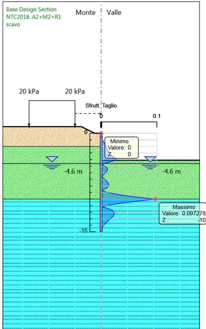
Involuppi Tasso di Sfruttamento a Taglio - SteelWorld
