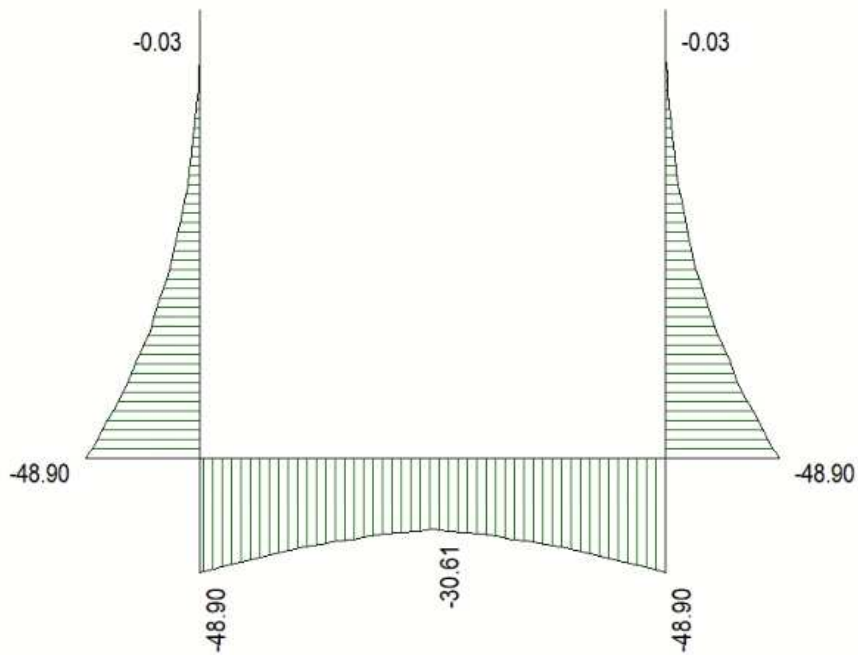
Figura 5 Involuppo SLU/Sisma: sforzo normale
