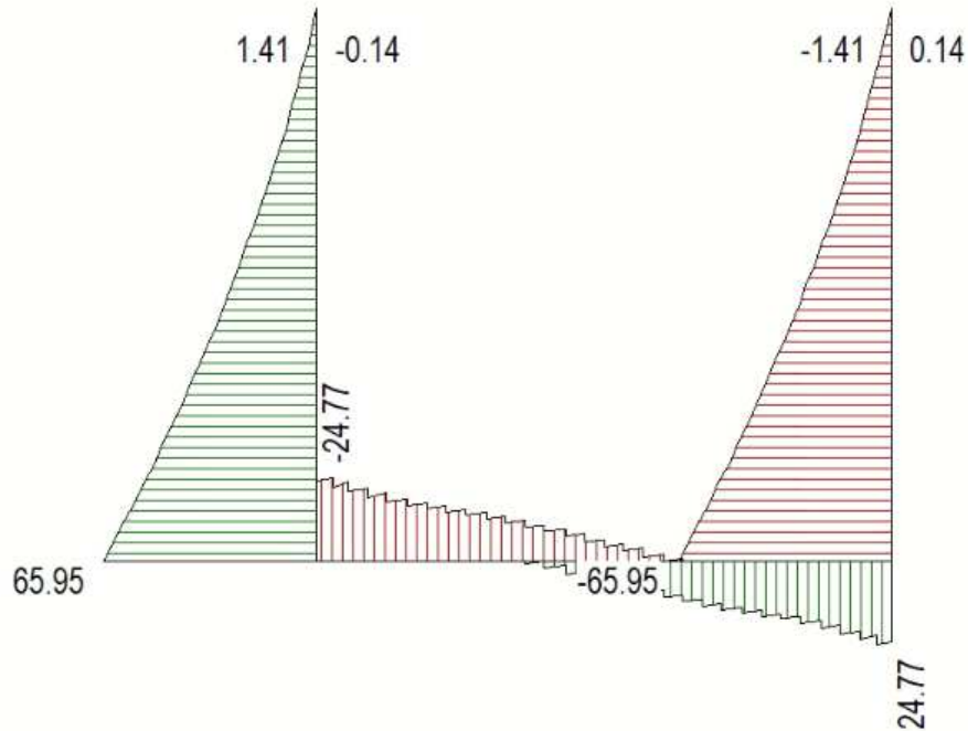
Figura 4 Involuppo SLU/Sisma: sollecitazioni taglianti
