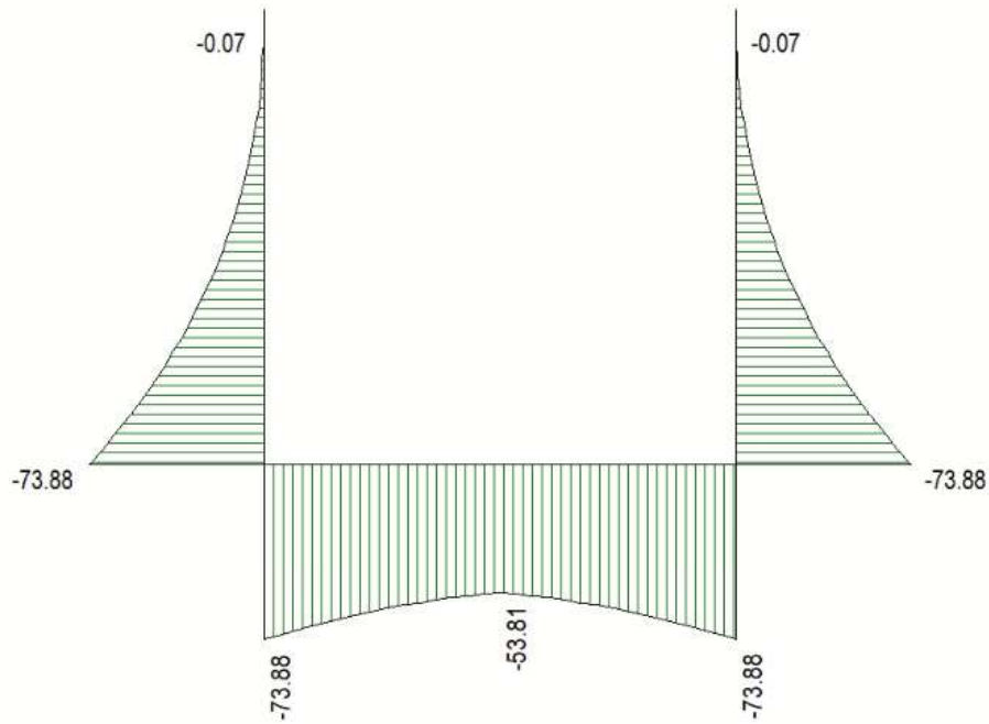
Figura 3 Involuppo SLU/Sisma: Momenti flettenti
