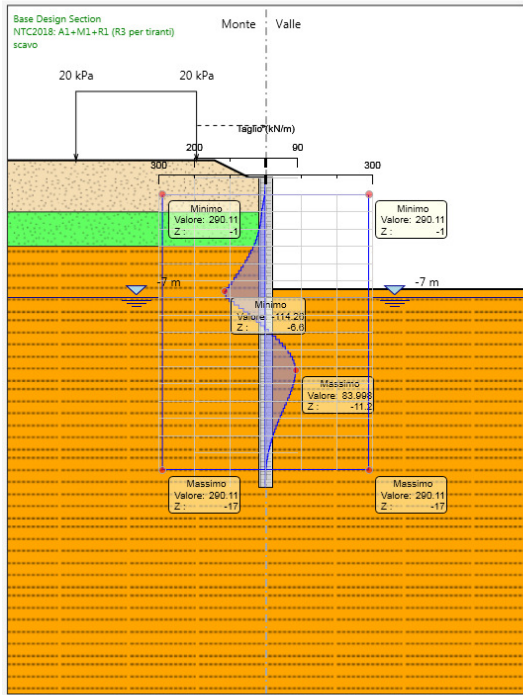
Figura 8: Modello SLU: Verifica a taglio
