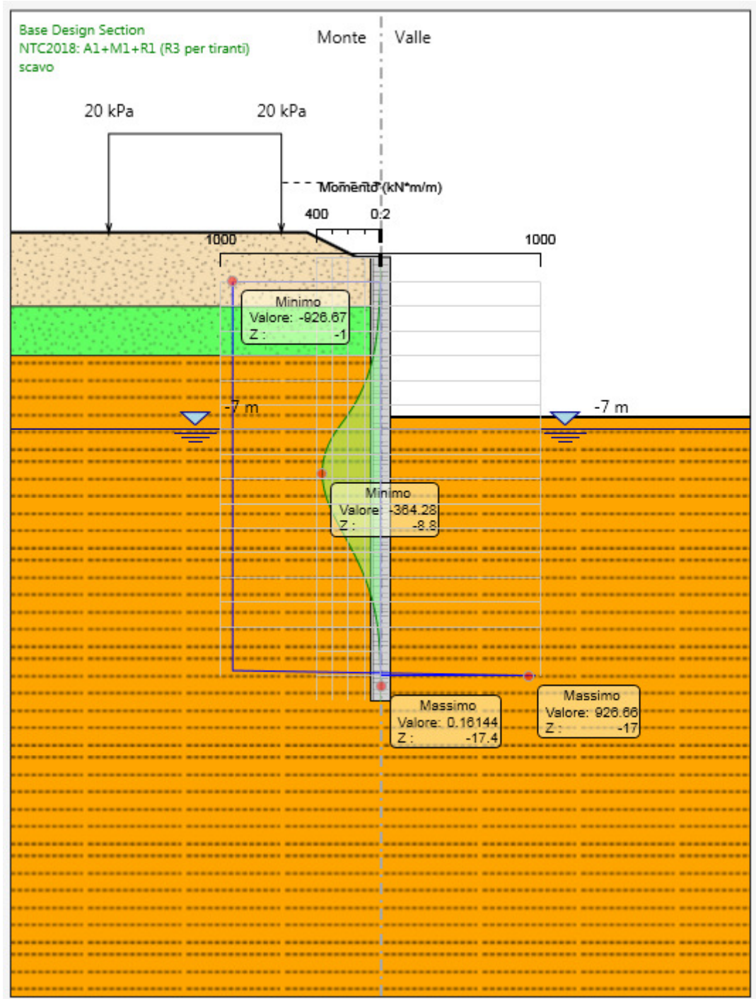
Figura 7: Modello SLU: Verifica flessionale
