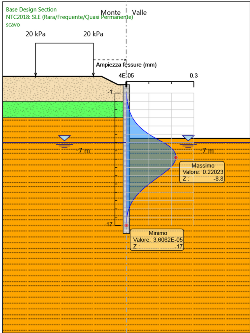
Involuppi Apertura Fessure - Cover
