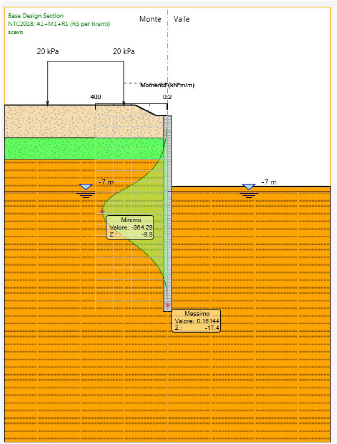
Figura 2: Modelli SLU: Involuppo Diagramma del Momento
