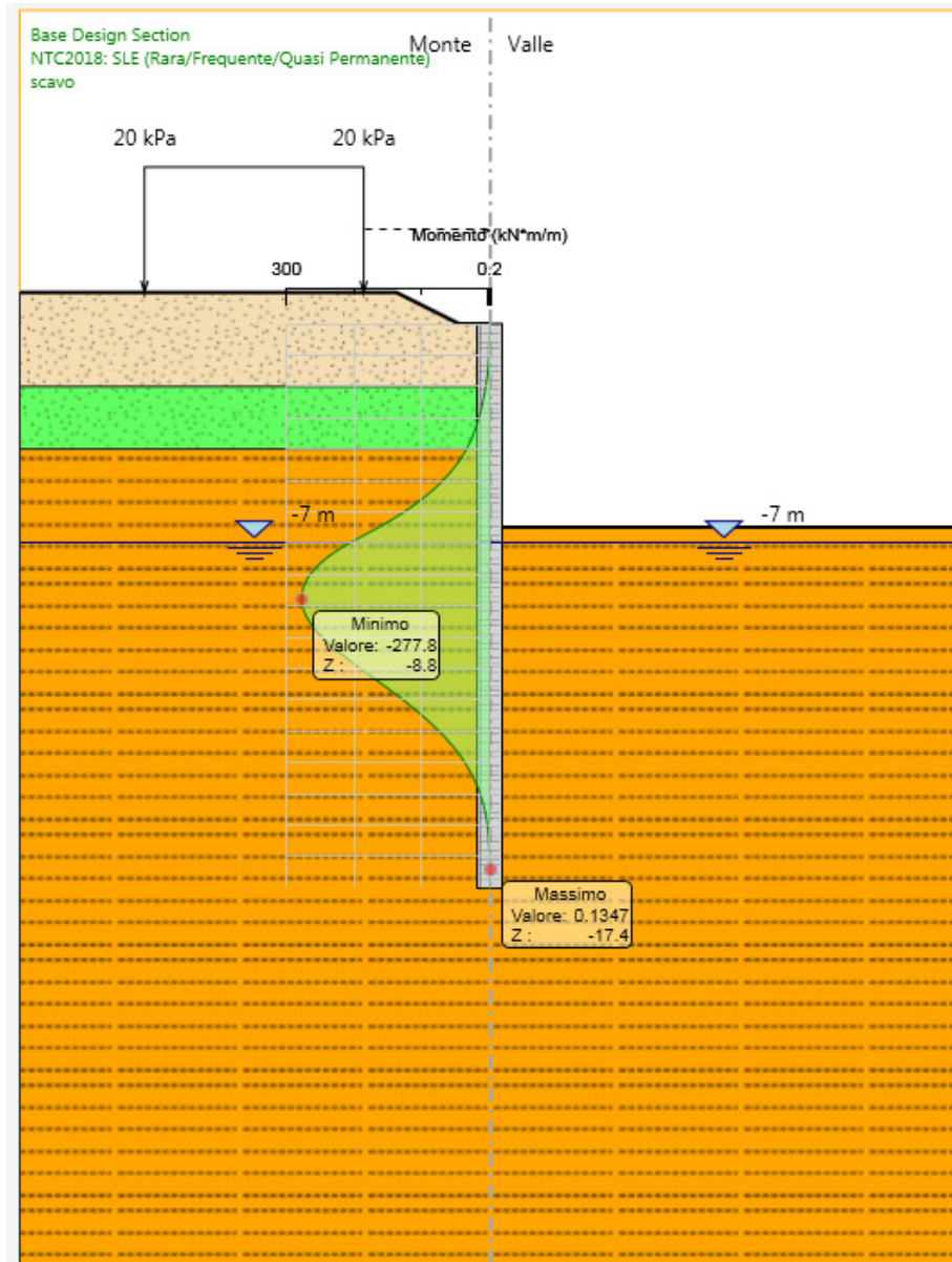
Figura 1: Modello SLE: Involuppo Diagramma del Momento
