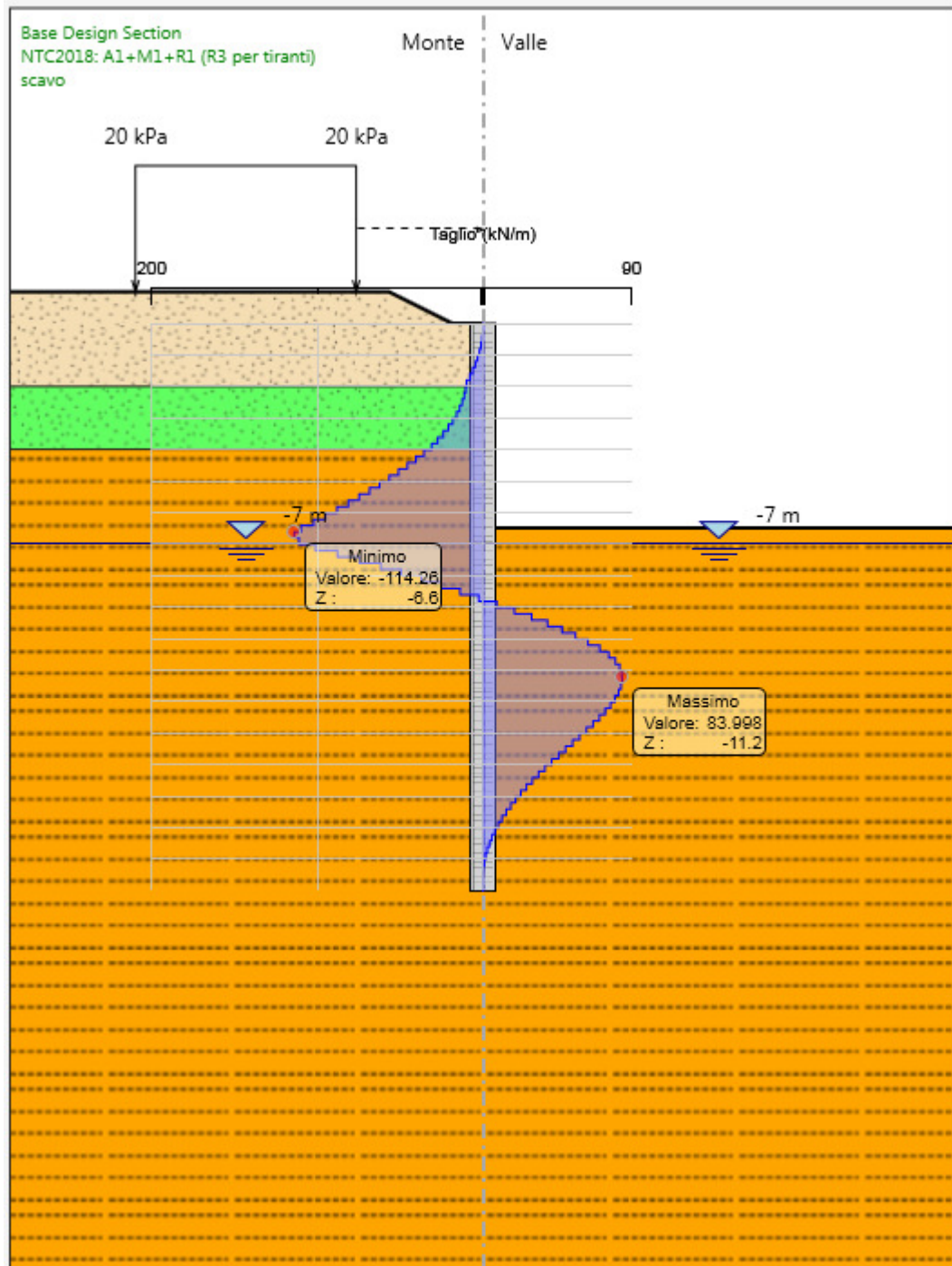
Figura 3: Modelli SLU: Involuppo Diagramma del Taglio
