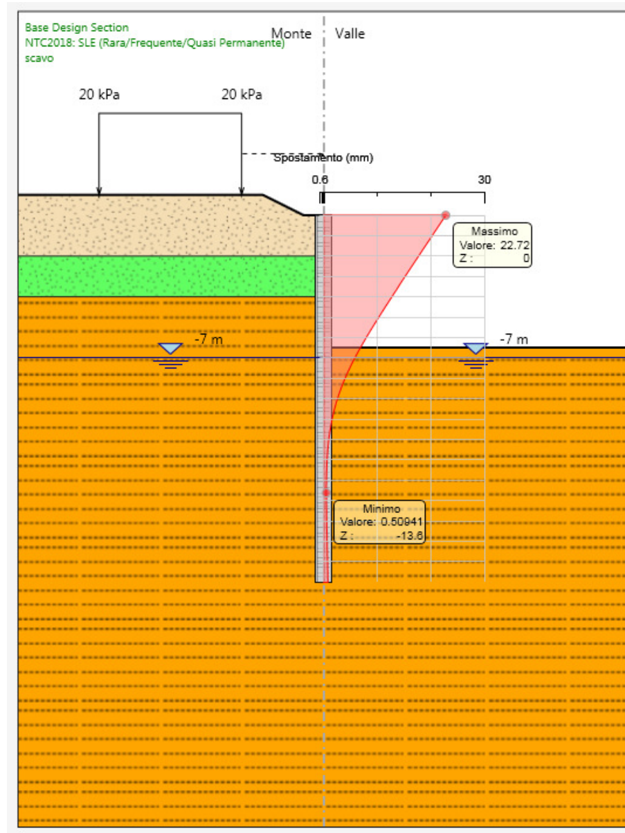
Figura 4: Modello SLE: Inviluppo degli spostamenti
