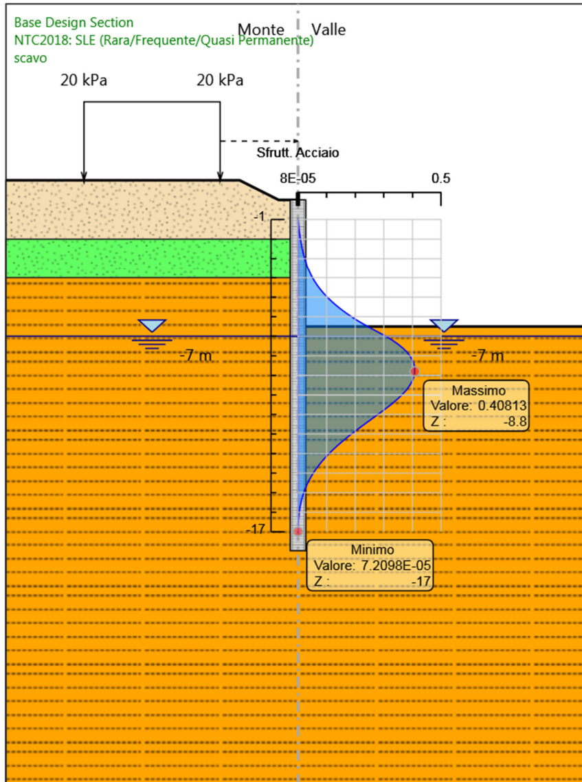
Involuppi Tasso di Sfruttamento Armature - Cover
