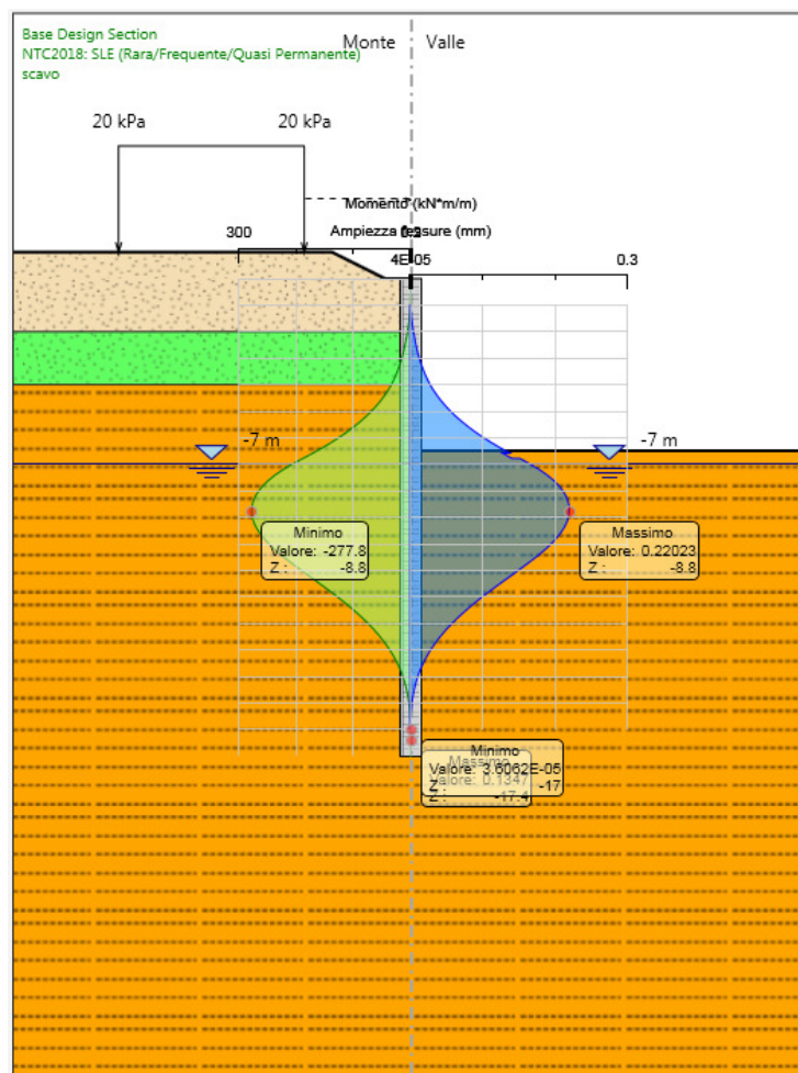
Figura 6: Modello SLE: verifica a fessurazione
