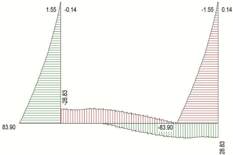
Figura 15 Inviluppo SLU/Sisma: sollecitazioni taglianti
