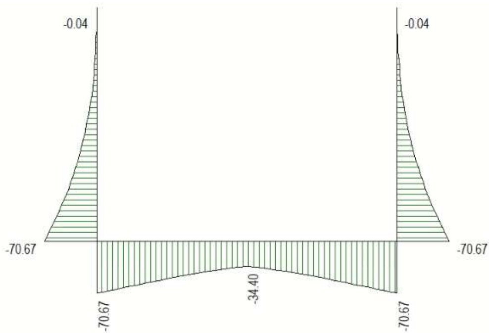
Figura 17 Inviluppo SLE Momenti flettenti
