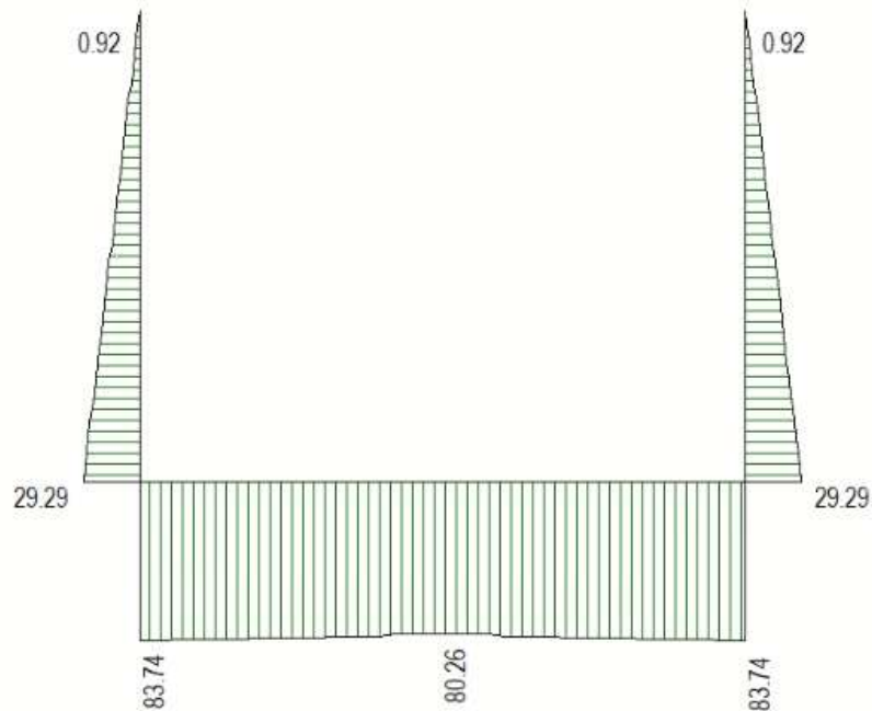
Figura 16 Inviluppo SLU/Sisma: sforzo normale
