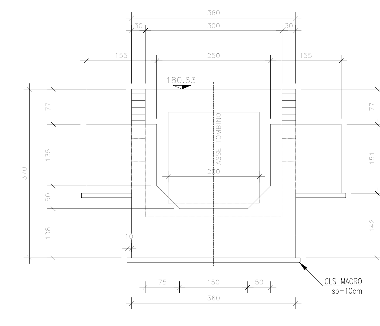
VISTA F-F Scala 1:50
