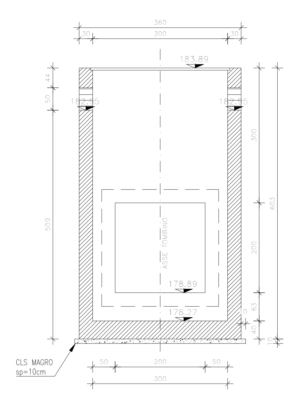
SEZIONE D-D Scala 1:50
