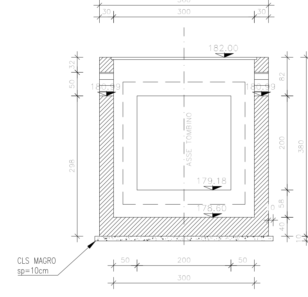
SEZIONE E-E Scala 1:50
