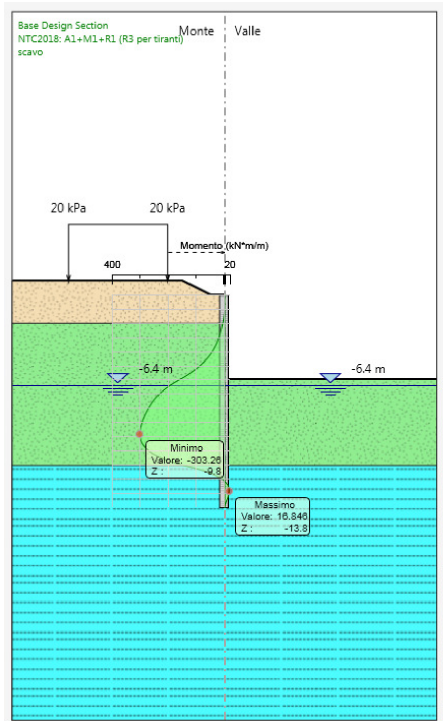
Figura 2: Modelli SLU: Involuppo Diagramma del Momento
