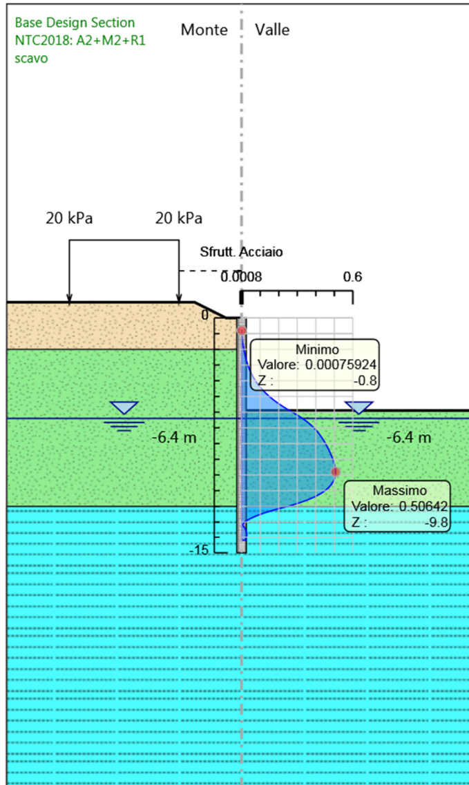
Involuppi Tasso di Sfruttamento Armature - Caver
