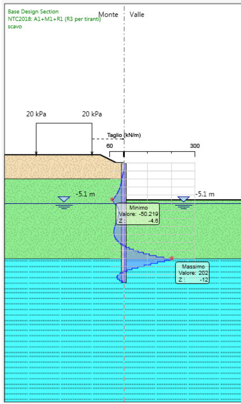
Figura 3: Modelli SLU: Inviluppo Diagramma del Taglio
