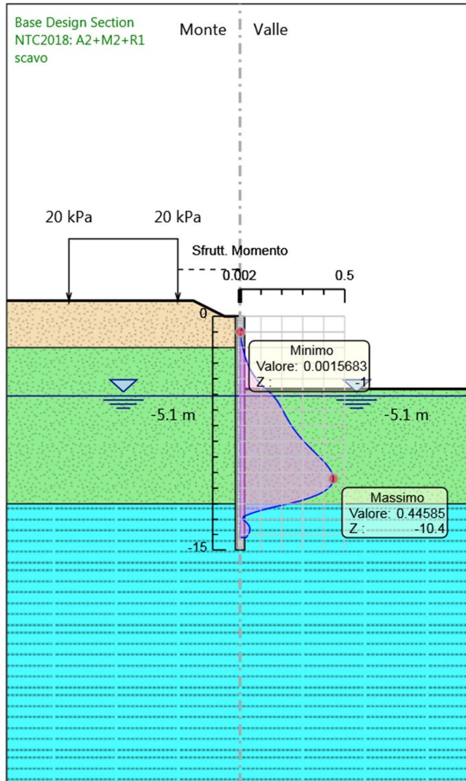
Involuppi Tasso di Sfruttamento a Momento - Cover
