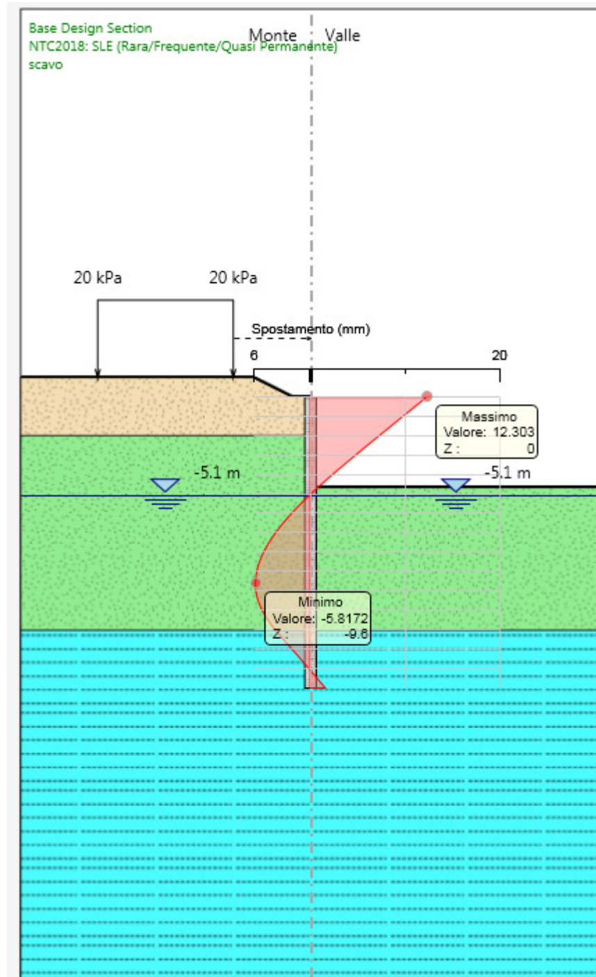
Figura 4: Modello SLE: Inviluppo degli spostamenti
