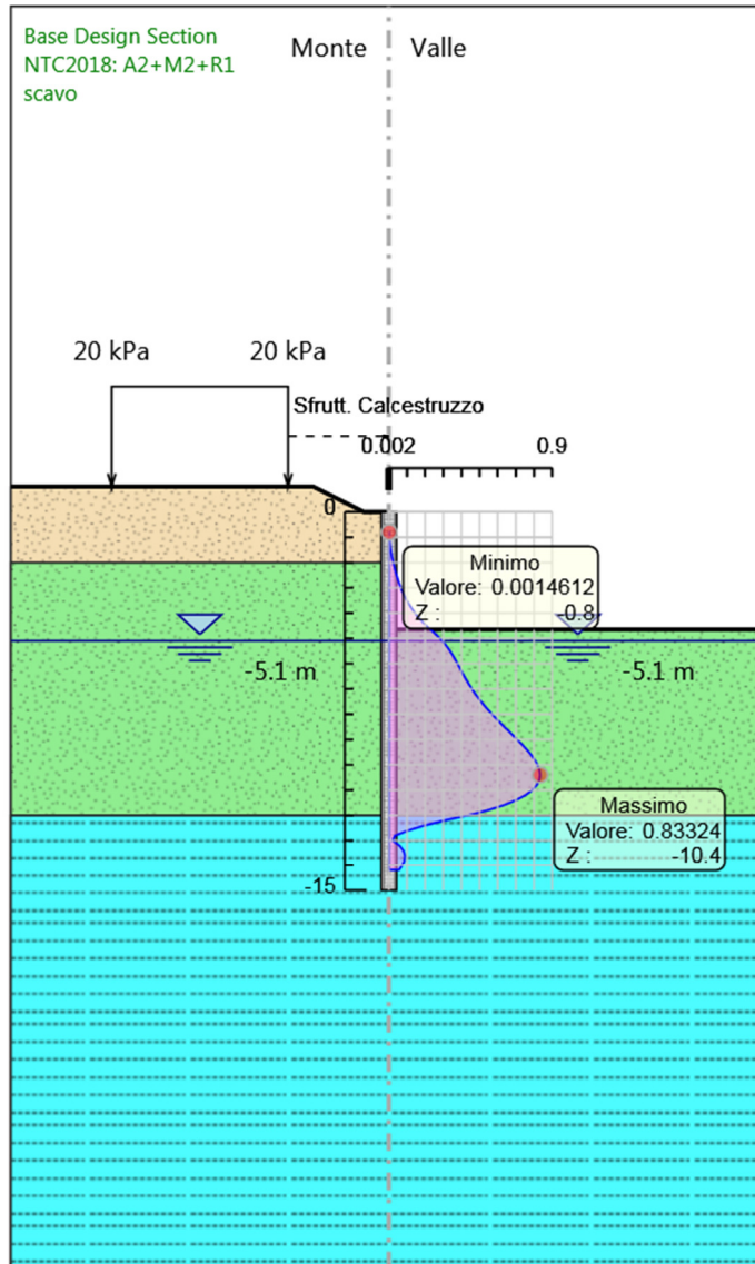
Involupi Tasso di Sfruttamento Calcestruzzo - Cover
