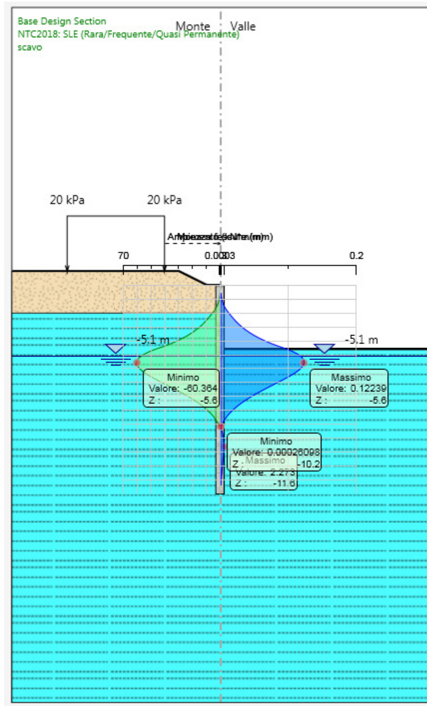
Figura 6: Modello SLE: verifica a fessurazione
