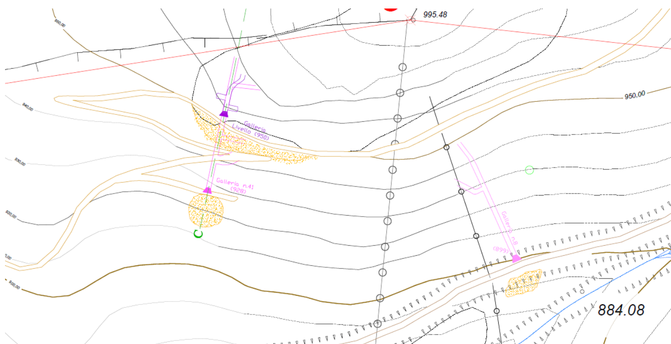
TAVOLA 4.2 – INGRANDIMENTO Planimetria PERDABILA ALTA - STATO ATTUALE
