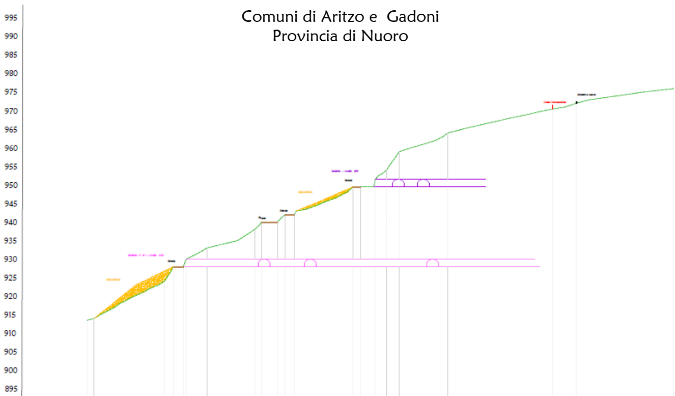
TAVOLA 4.6 – Sezione C-C PERDABILA ALTA - STATO ATTUALE
