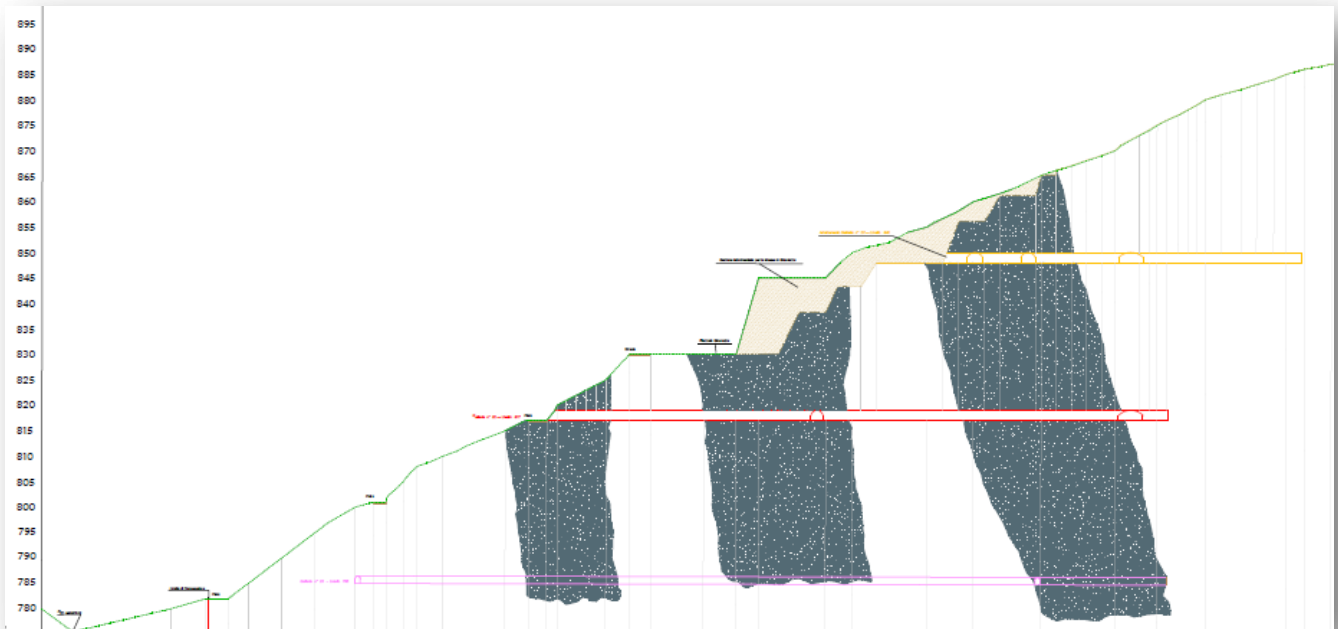
Tav. 5.1.1- MESSA IN SICUREZZA SEZIONE A-A PERDABILA
