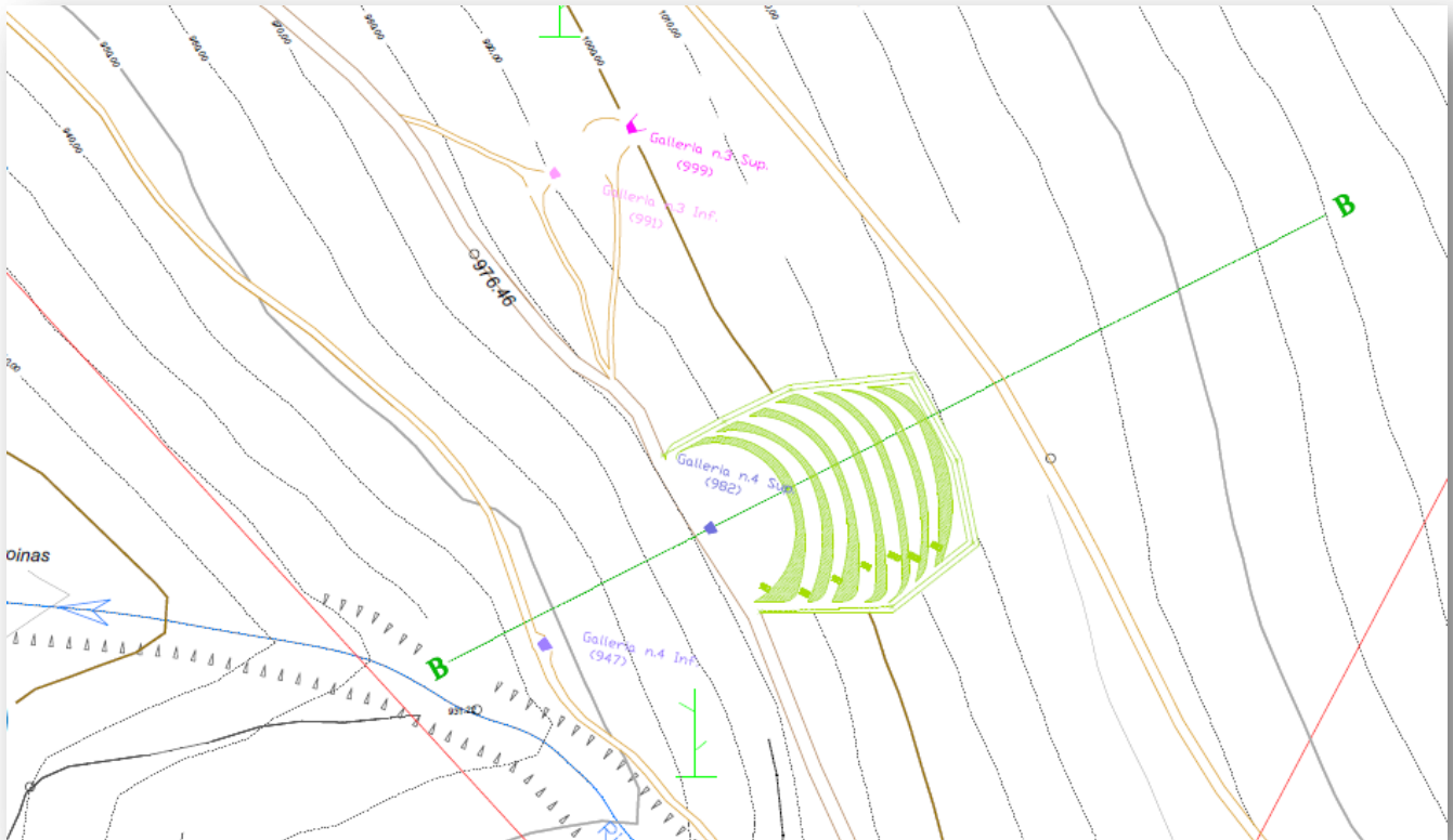
Tav. 5.2- MESSA IN SICUREZZA Planimetria MAMOINI
