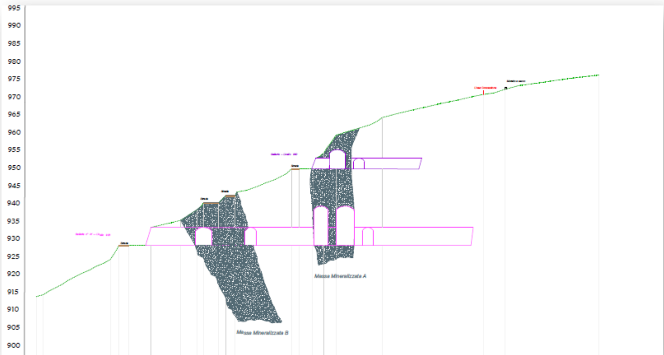
Tav. 6.3- Coltivazione Sotterraneo 5 anni SEZIONE C-C PERDABILA ALTA
