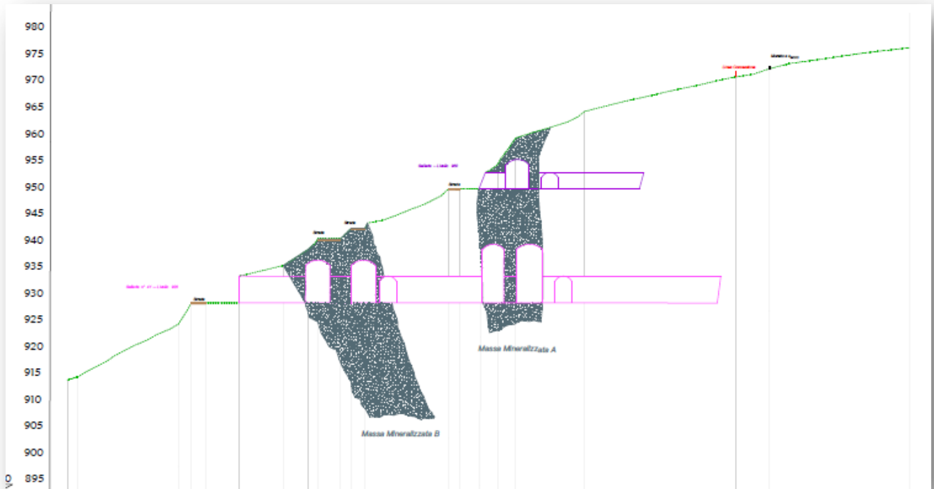
Tav. 7.3- Coltivazione Sotterraneo 10 anni SEZIONE C-C PERDABILA ALTA
