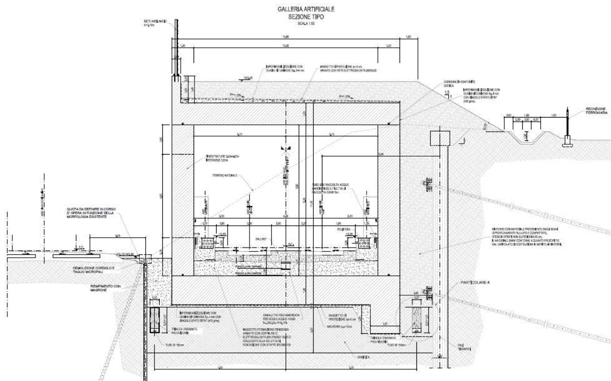
Figura 2. GA27-sezione tipo
