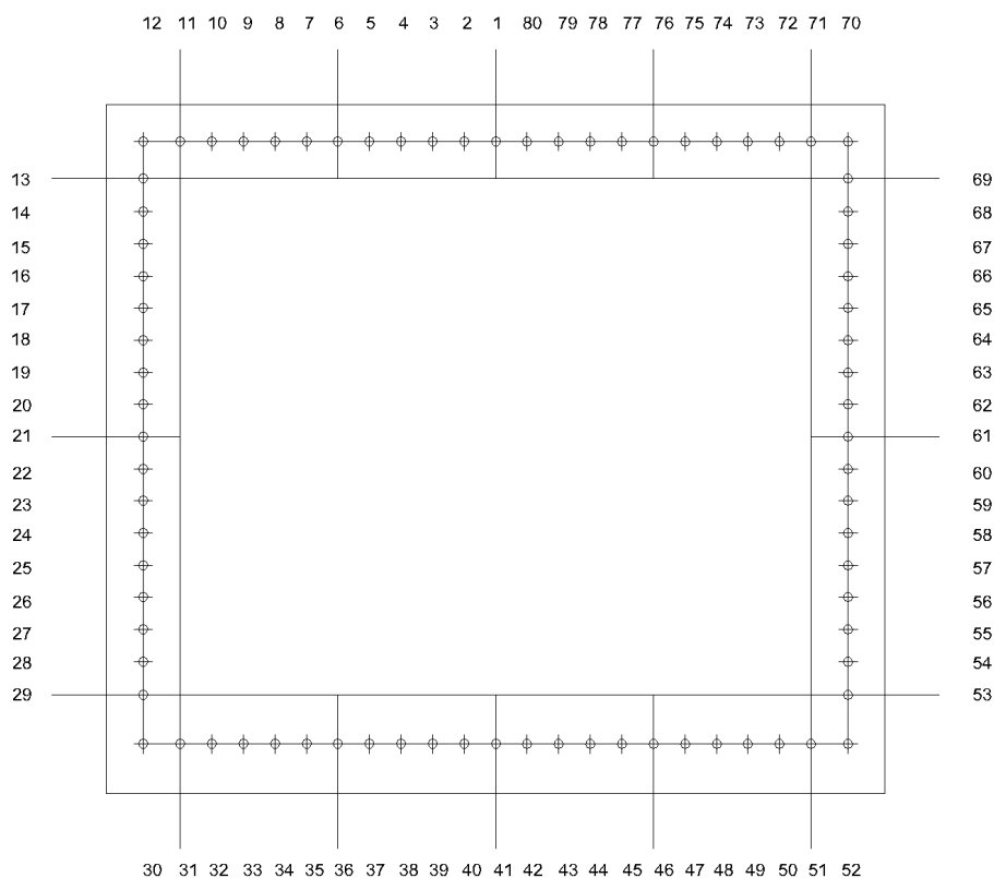
Figura 5. Numerazione dei nodi presenti nel modello– Galleria GA27.
