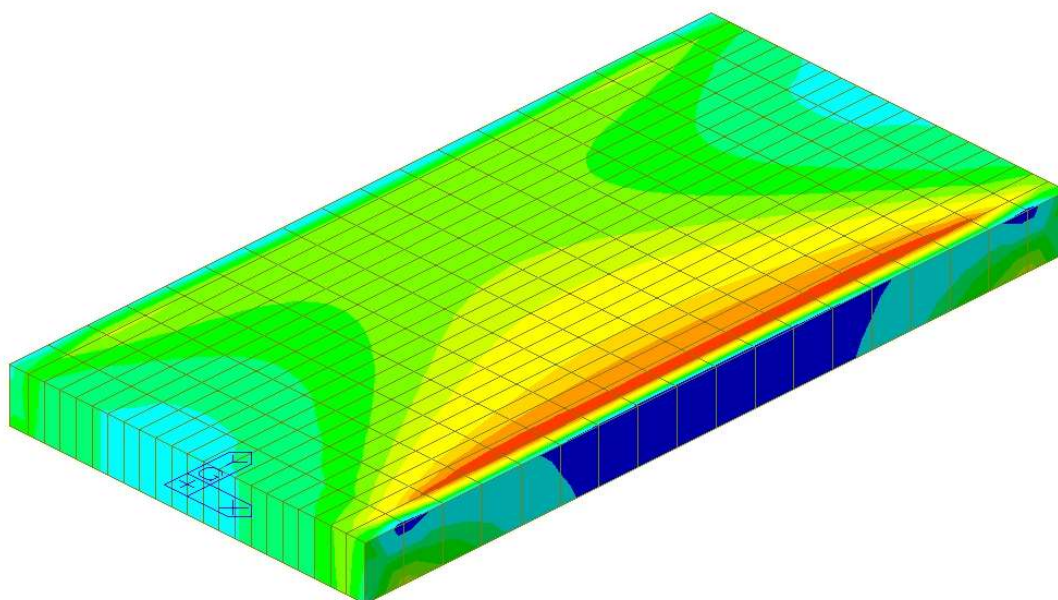
Figura 74. Tensioni in direzione longitudinale - Fondazione – Fase 2 - Galleria GA27.
