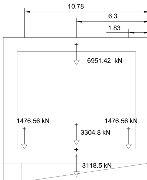
Figura 55. Peso permanente – Galleria GA27.
