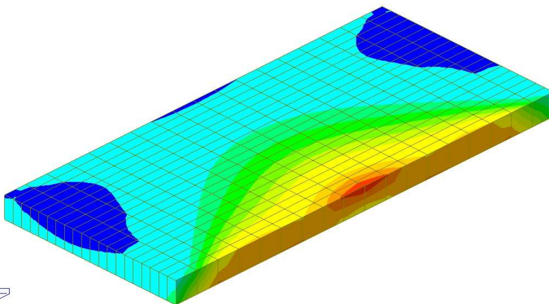
Figura 78. Tensioni in direzione longitudinale - Copertura – Fase 2 - Galleria GA27.
