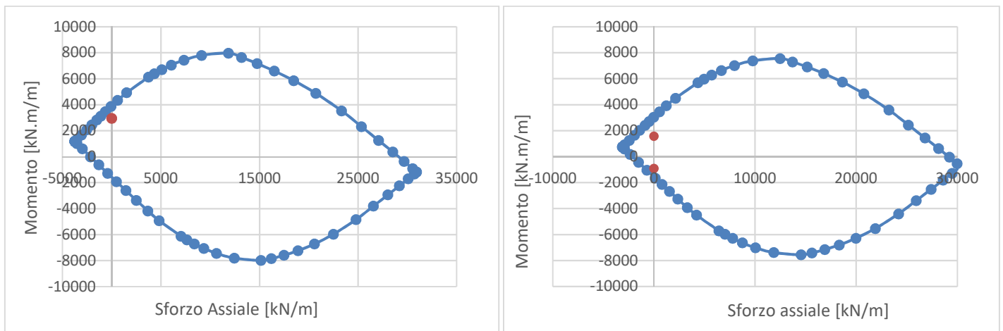
Figura 37. Dominio M, N – Sezione S7 e S8 - Galleria GA27.
