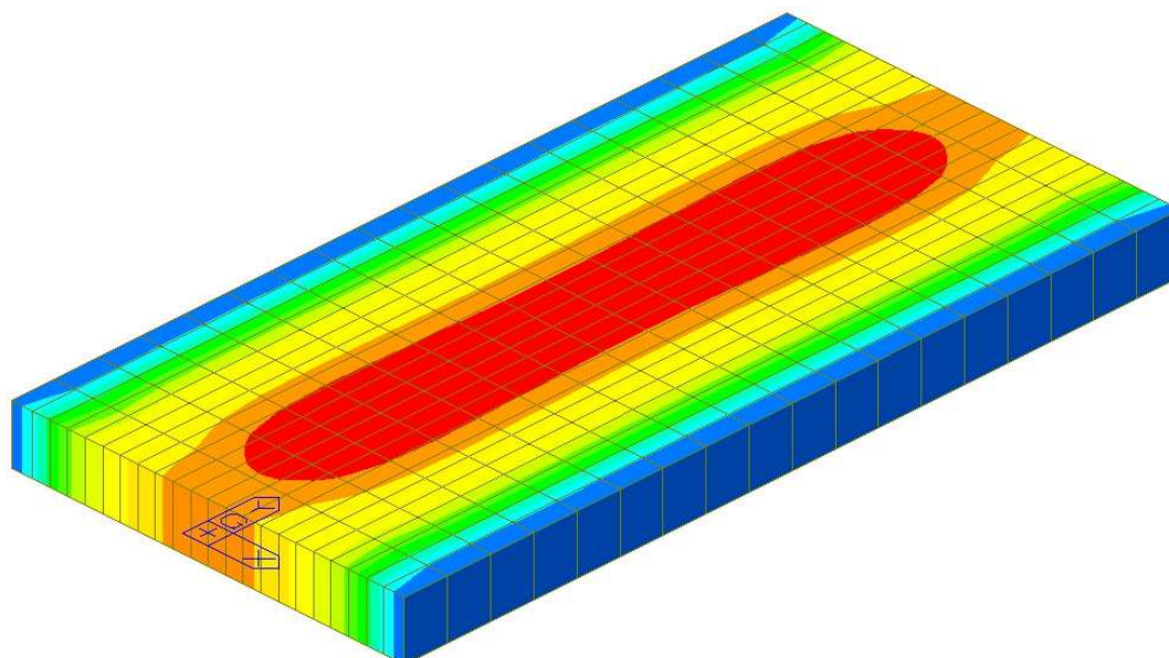
Figura 73. Tensioni in direzione trasversale – Fase 1 - Galleria GA27.
