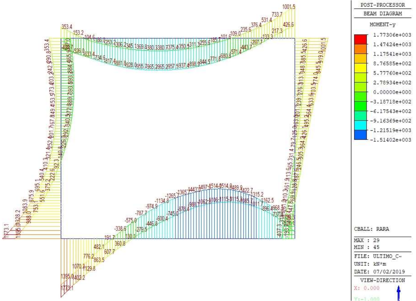
Figura 32. RARA– Involuppo delle sollecitazioni – Momento flettente -Galleria GA27.
