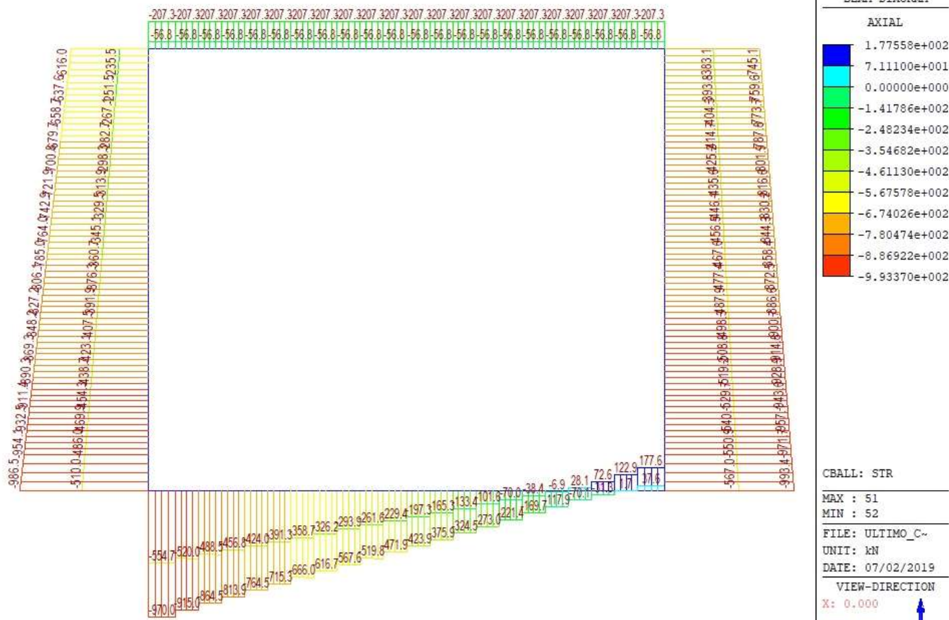
Figura 28. STR – Involuppo delle sollecitazioni – Sforzo assiale – Galleria GA27.
