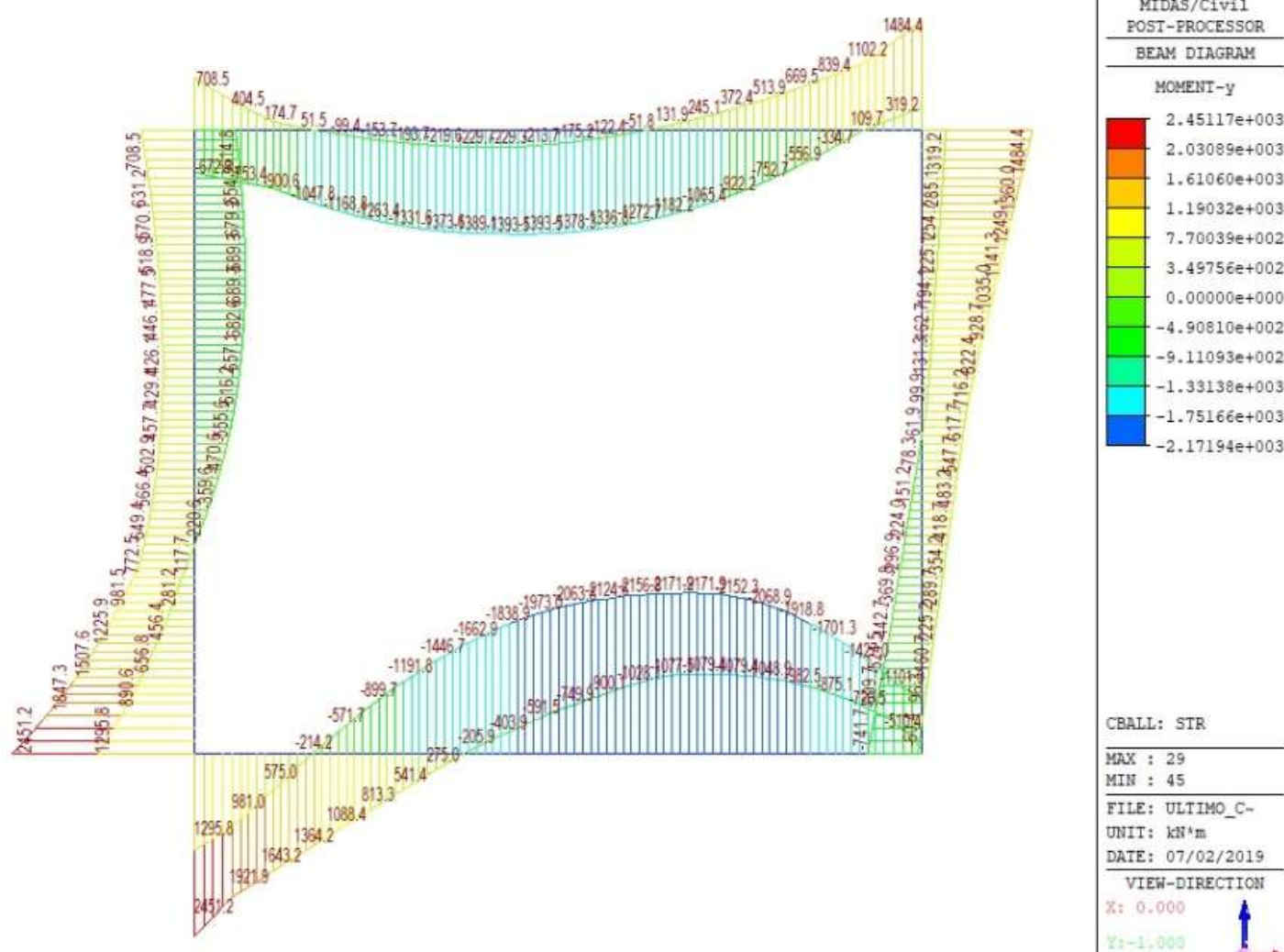
Figura 26. STR– Involuppo delle sollecitazioni – Momento flettente – Galleria GA27.
