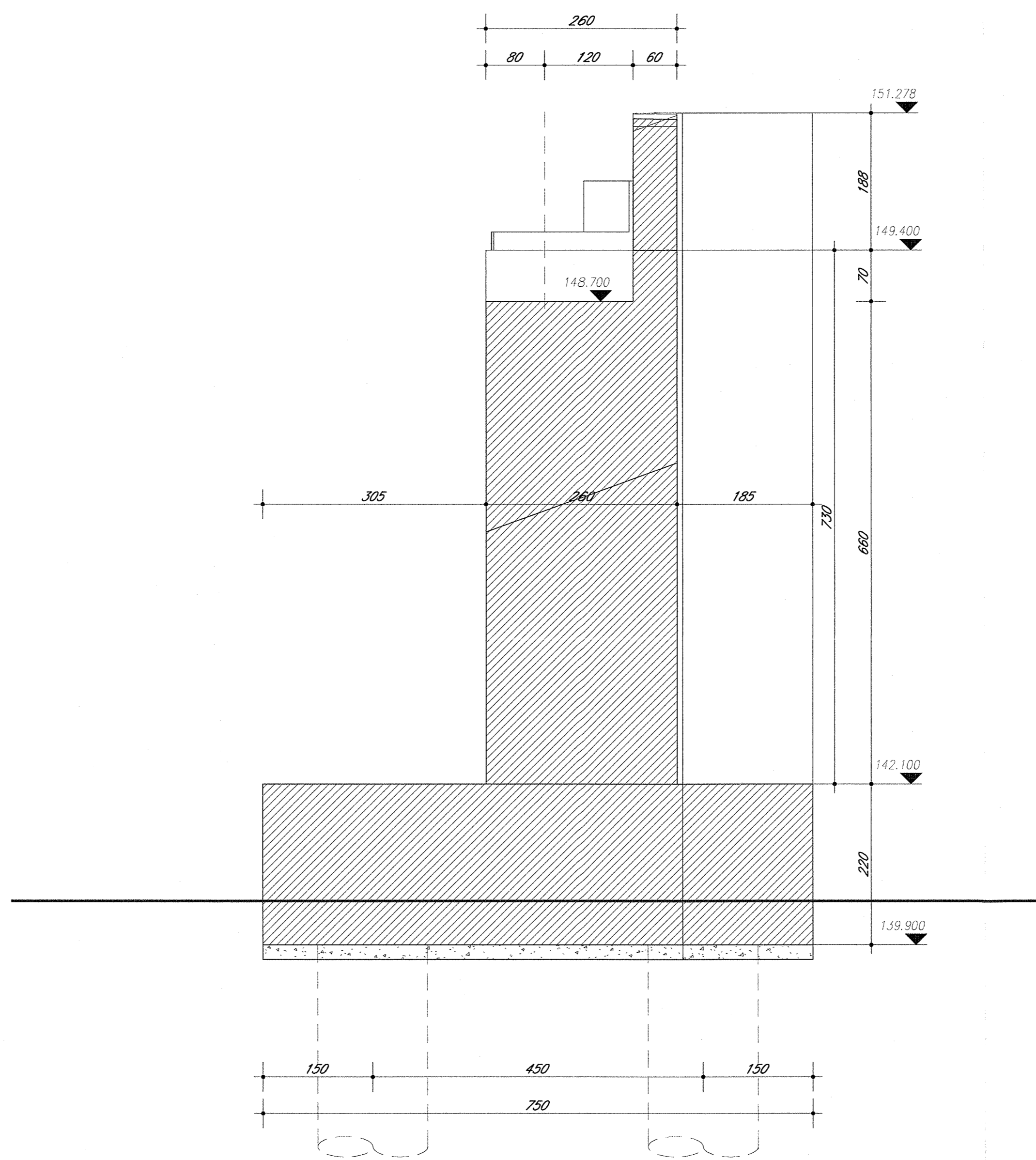
3 SpallaB - Sezione trasversale 1 : 50
