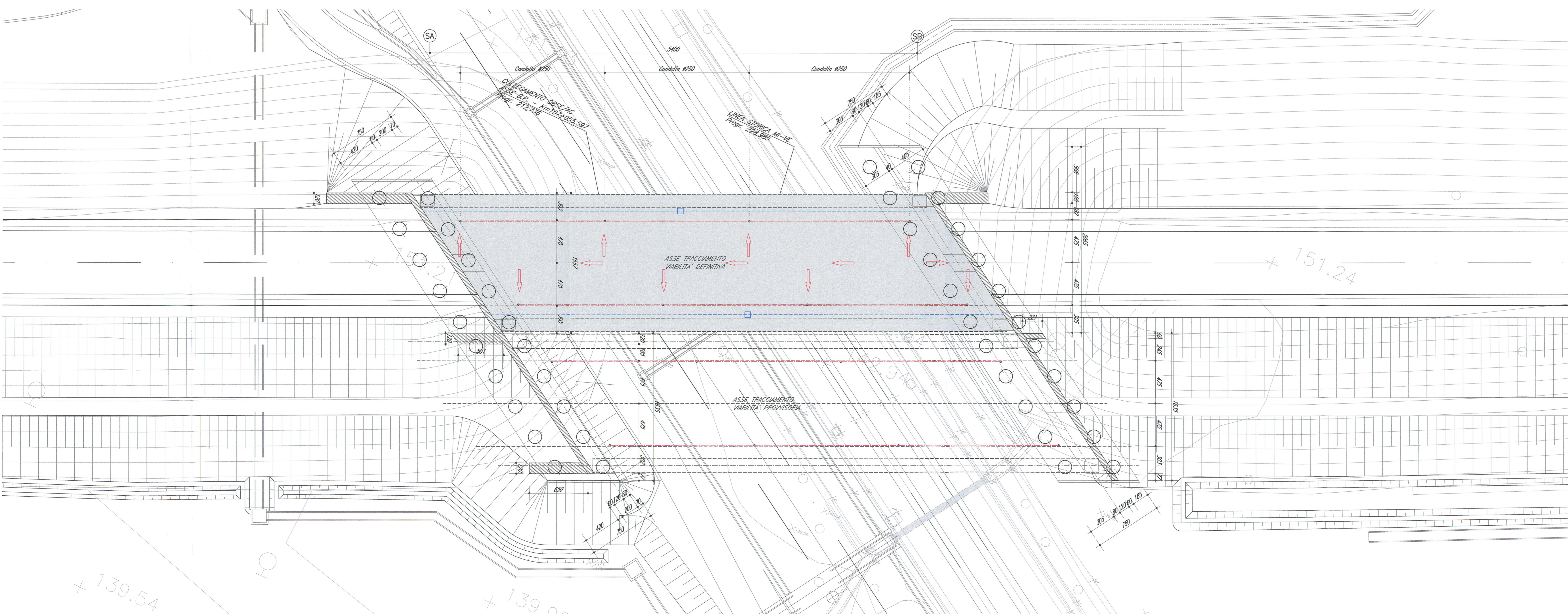
PIANTA IMPALCATO 1:200
