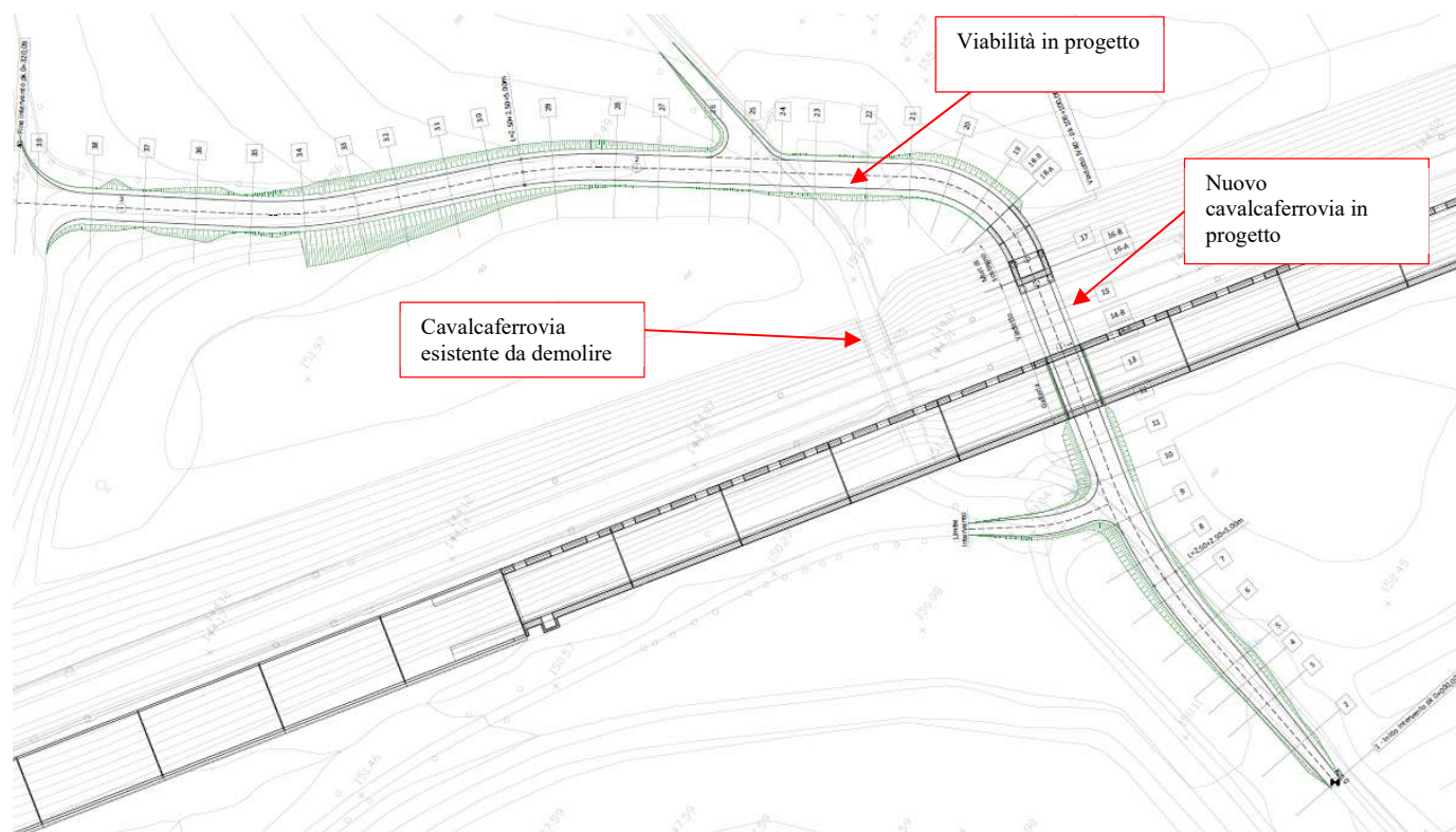
Figura 4 – planimetria
