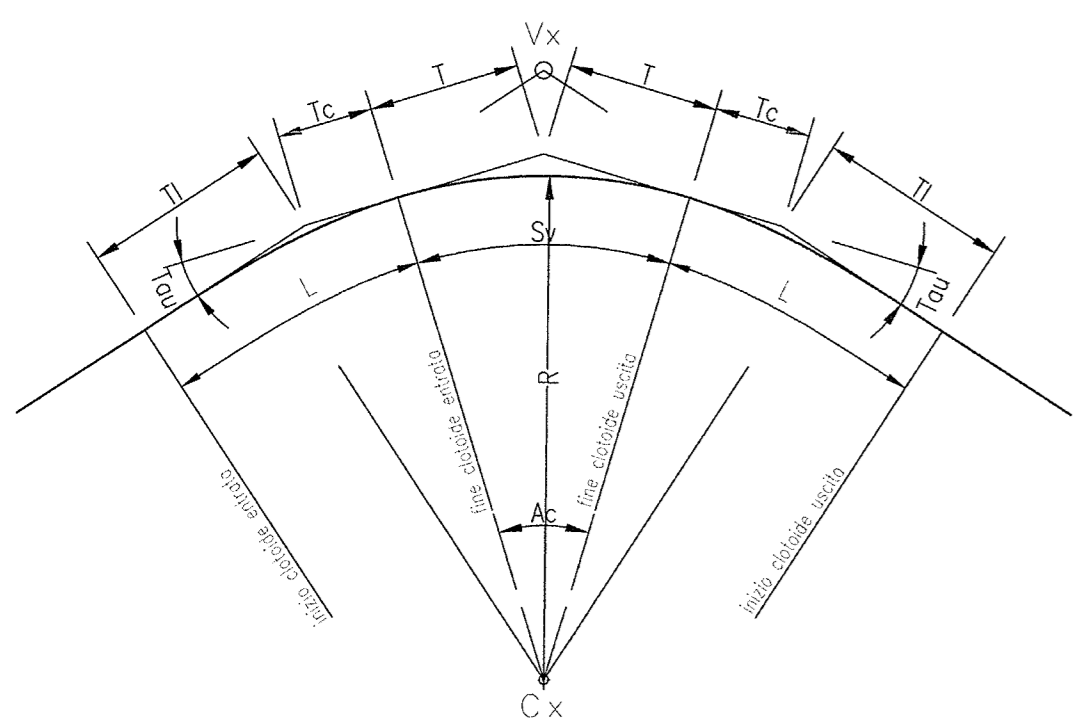
SCHEMA ESPLICATIVO TRACCIAMENTO
