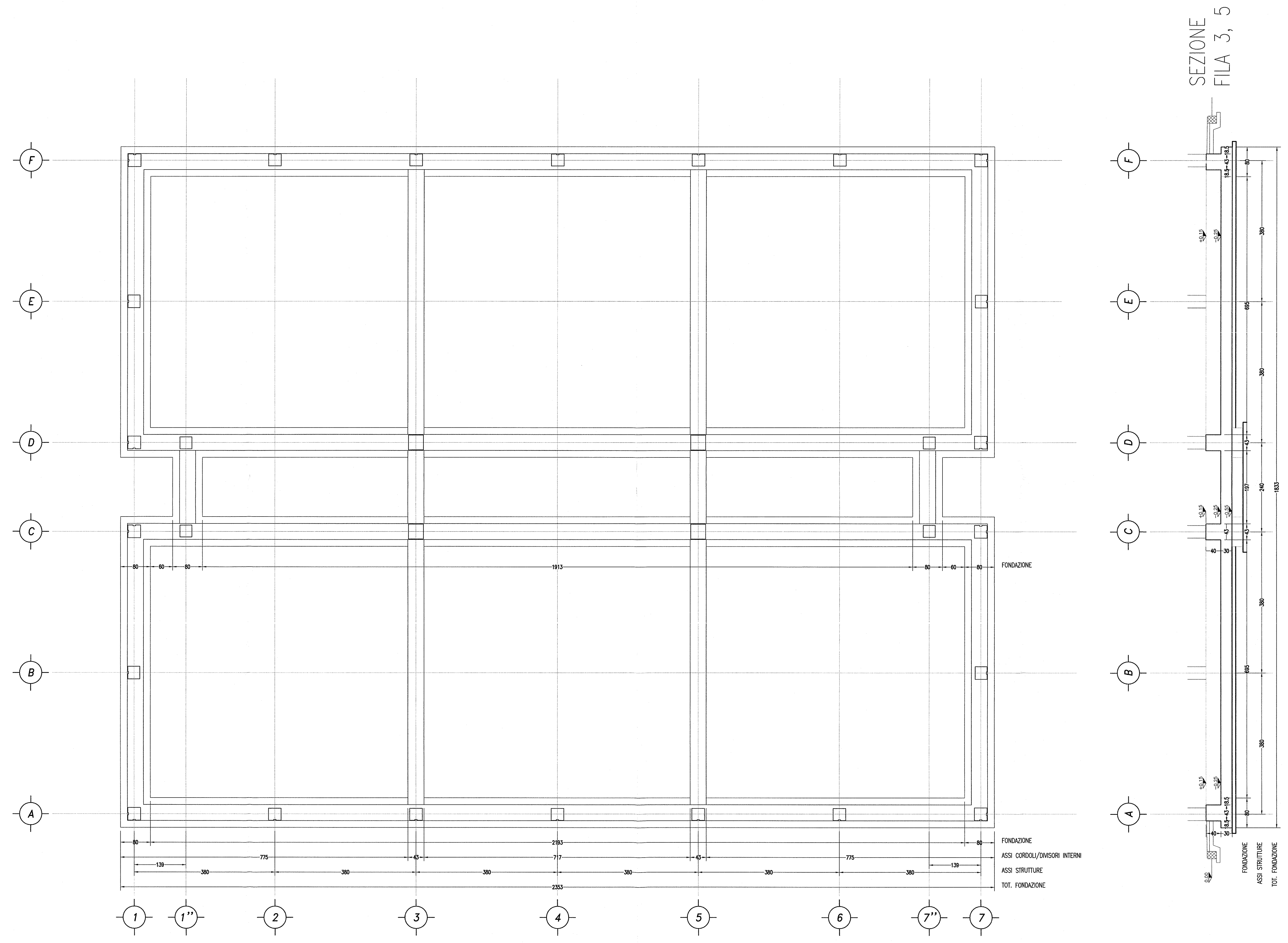
CARPENTERIA FONDAZIONI
