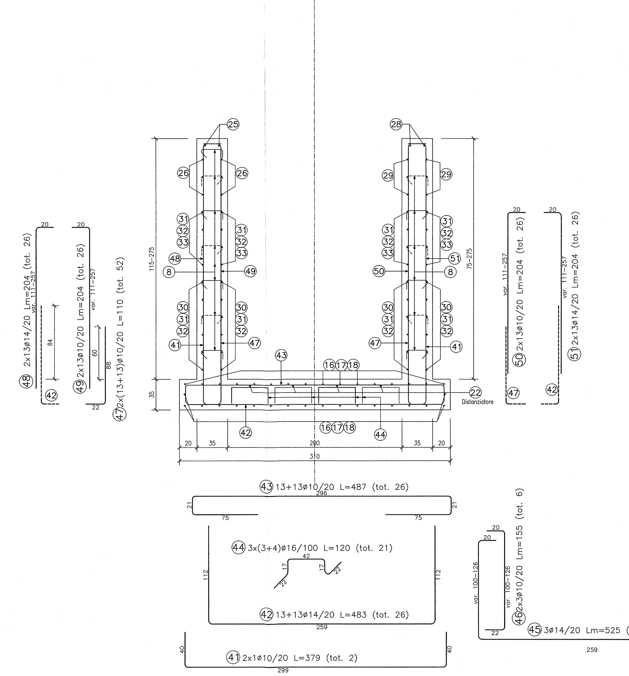
1/2 SEZIONE TRASVERSALE "B-B" scala 1:25
