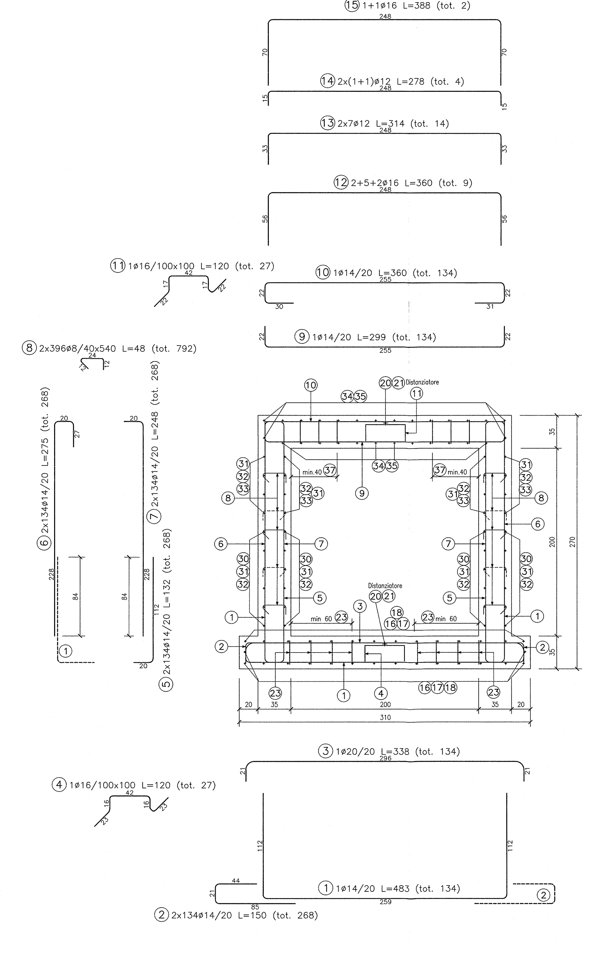
SEZIONE TRASVERSALE "A" scala 1:25
