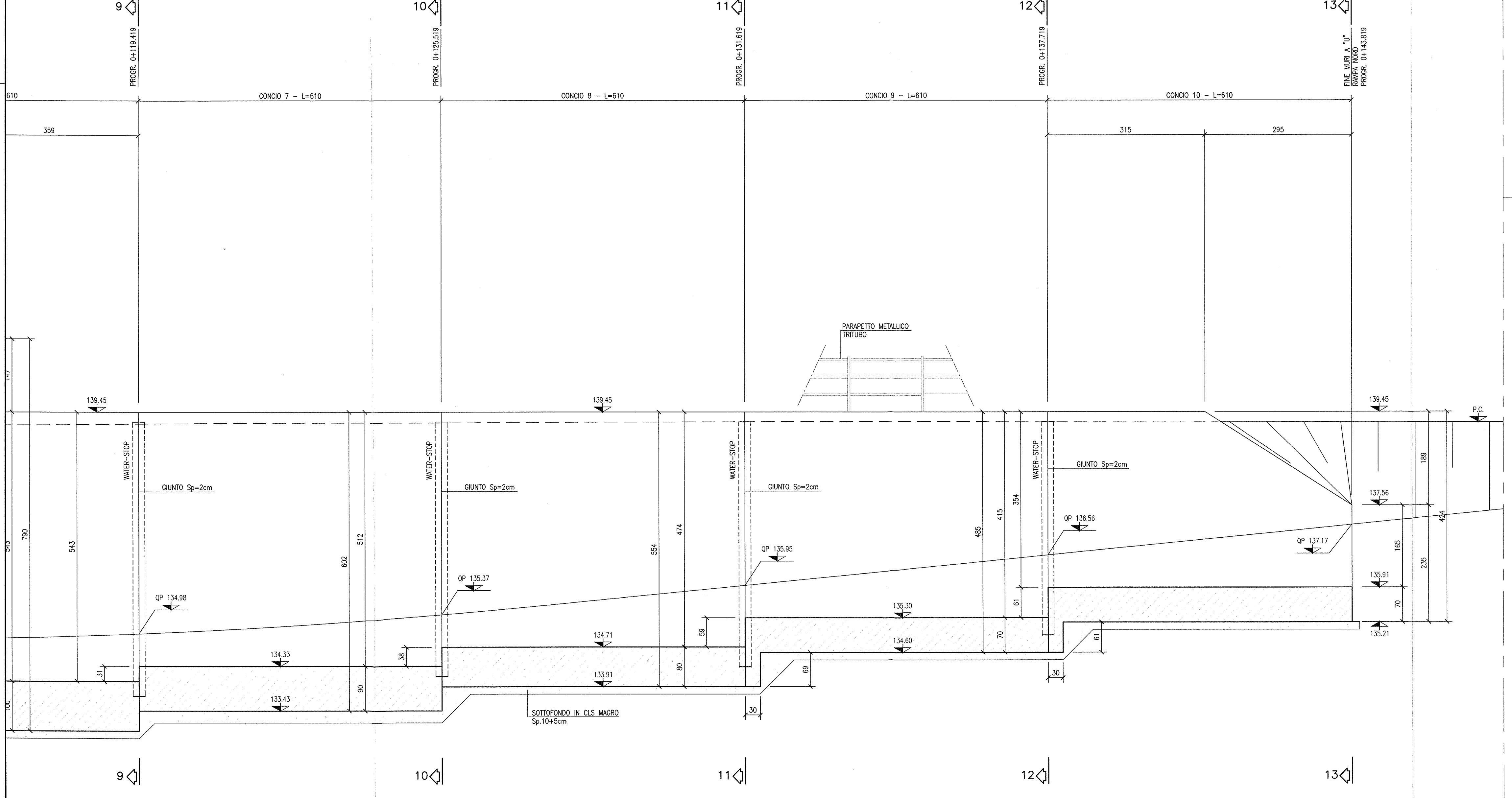
SEZIONE LONGITUDINALE IN ASSE SCALA 1:50
