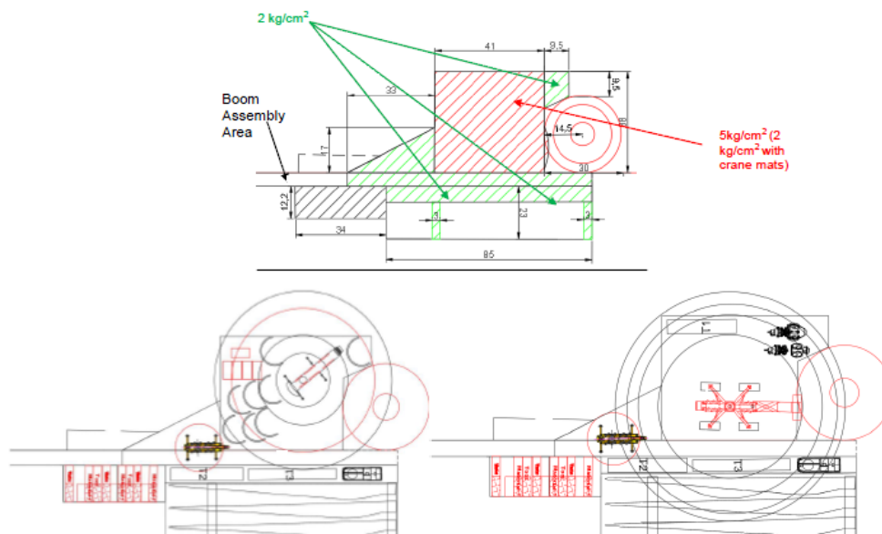
Figura 1: Schema piazzola tipologica in fase di cantiere per il montaggio dell'aerogeneratore
