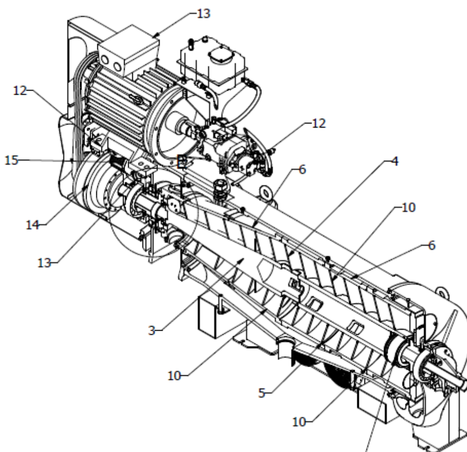
Figura 5.13: componenti interni della centrifuga
