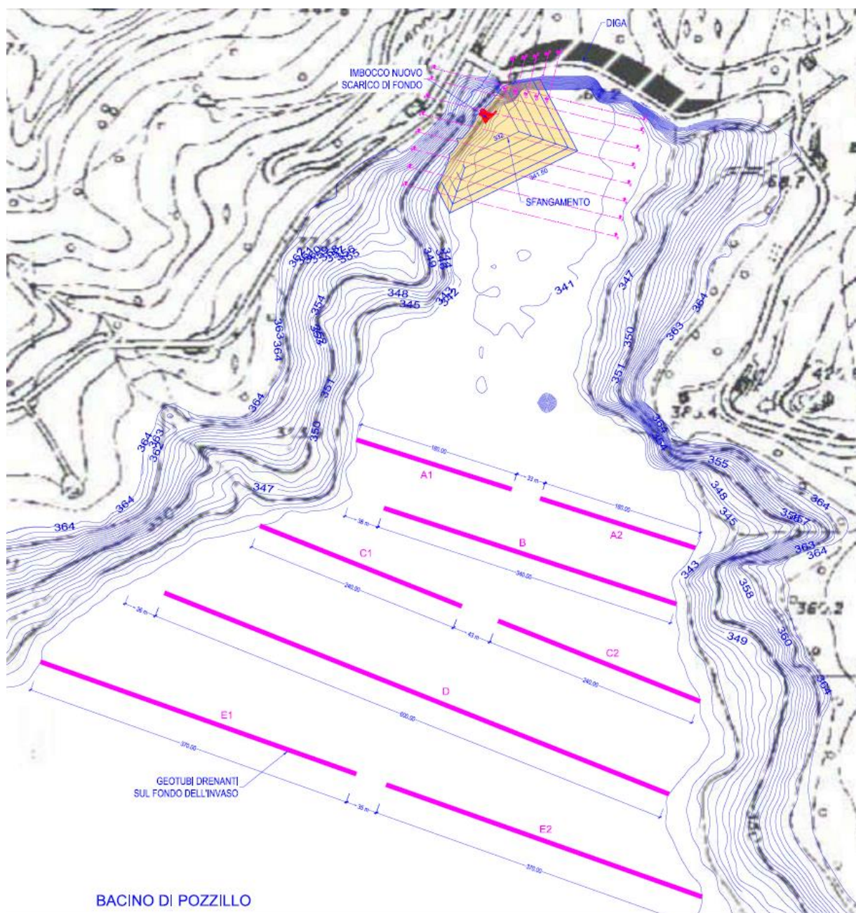
Figura 4.3: Tavola 1 - Batimetria bacino con ubicazione geotubi
