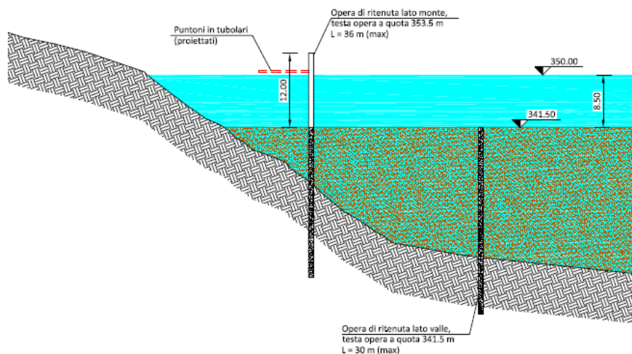
Figura 6.4: Fase 2 di realizzazione delle opere nel bacino
