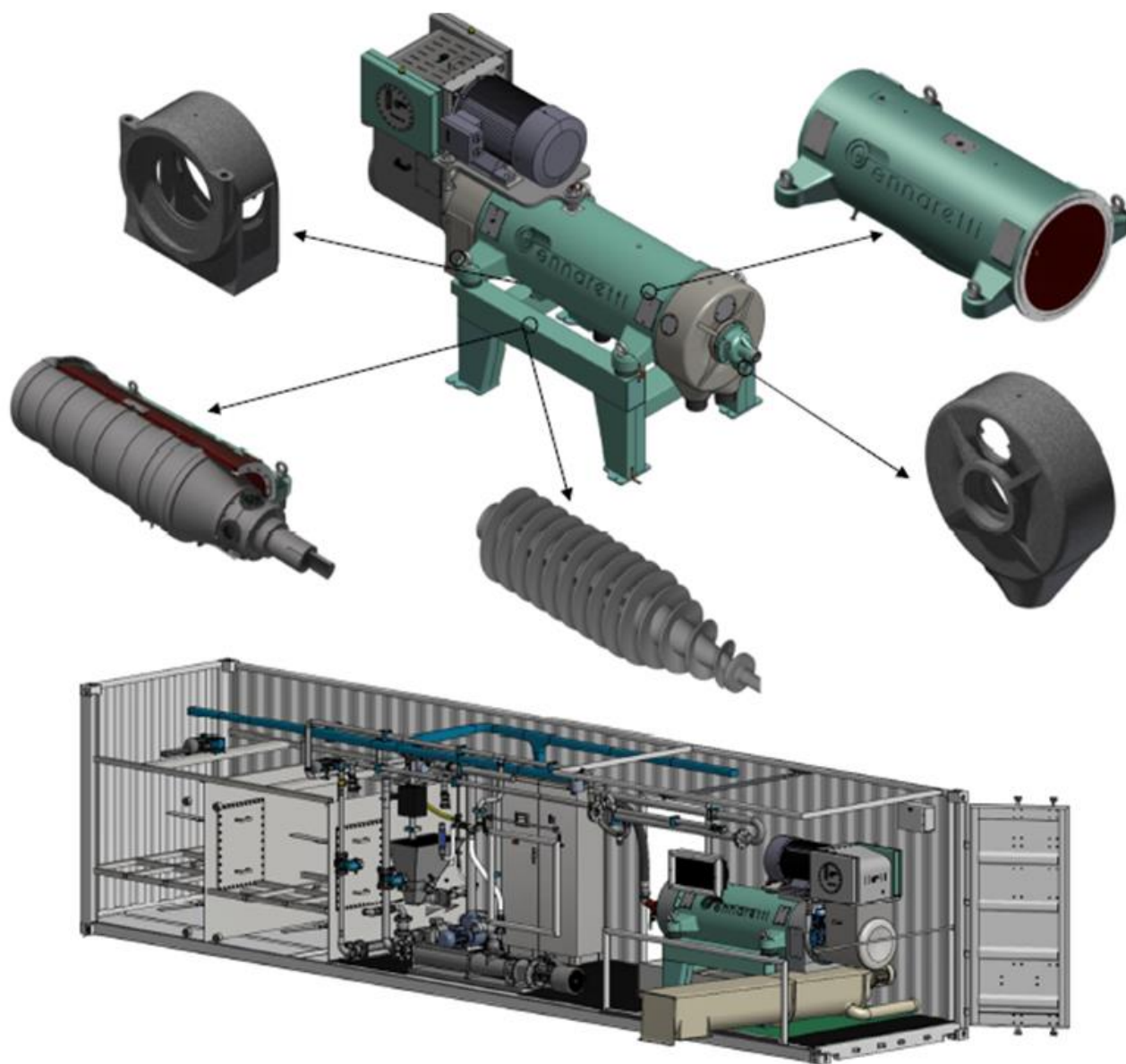
Figura 5.12: schema strutturale della centrifuga e dell'impianto di ispessimento.
