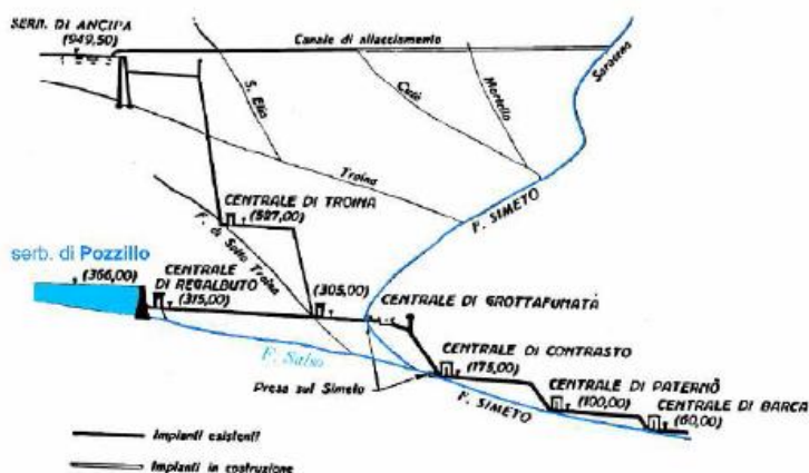
Figura 2.1: Ubicazione della diga e schema degli impianti
