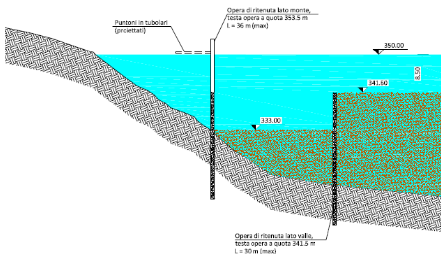
Figura 6.5: Fase 3 di realizzazione delle opere nel bacino
