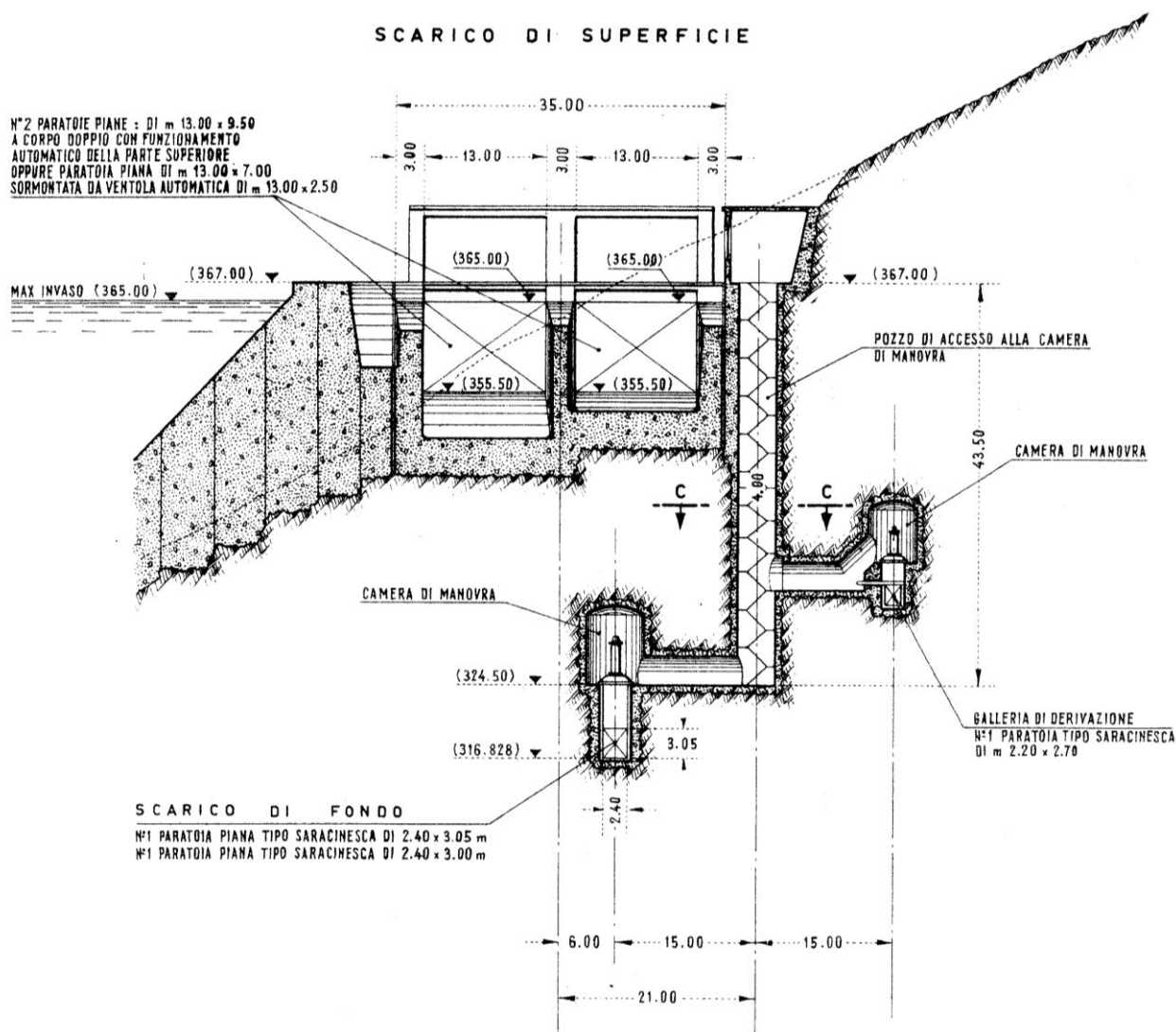
Figura 3.3: Prospetto dello scarico di superficie dal progetto originale della diga
