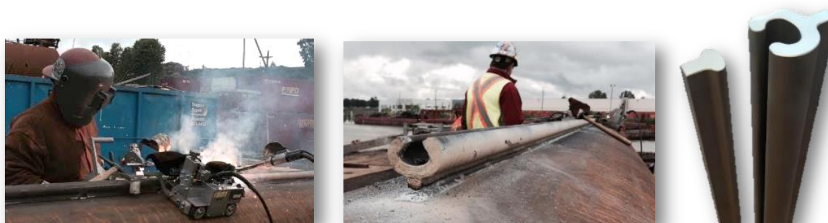
Figura 5.5: Gargame ad omega durante la fase di saldatura lungo il fusto del lamierino.
