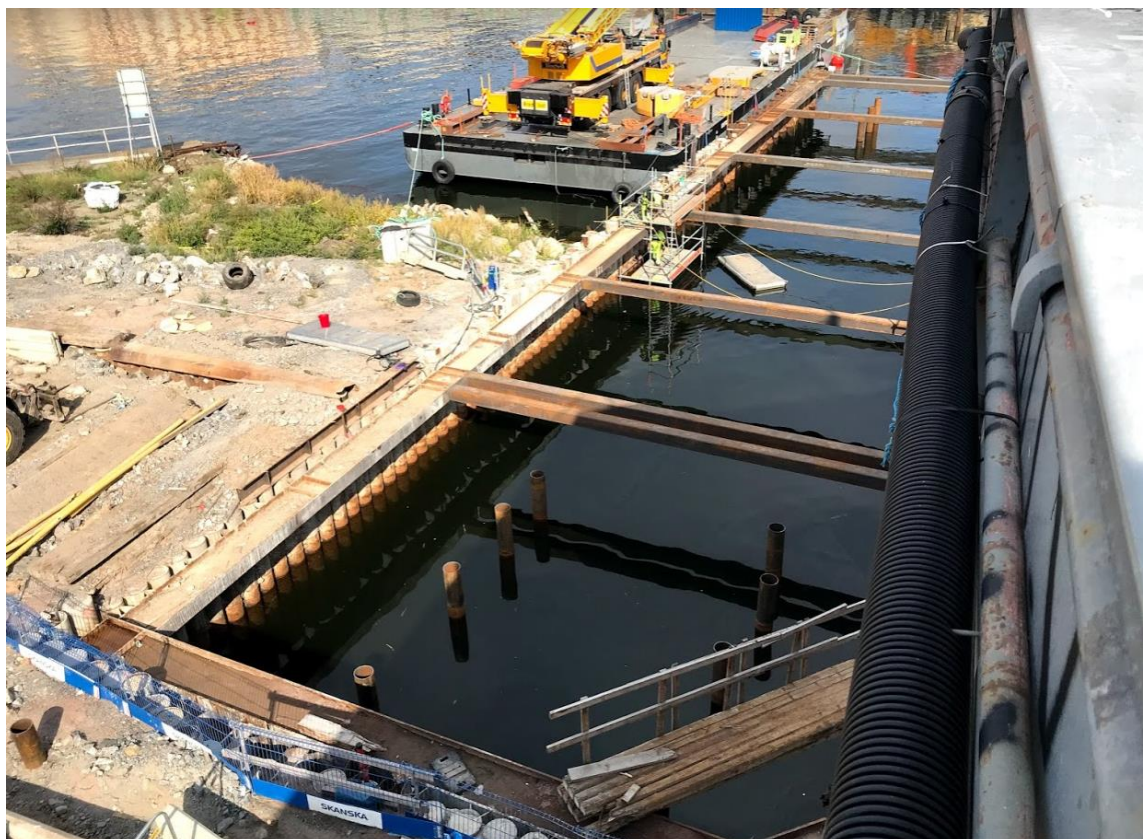
Figura 5.10: Impianto cantiere durante la realizzazione delle paratie nella laguna di Stoccolma per la realizzazione di una nuova chiusa.
