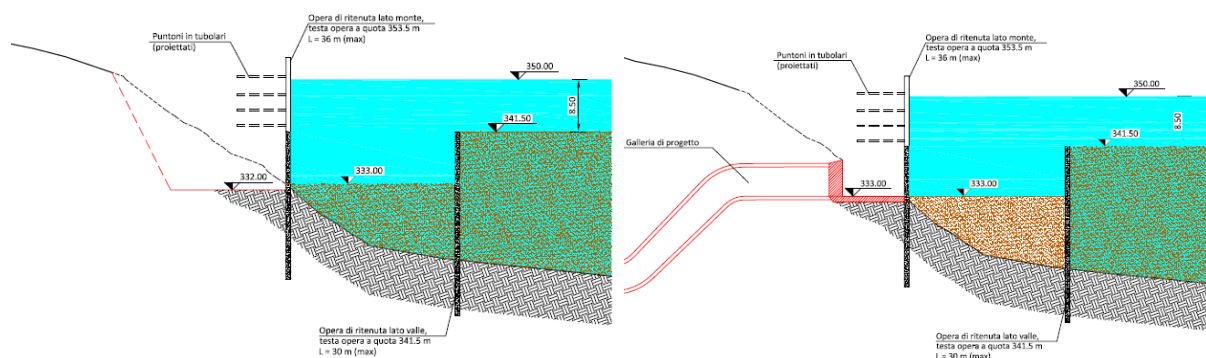
Figura 6.7: Fasi 11-12 di realizzazione delle opere nel bacino
