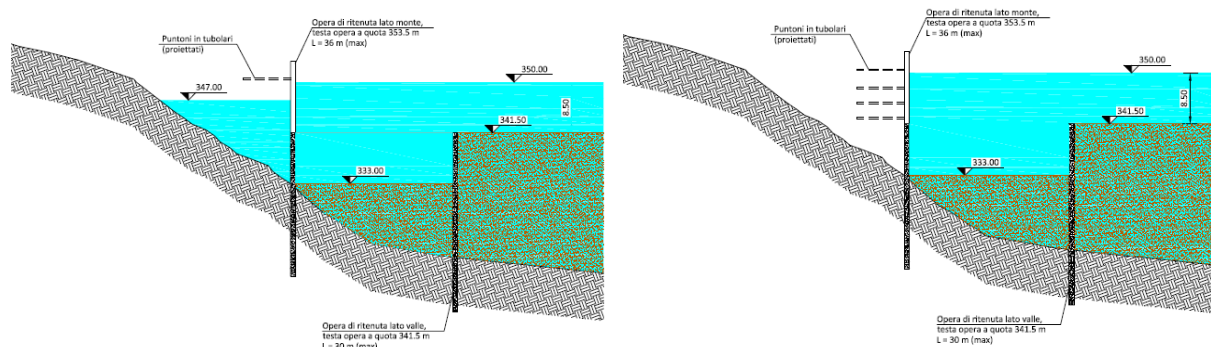
Figura 6.6: Fasi 4-10 di realizzazione delle opere nel bacino
