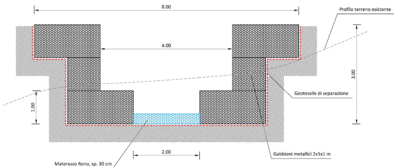
Figura 6.12: sezione d'alveo a valle della briglia.
