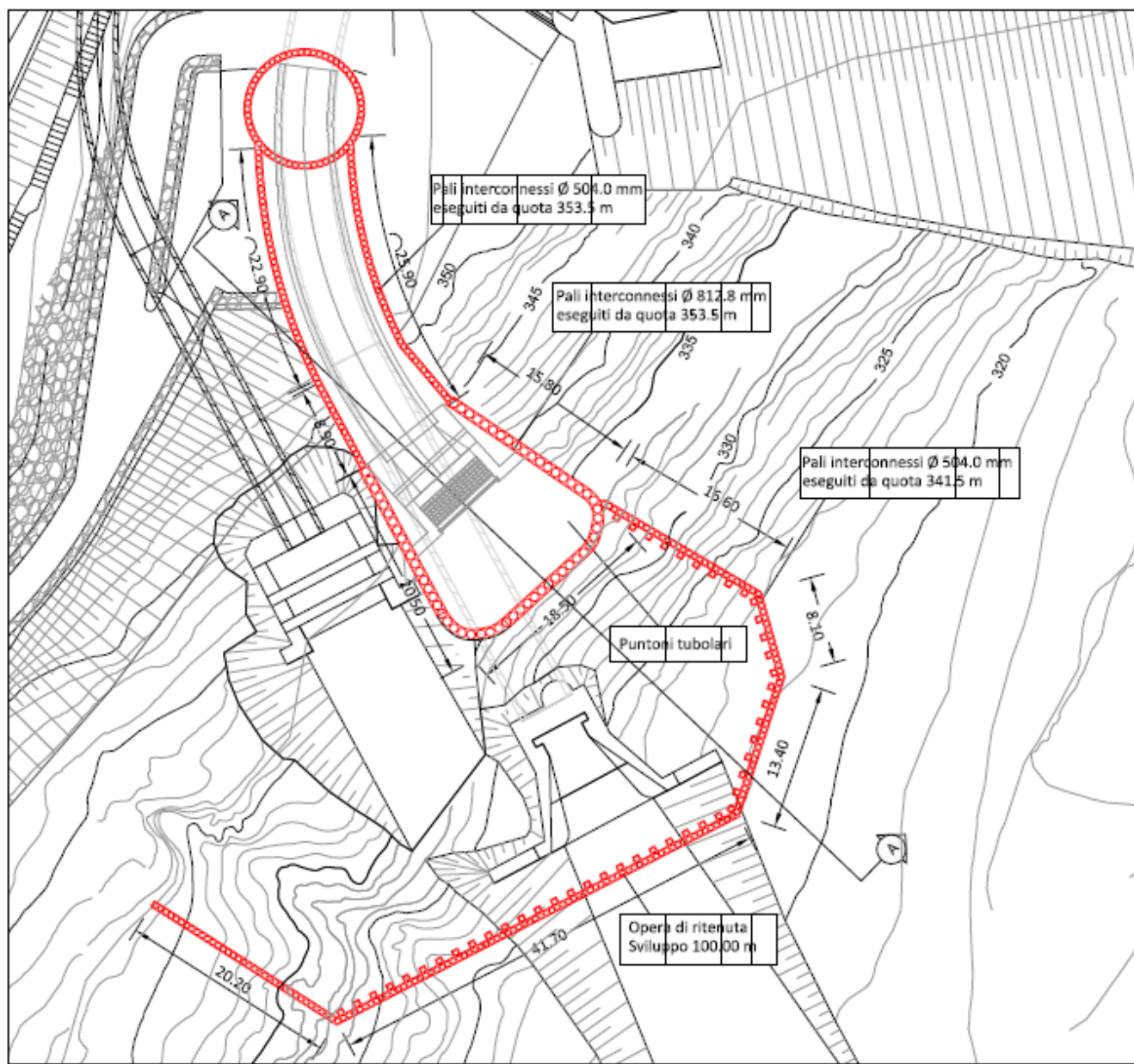
Figura 6.1: Planimetria opere provvisorie
