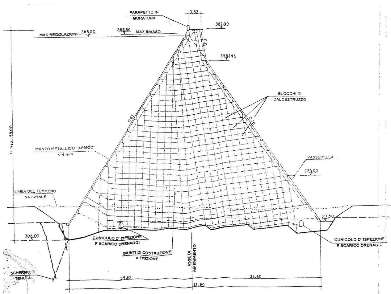
Figura 3.2: Sezione trasversale tipo della diga
