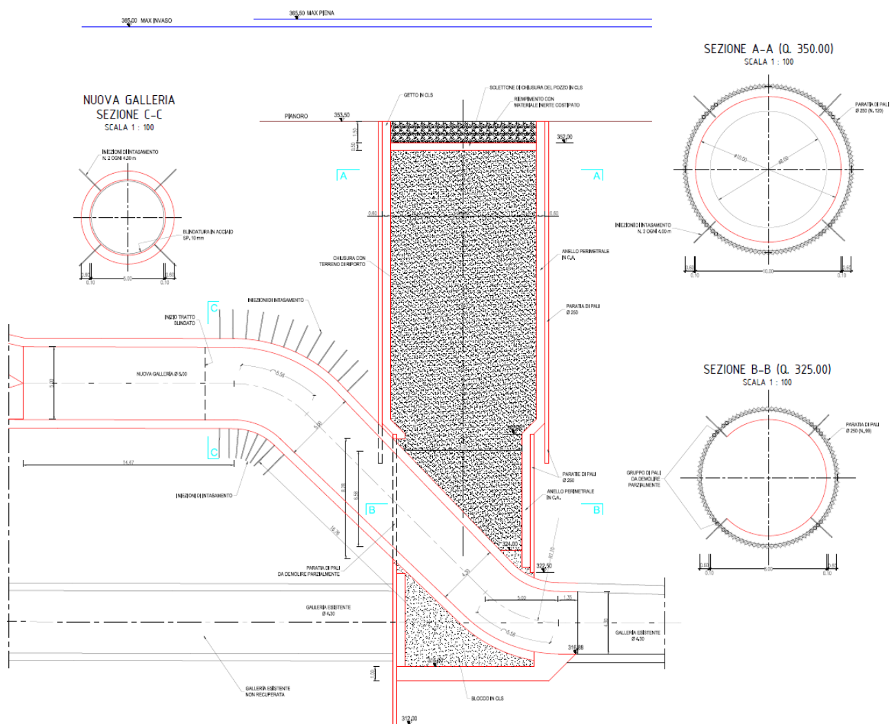
Figura 4.1: Tavola 5 - Sezioni particolari pozzo e galleria
