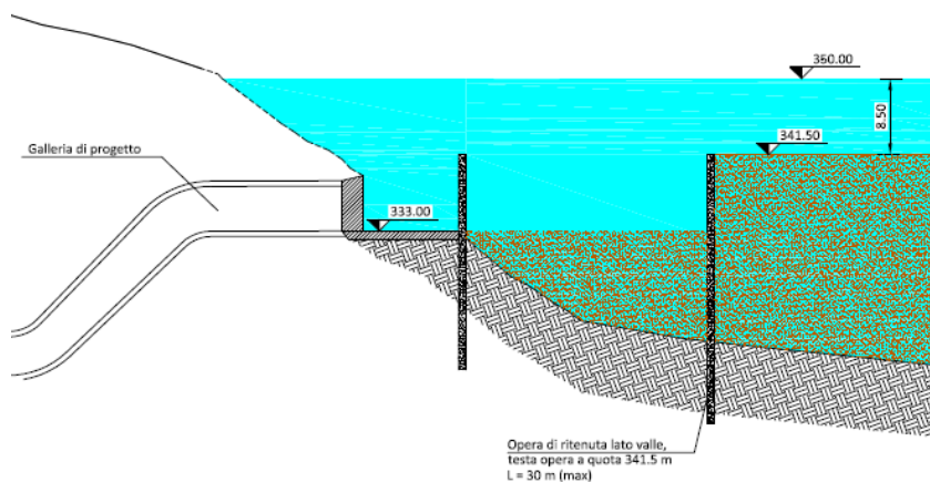
Figura 6.9: Fase 14 di realizzazione delle opere nel bacino
