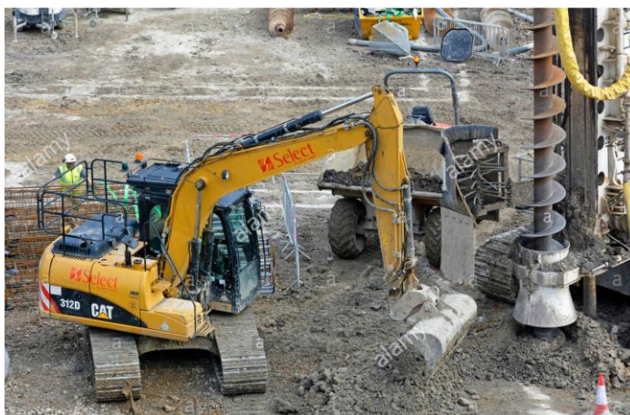
Figura 5.1: tecniche di scavo tradizionali, a sinistra il cucchiaio a destra l'elica continua.
