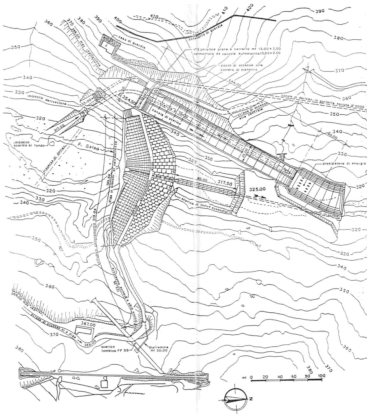
Figura 3.1: Planimetria della diga
