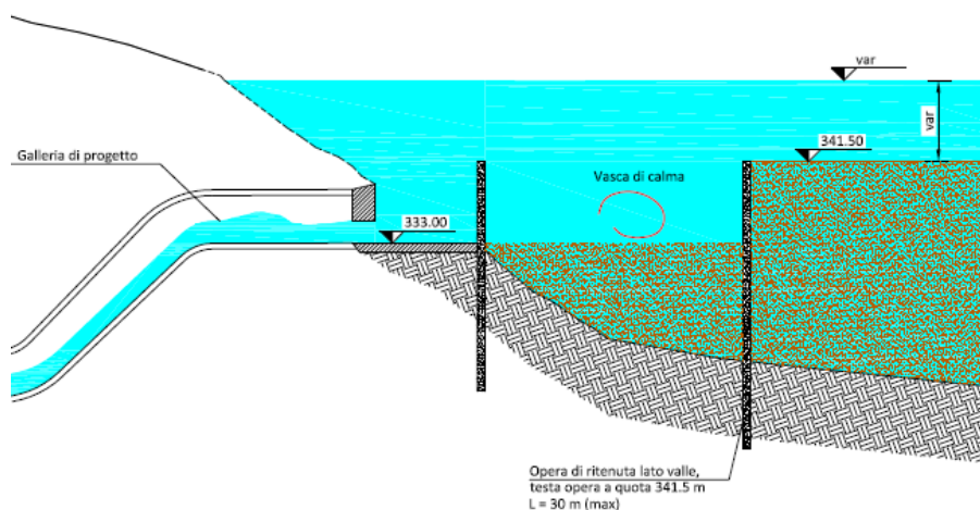
Figura 6.10: Fase 15 di realizzazione delle opere nel bacino
