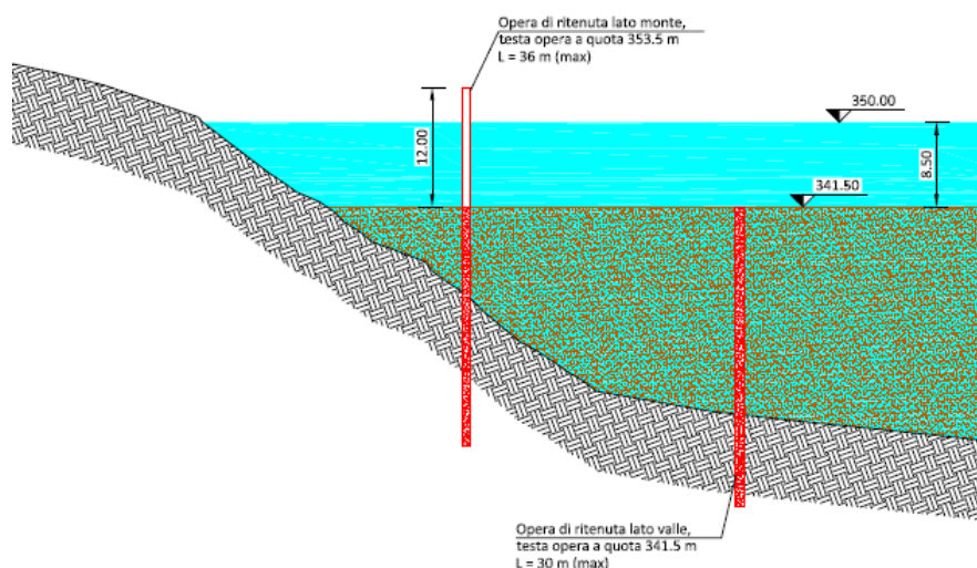
Figura 6.3: Fase 1 di realizzazione delle opere nel bacino
