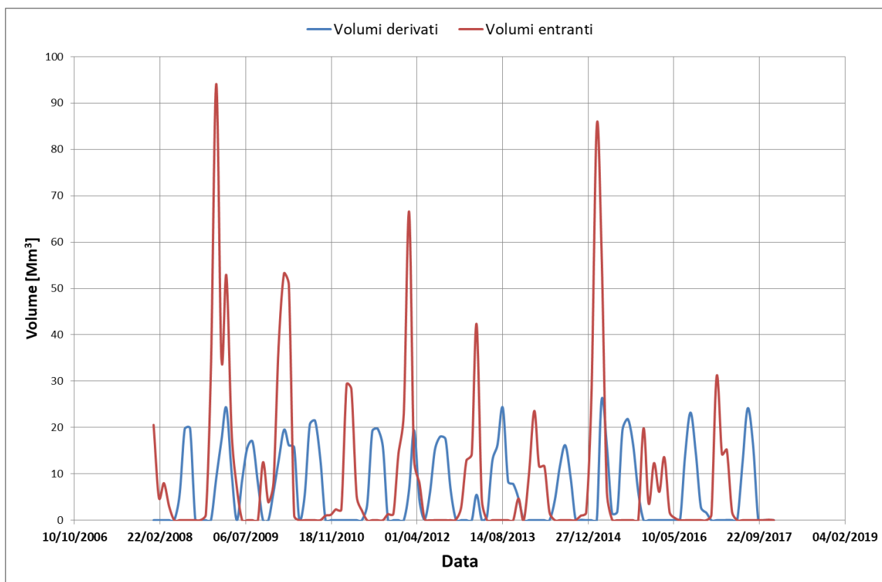
Figura 7.1: Andamento dei volumi entranti e derivati mensilmente dall'invaso (dal 2006 ad oggi)
