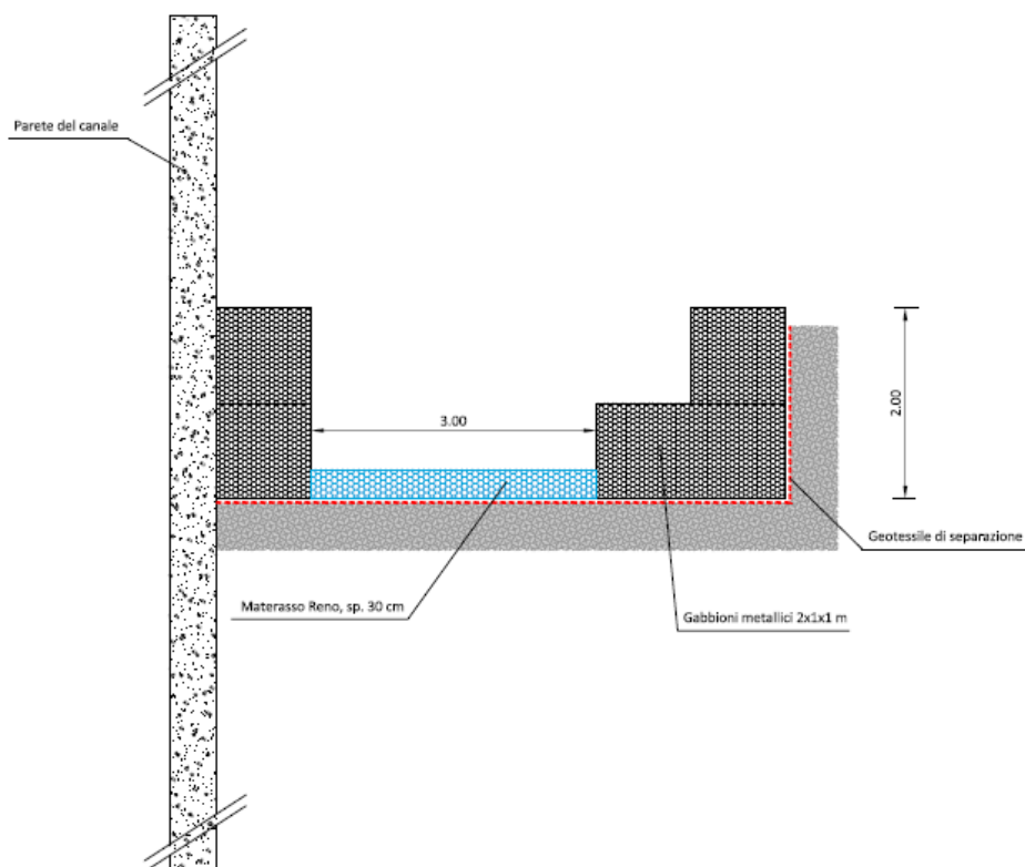
Figura 6.13: sezione d'alveo parallela al muro.
