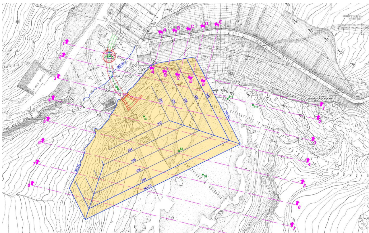
Figura 4.2: Tavola 2 - Planimetria Area Dragaggio
