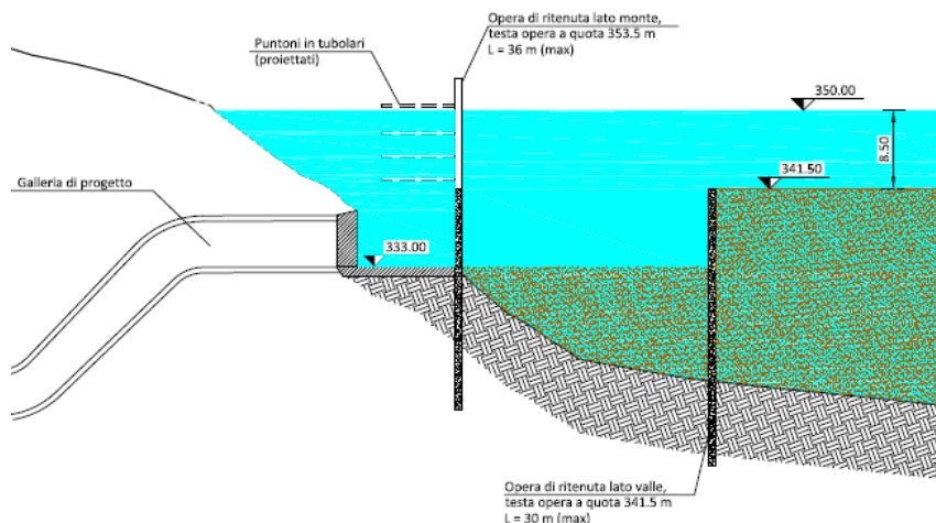
Figura 6.8: Fase 13 di realizzazione delle opere nel bacino
