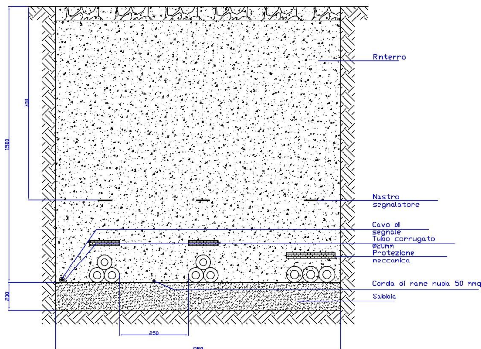
Sezione cavidotto MT
