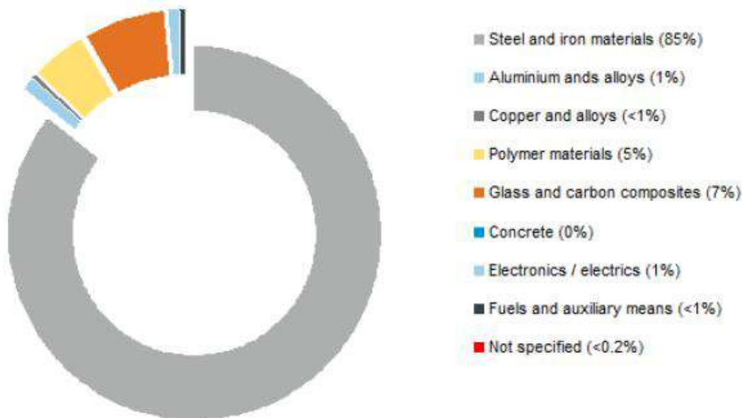
Figura 1: % in massa dei materiali che compongono l'aerogeneratore Vestas V117 3,45 MW-HH 91,5m Sulla base del sopraccitato studio, si elencano di seguito i materiali e componenti in funzione della modalità di gestione prevista.
