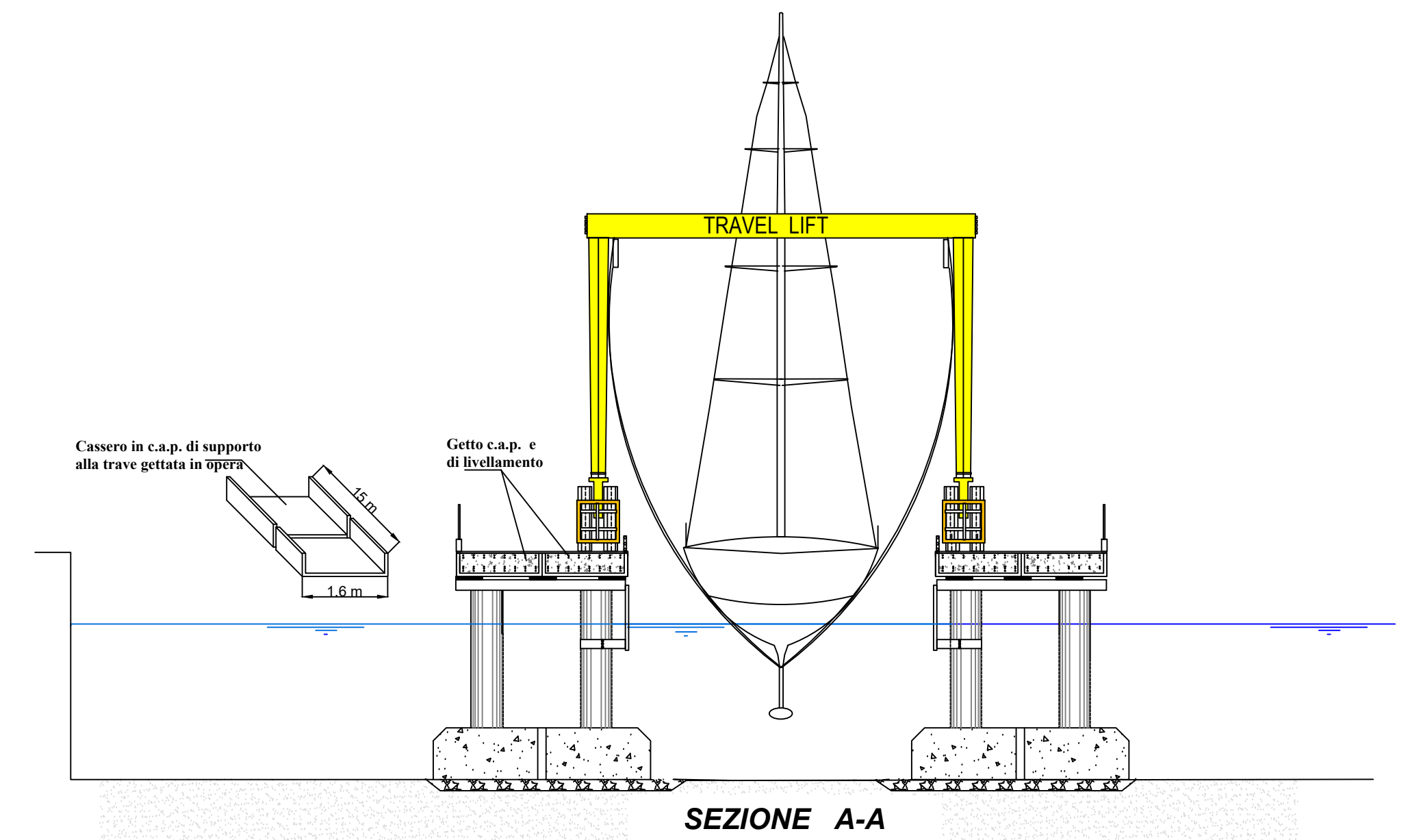
Schema con impiego di scatolari prefabbricati a SCALA 1:100
