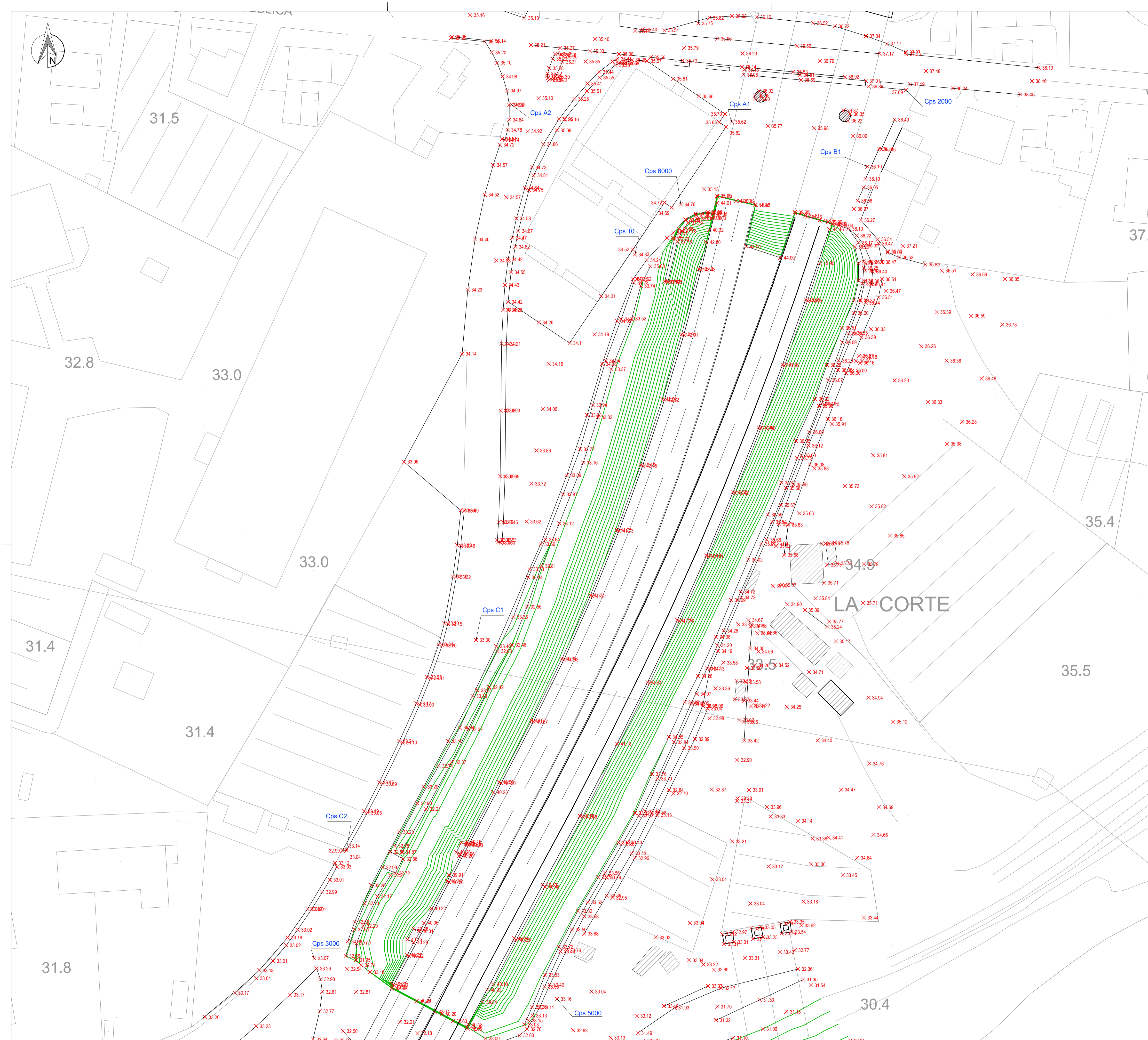
PLANIMETRIA DI RILIEVO - Inquadramento estremità Sud SCALA 1:500
