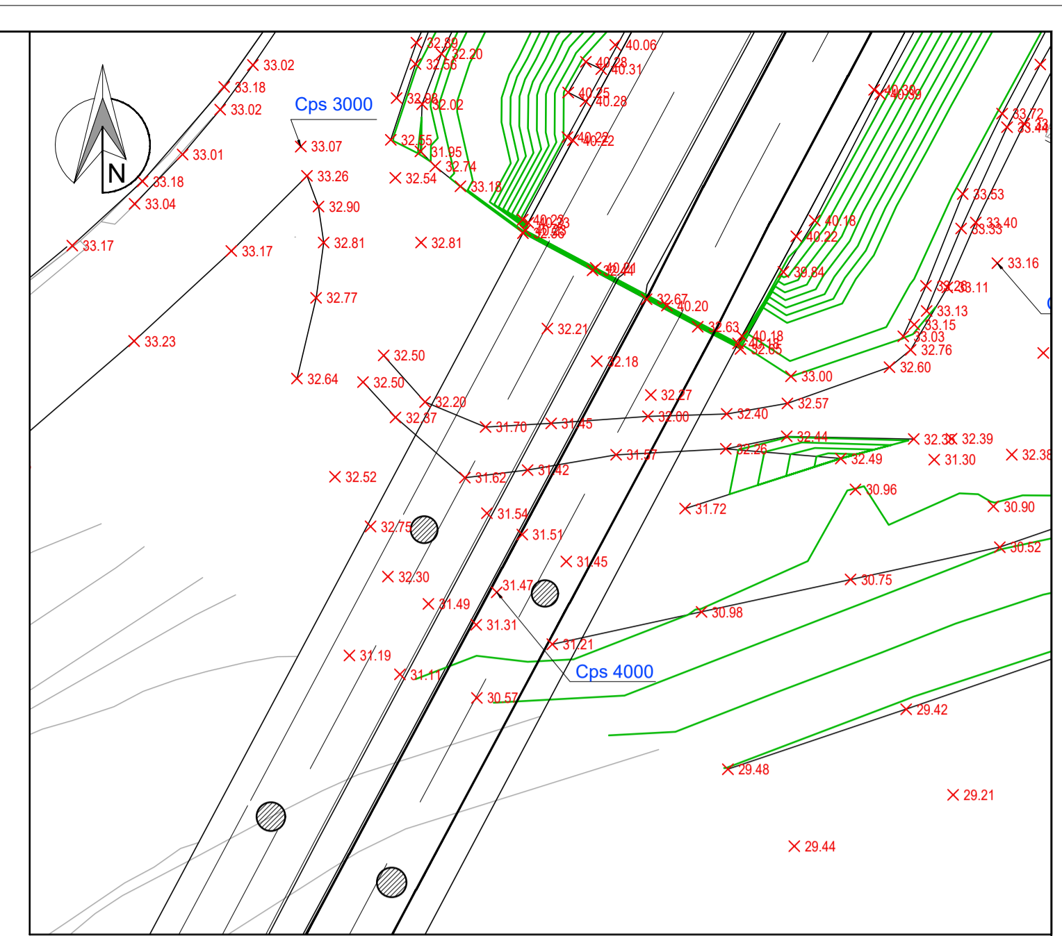
PLANIMETRIA DI RILIEVO - Inquadramento estremità Sud SCALA 1:500
