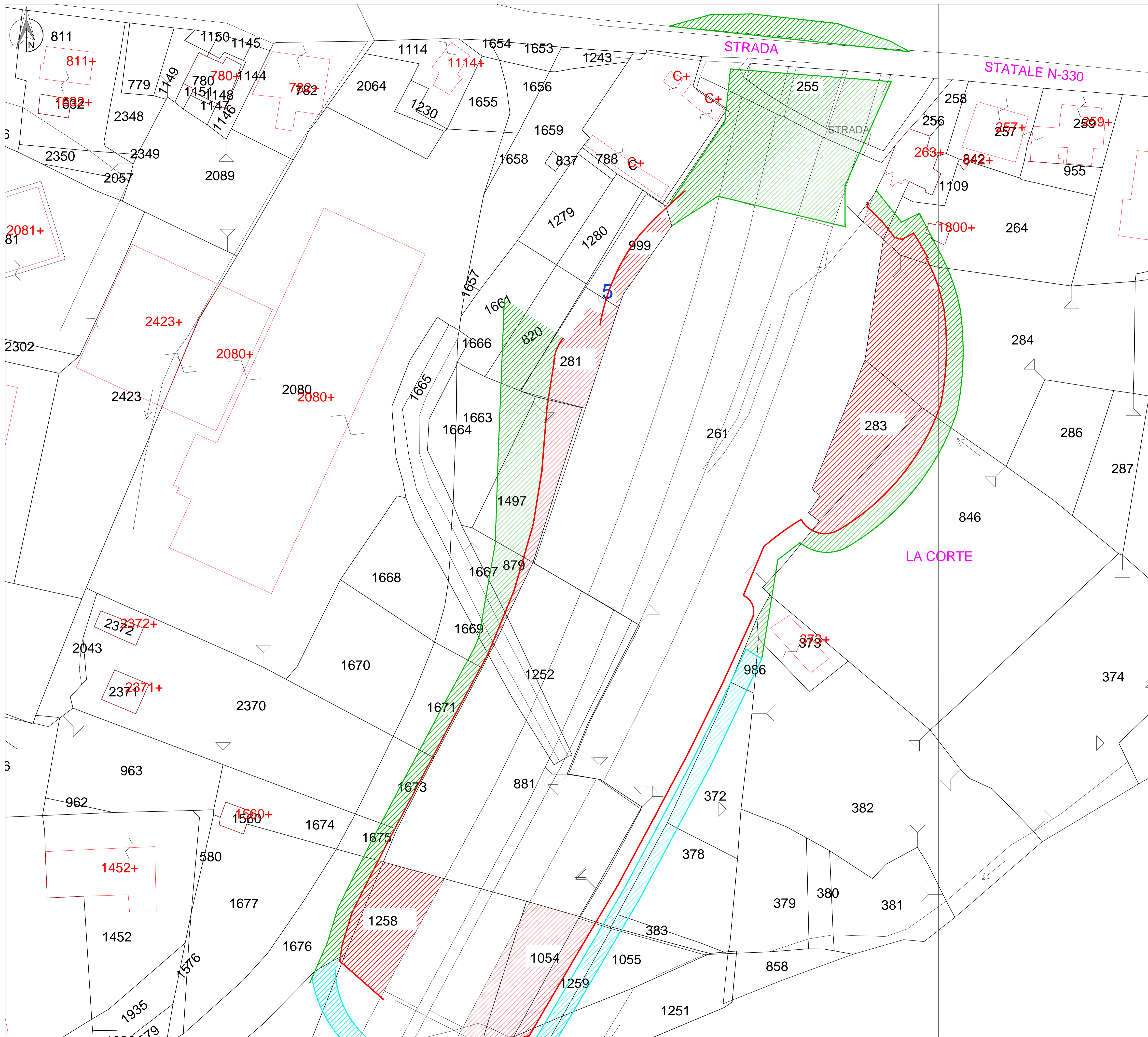
PIANO PARTICELLARE DI ESPROPRIO SCALA 1:500
