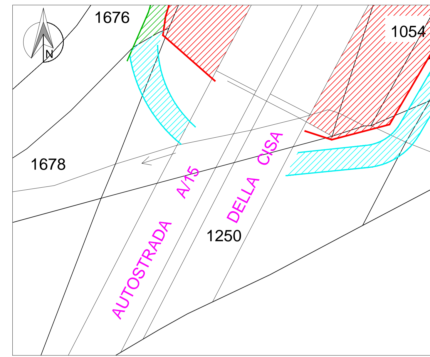
PIANO PARTICELLARE DI ESPROPRIO - Inquadramento estremità Sud SCALA 1:500
