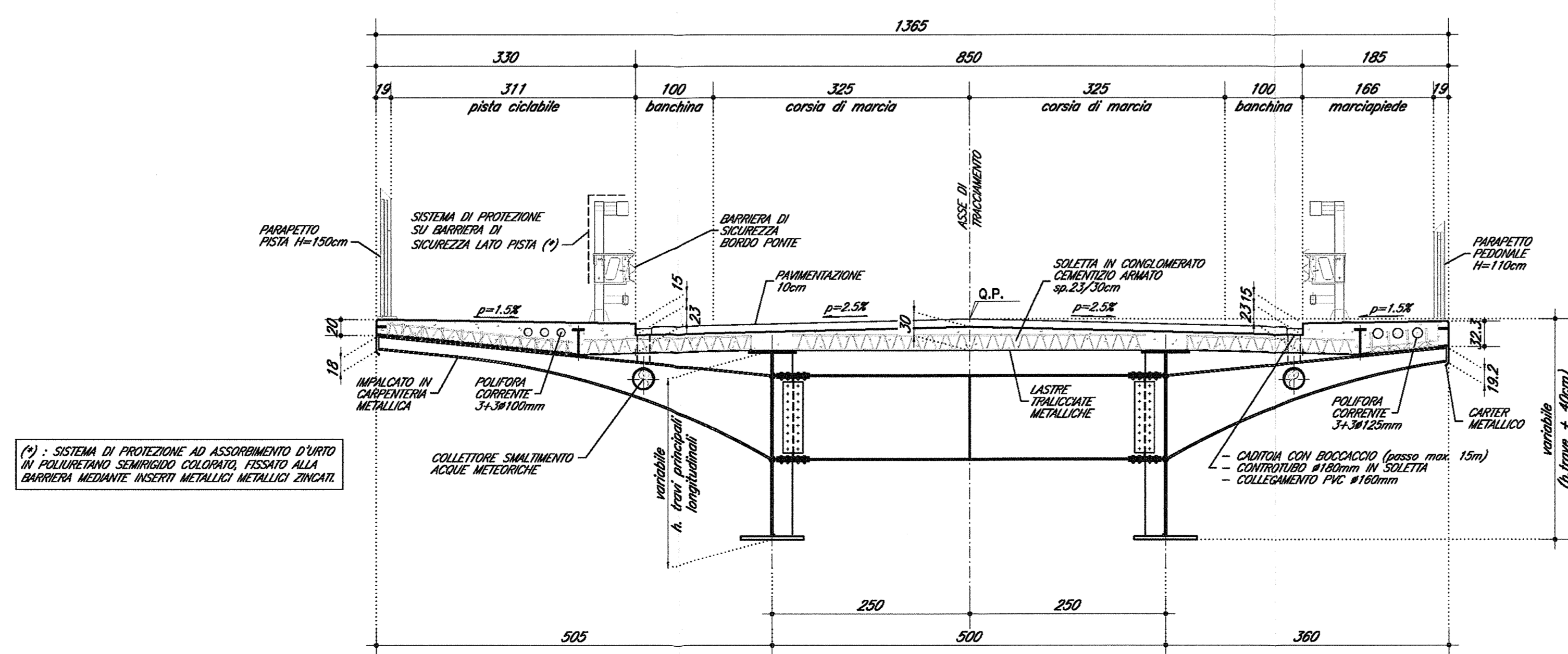
SEZIONE TRASVERSALE TIPO IMPALCATO 1:50 (Cat. F2 + pista ciclopedonale)
