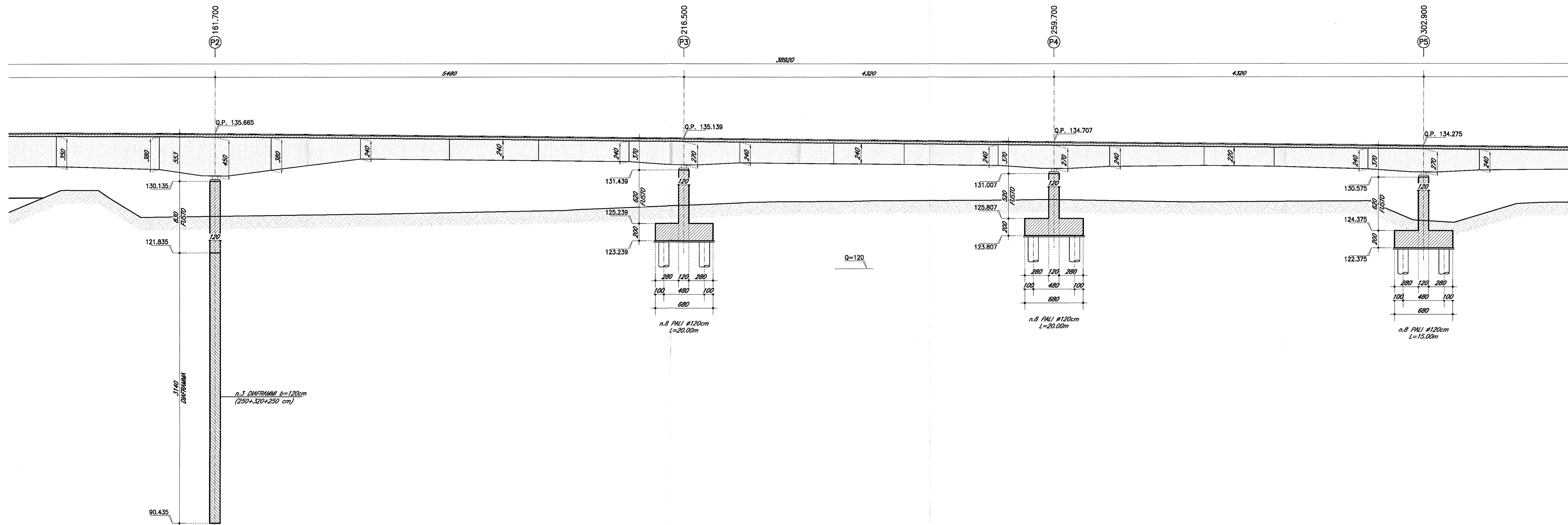
PROSPETTO LONGITUDINALE (2/3) 1:200
