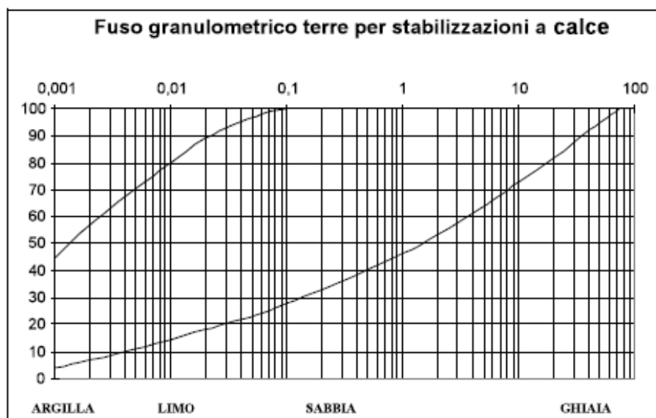
Figura 1 - Fuso granulometrico di riferimento (CNR-UNI 10006:2002).
