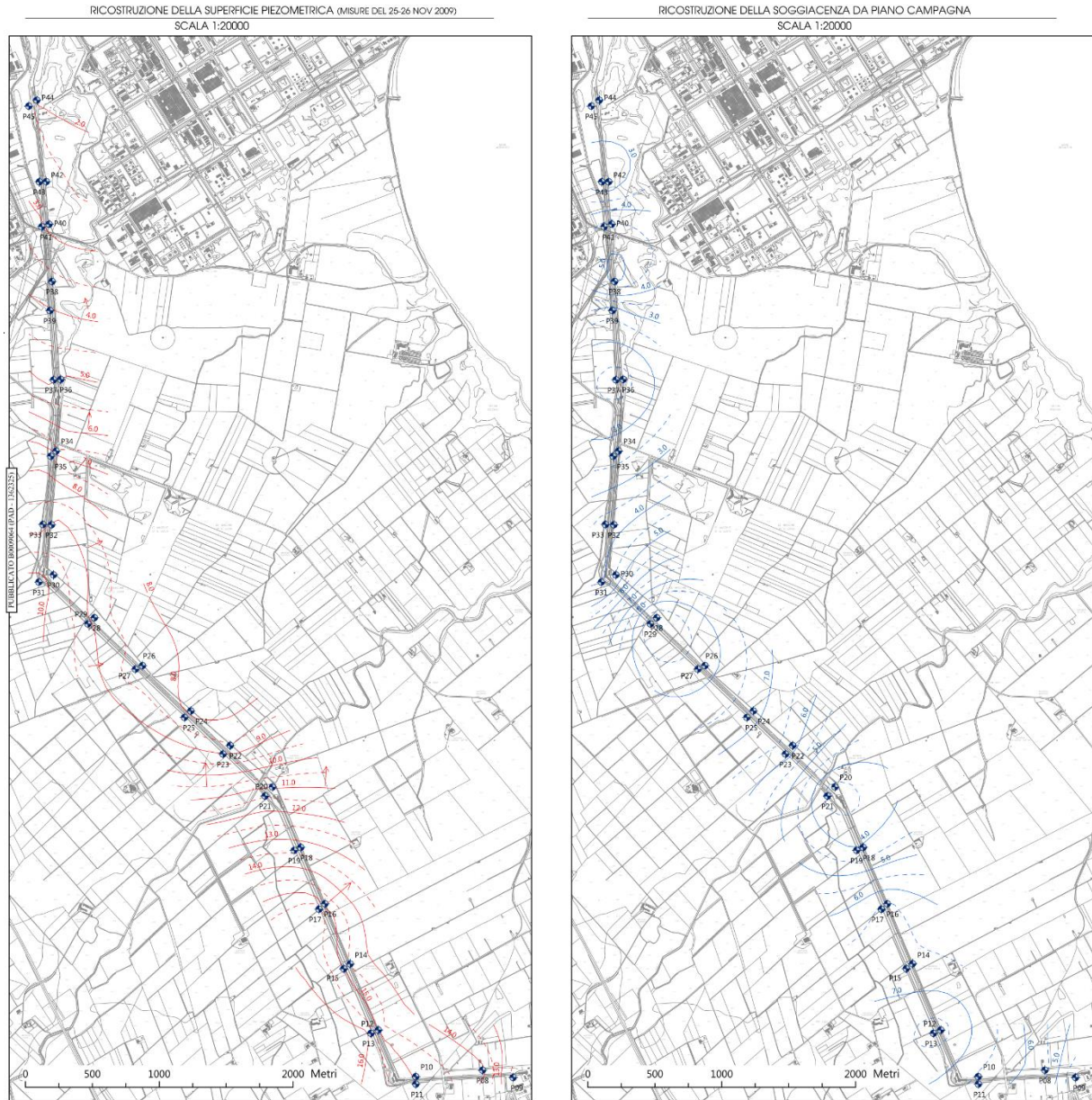
Figura 2 – Ricostruzione della superficie piezometrica della falda superficiale e della soggiacenza (m da p.c.) lungo l’Asse Attrezzato Policombustibile.
