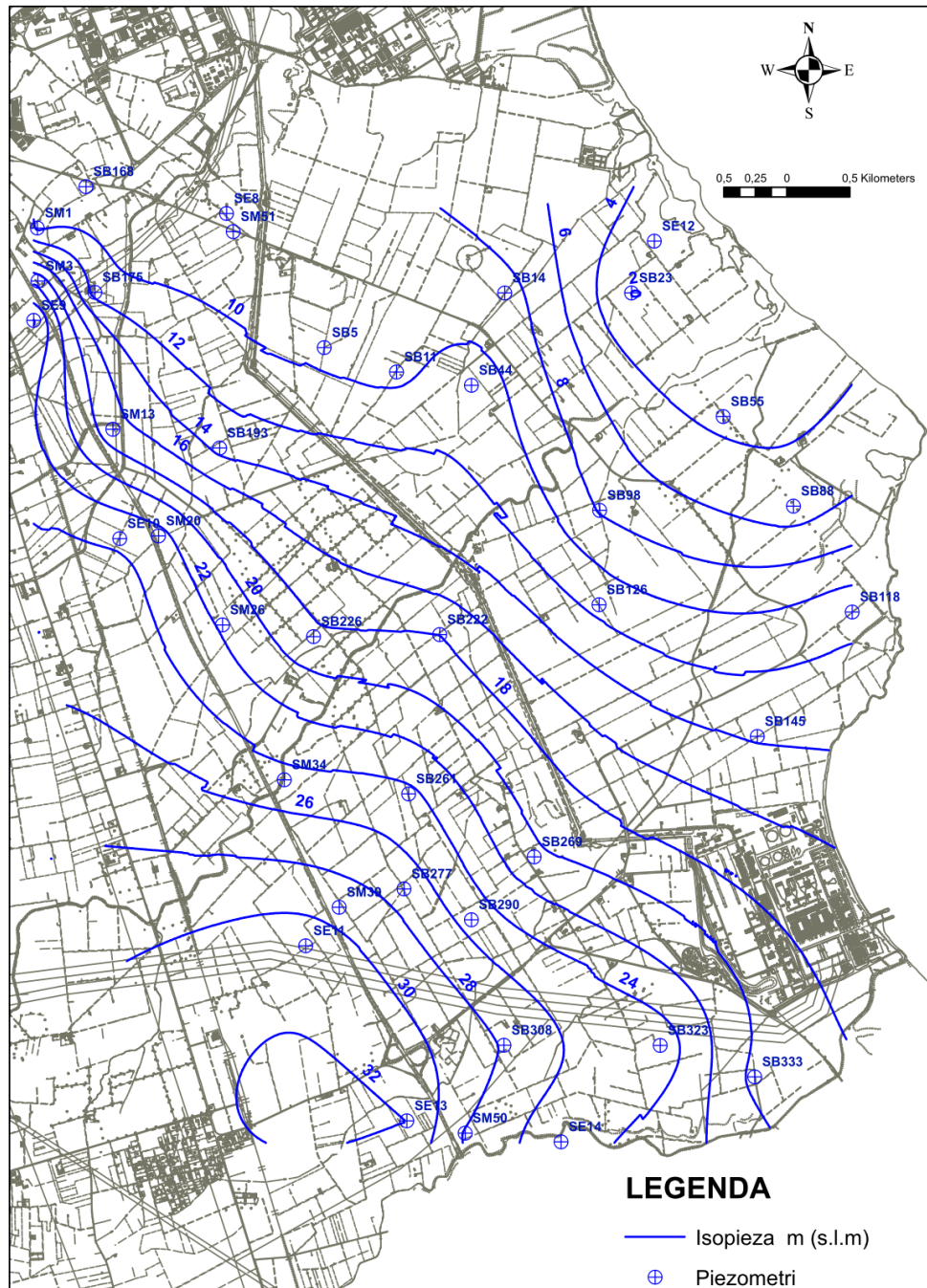
Figura 3 – Ricostruzione della superficie piezometrica della falda superficiale dell’area d’intervento.
