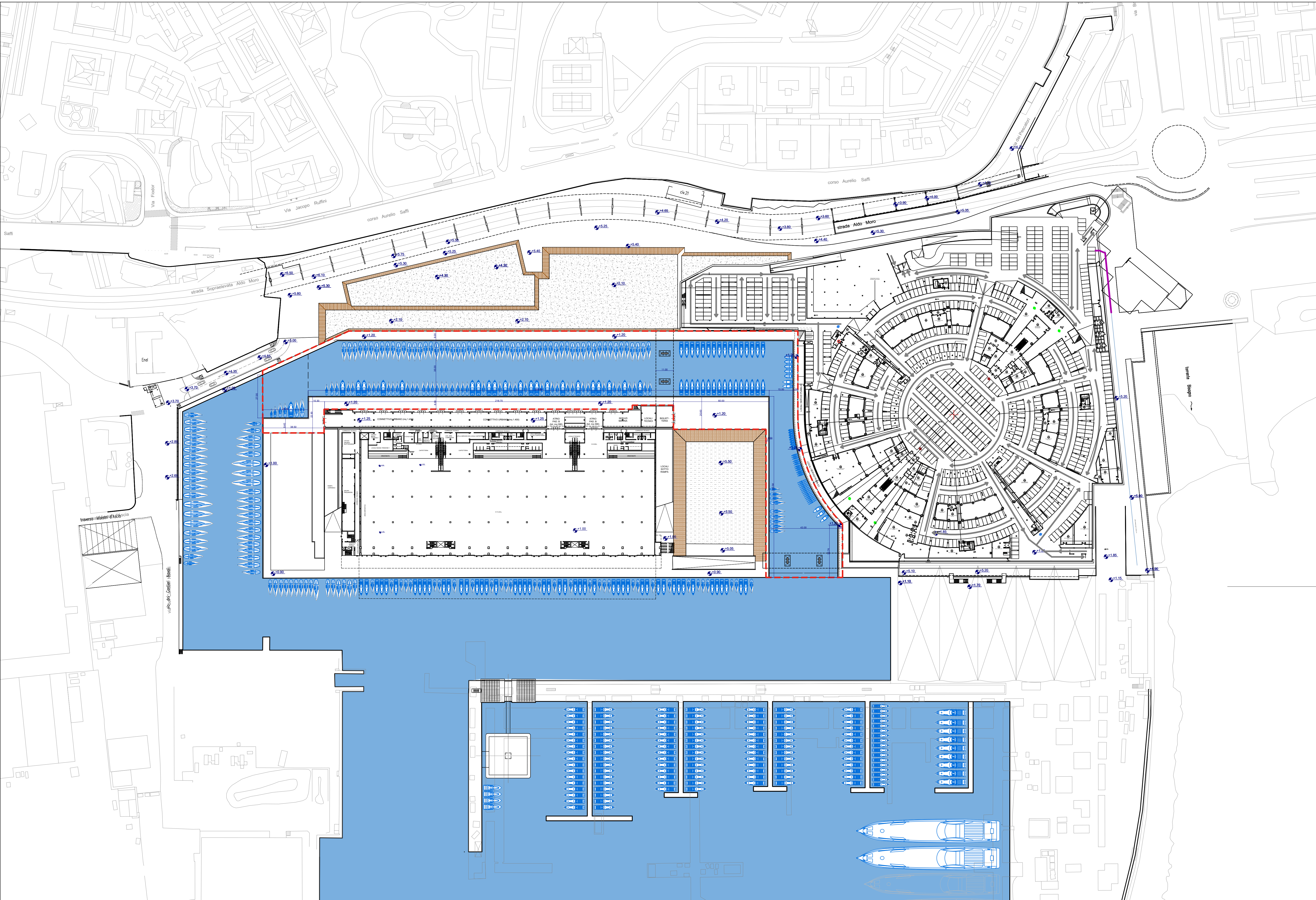
PLANIMETRIA DI PROGETTO - FASE 2-3 - scala 1:1.000
