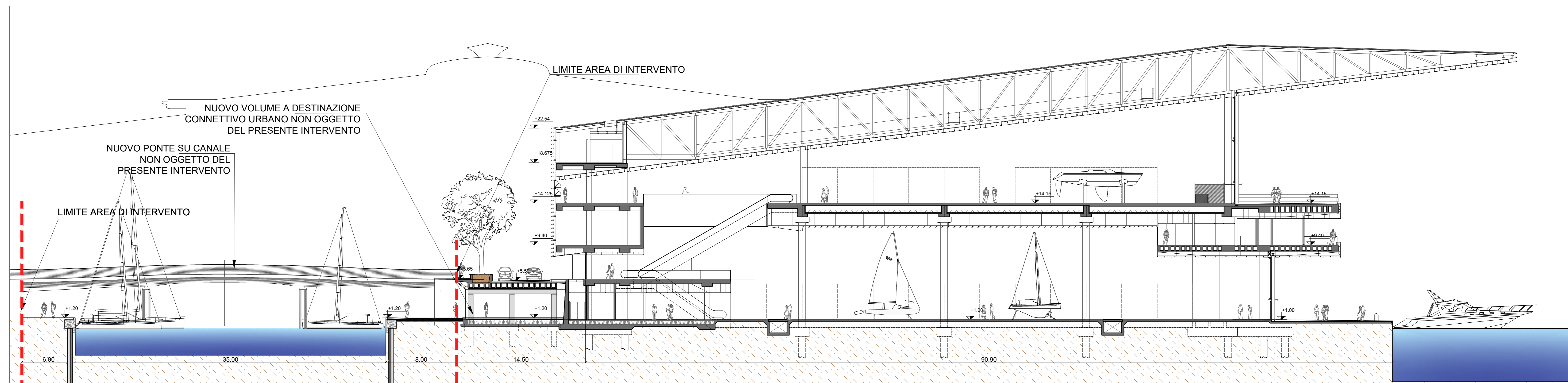
SEZIONE TRASVERSALE (E-E) scala 1:200
