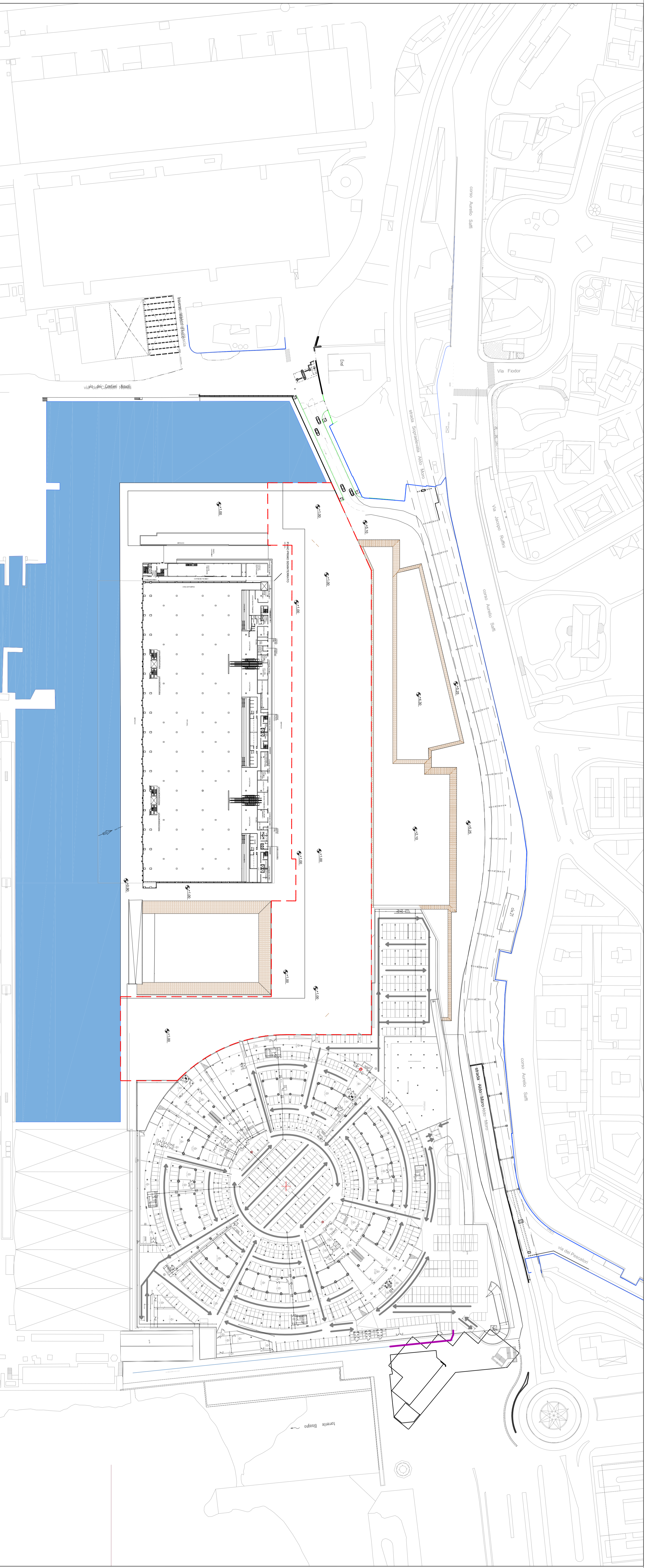
PLANIMETRIA GENERALE REALIZZAZIONE CANALI - ANTE OPERAM- Scala 1:1000
