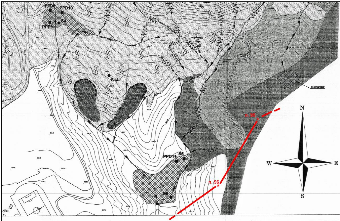
Figura 3.4.3/5 – Estratto della Carta Geologica e Geomorfologica – Tav. 3” allegata al “Progetto della sistemazione idrogeologica ed idraulica del lato meridionale del sito (versante Balangero) – Progetto definitivo (ridis.).
