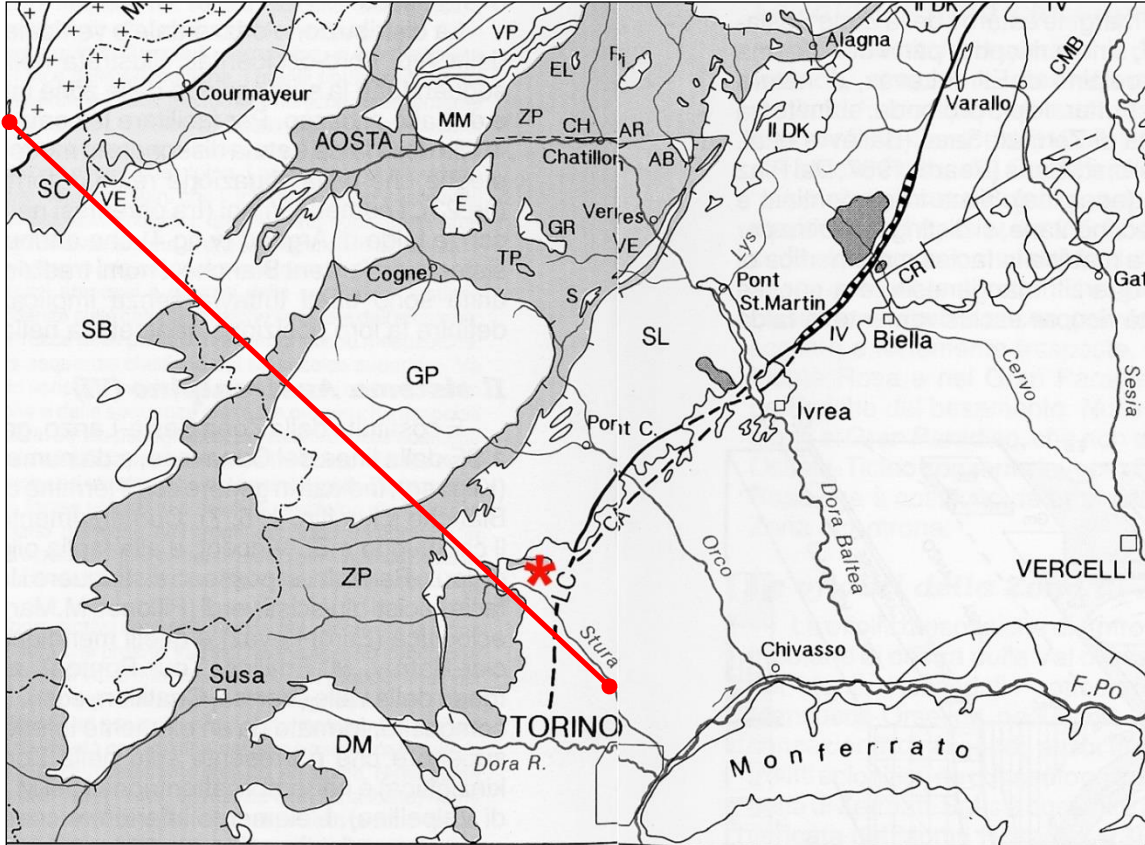
fig.21. Carta strutturale delle Alpi nord-occidentali. La catena a falde a vergenza europea (in media NW) comprende, dall'alto al basso e dall'interno all'esterno: a) Austroalpino: la Zona Sesia-Lanzo (SL), interna, comprendente i klippen della II Zona diorito-kinzigitica (IIDK); i lembi Austroalpini settentrionali di Verres (VE), Pillonet (Pi), Etinol-Levaz (EL), M.Mary (MM) e Dent Blanche (DB), comprendente il klippe della Valpelline (VP), e quelli meridionali del Santanel (S), Chatillon (CH), Glacier-Rafray (GR), Tour Ponton (TP) e M.Emilius (E); Scisti di Fobello - Rimella (FR); b) unità ofiolitiche della Zona Piemontese (ZP), indifferenziate; c) falde Pennidiche superiori del Monte Rosa (MR), Arcesa-Brusson (AB), Gran Paradiso (GP) e Dora-Maira (DM); d) unità ofiolitica di Antrona (An); e) sistema medio-pennidico del Gran San Bernardo (SB), indifferenziato, ed unità "radicali" di Camughera-Moncuoco (CM) e Berisal (B); e) unità Pennidiche inferiori nella finestra dell'Ossola: falde di basamento del Monte Leone (ML), Lebedun (LB), Antigorio (A) e Verampio (V); in Ticino: Adula (AD), Margna (MA), Simano (SI) e Lucomagno-Leventina (Lu-Le), separate da coperture mesozoiche e dalle unità ofiolitiche della Zona Vallesana (VA), indistinte; f) Unità Pennidiche esterne della Valle d'Aosta: unità ofiolitica del Versoyen (VE) e falde di scollamento della Zona Sion-Courmayeur (SC), sostituite a S di Mutiers dalle unità Subbrianzonesi (SBR); il piano di sovrascorrimento che delimita alla base e alla fronte la Zona Pennidica è detto fronte Pennidico (FP); g) Zone esterne: unità di basamento (crocette; PE: Pelvoux) e falde Delfinesi, Elvetiche ed Ultraelvetiche, indifferenziate, ricoperte dalla pila di falde Pennidiche di scollamento delle Prealpi Romande e del Chiabiese; h) Molassa esterna (MO). Lungo il lineamento Periadriatico (linea del Canavese: LC) è situata la Zona del Canavese (CA). Segue, al suo interno, il sistema S-vergente delle Alpi Meridionali che è formato, da NW a SE e dal basso all'alto, dalla Zona Ivrea-Verbano (IV) e dalla Serie dei Laghi (LA). Linee tettoniche: Tonale (TO), Sempione (LS), Centovalli (LC), Aosta-Ranzola (AR), Cremosina (CR), Cossagno-Mergozzo-Brissago (CMB). Sono messe in evidenza le unità Piemontesi (1) e Vallesane (2) ed i corpi plutonici (3a) e vulcanici (3b) Periadriatici di età oligocenica.
