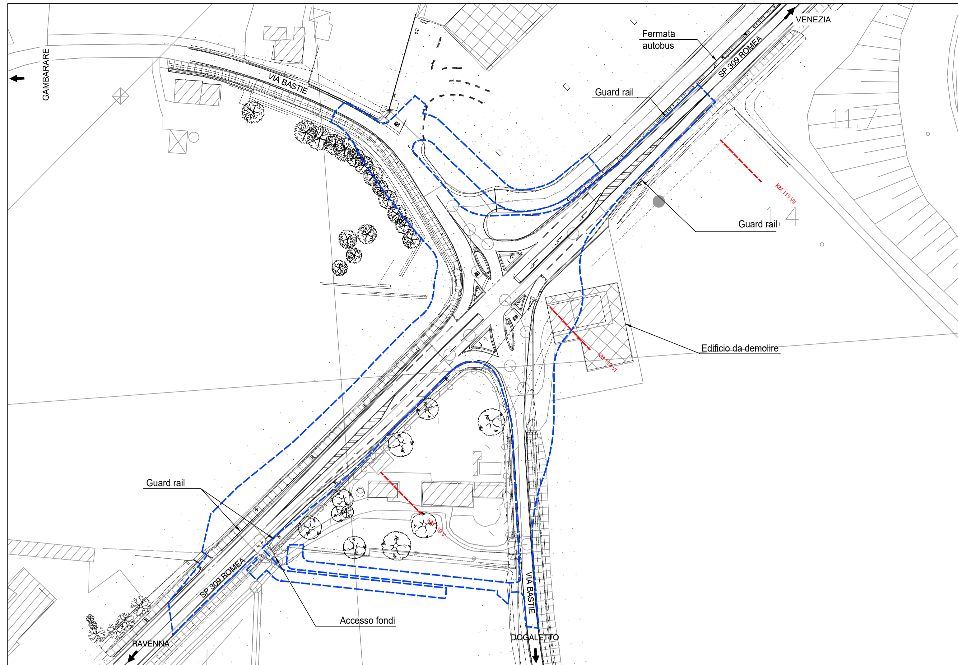
PLANIMETRIA STATO DI FATTO - RILIEVO Scala 1:1000
