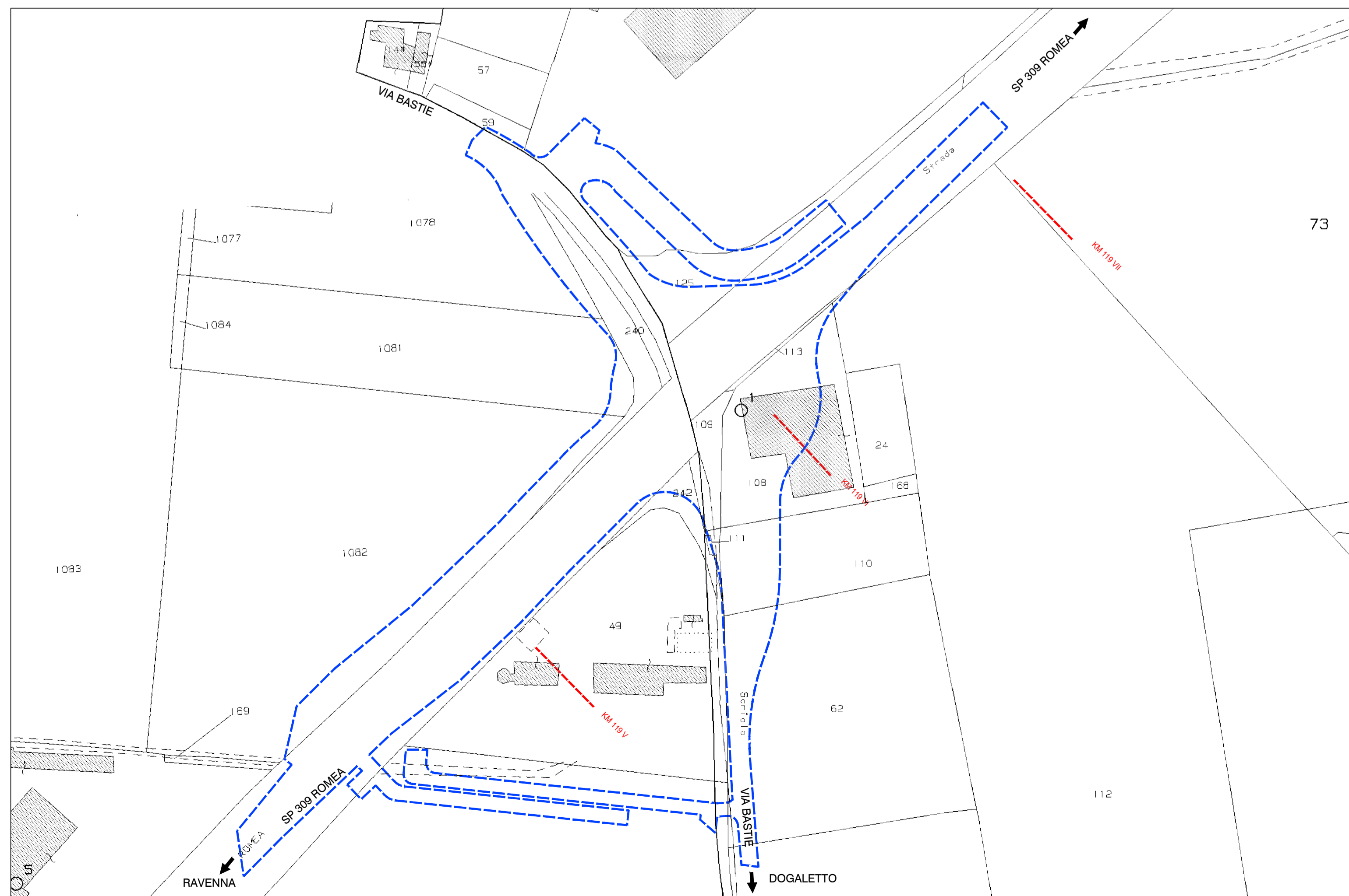
PLANIMETRIA CATASTALE Scala 1:1000
